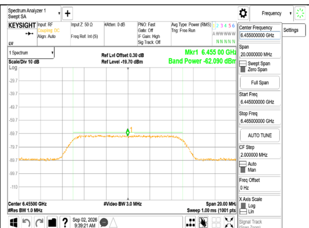
802.11be 20MHz 6455MHz AWGN:6455MHz
