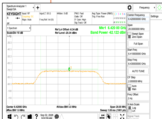
802.11be 320MHz 6265MHz AWGN:6420
