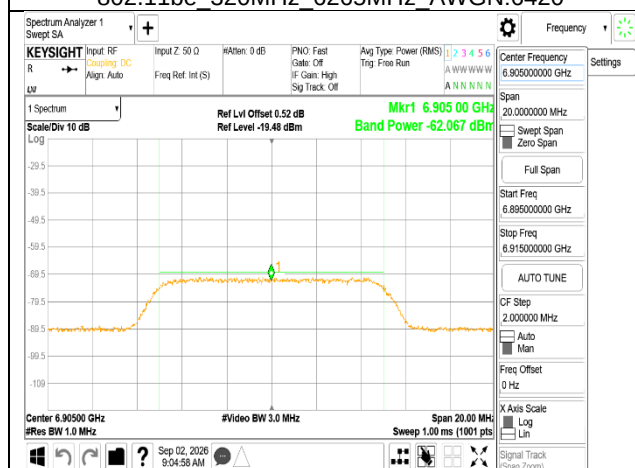
802.11be 320MHz 6905MHz AWGN:6905MHz
