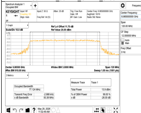
802.11ax_80MHz_Chain1_6865MHz
