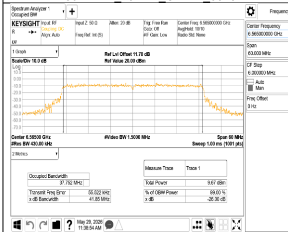
802.11be 40MHz Chain1 6565MHz
