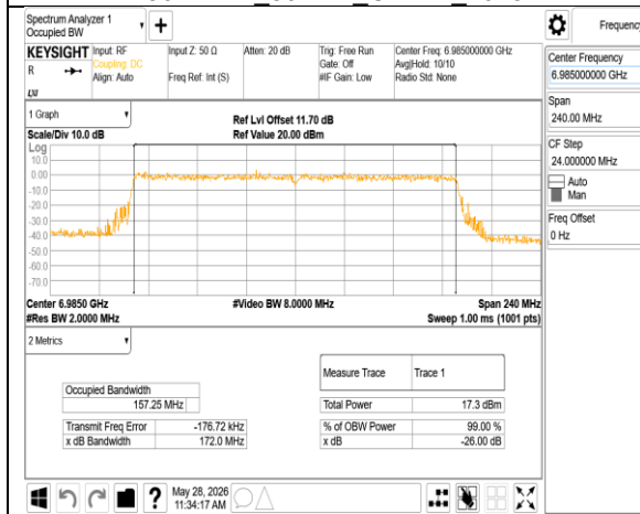
802.11ax 160MHz Chain0 6985MHz
