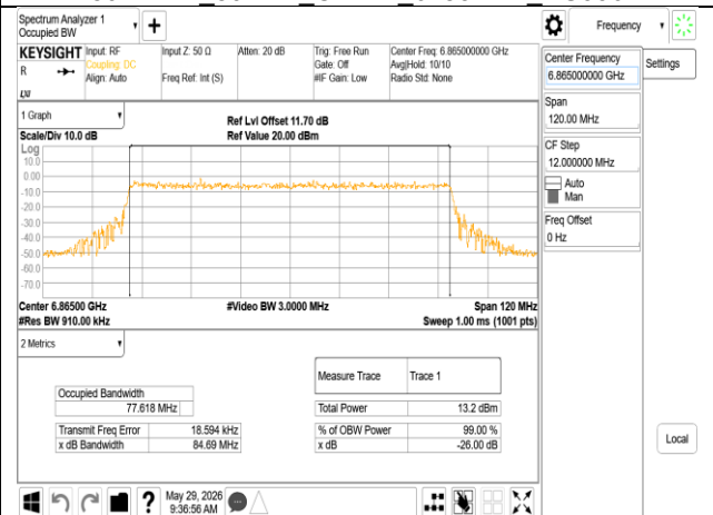
802.11ax_80MHz_Chain1_6865MHz RU996
