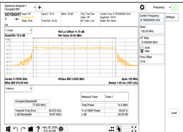
802.11ax_80MHz_Chain1_6785MHz RU996
