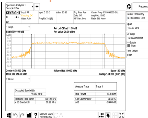
802.11ax_80MHz_Chain1_6785MHz
