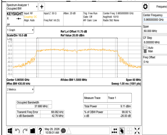
802.11be 40MHz Chain1 5965MHz
