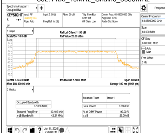
802.11be 40MHz Chain0_6845MHz
