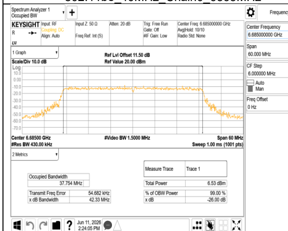
802.11be 40MHz Chain0_6685MHz
