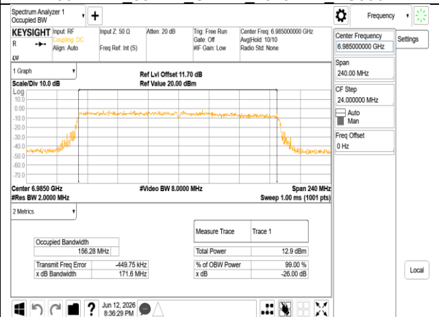
802.11ax 160MHz Chain0 6985MHz RU996x2
