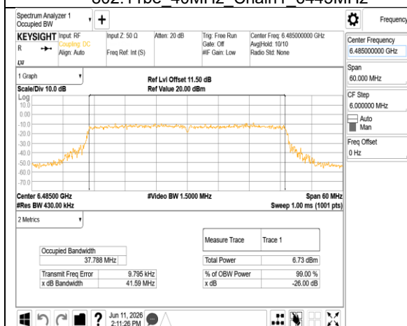
802.11be 40MHz Chain1 6485MHz
