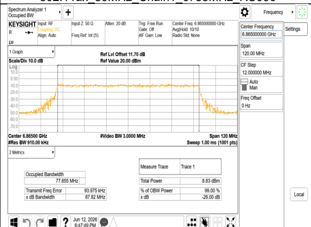
802.11ax 80MHz Chain1 6865MHz RU996
