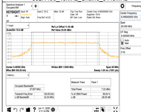
802.11be_40MHz_Chain0_6485MHz
