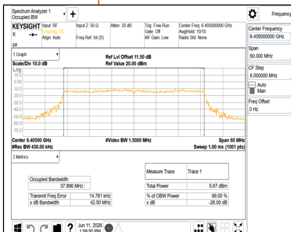
802.11be 40MHz Chain1 6405MHz
