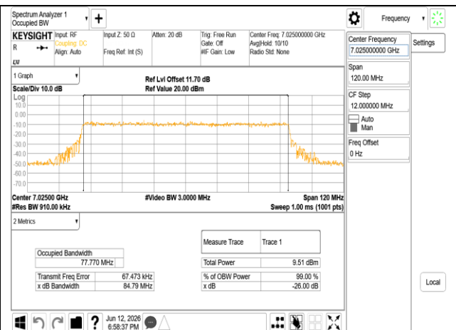
802.11ax 80MHz Chain1 7025MHz RU996
