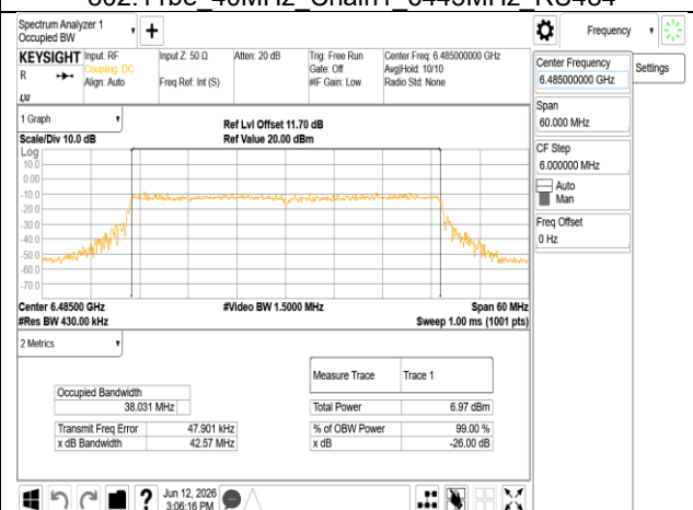
802.11be 40MHz Chain1 6485MHz RU484
