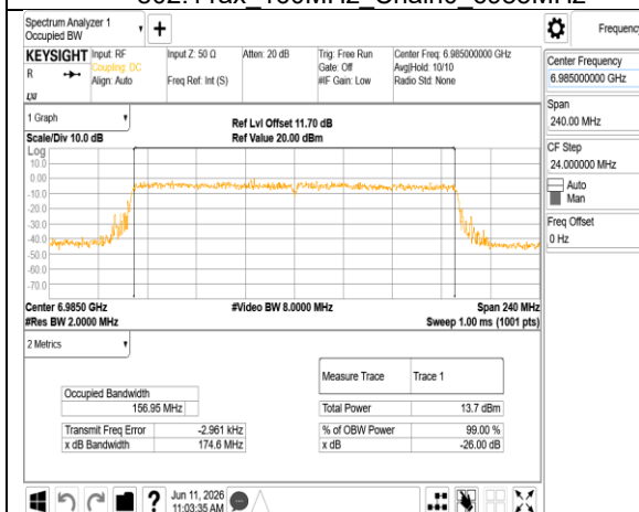
802.11ax 160MHz Chain1 6985MHz
