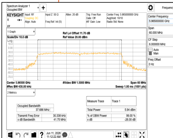
802.11be 40MHz Chain0 5965MHz
