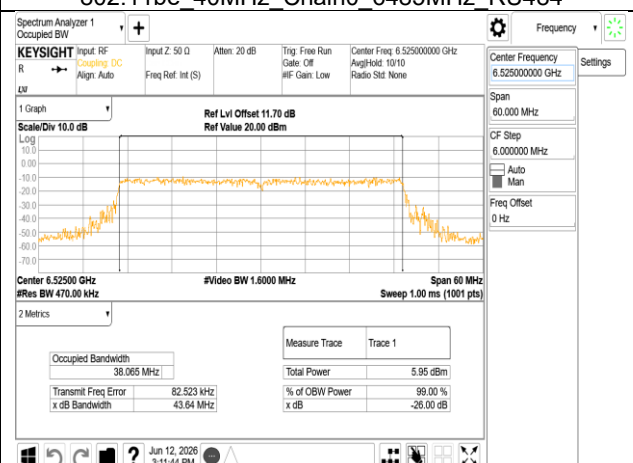
802.11be_40MHz_Chain0_6525MHz RU484
