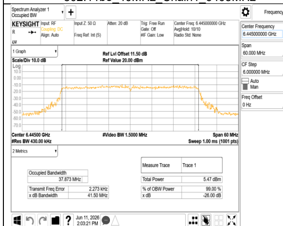
802.11be 40MHz Chain1 6445MHz
