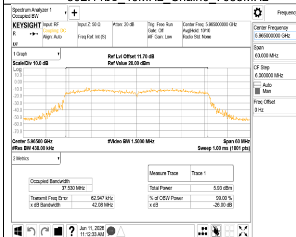
802.11be 40MHz Chain1 5965MHz
