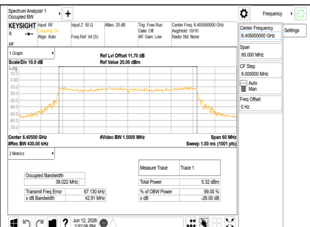
802.11be 40MHz Chain1 6405MHz RU484
