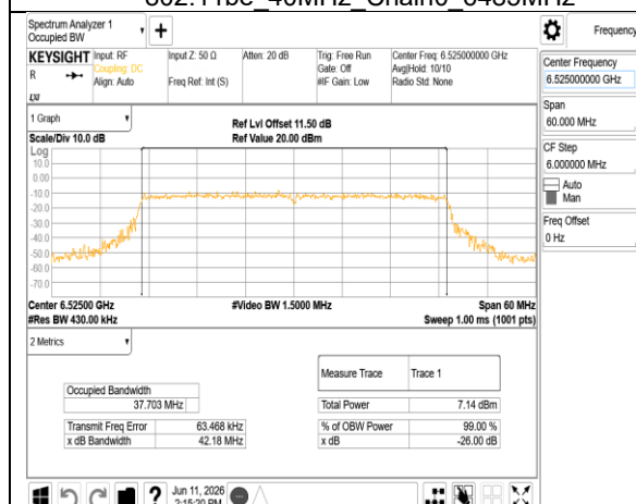
802.11be_40MHz_Chain0_6525MHz
