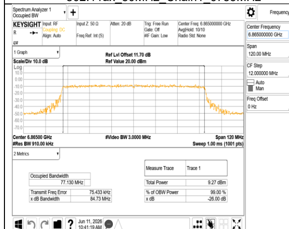
802.11ax 80MHz Chain1 6865MHz
