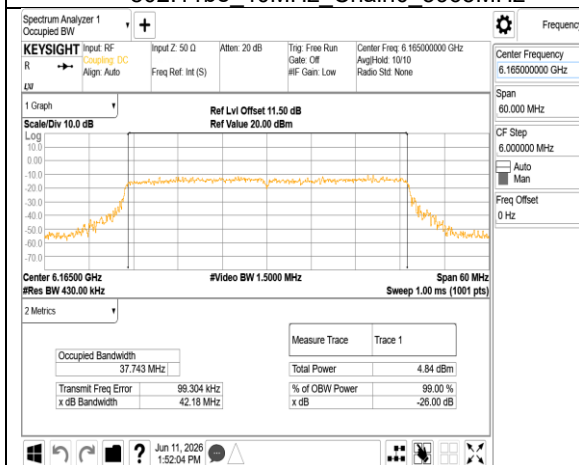
802.11be 40MHz Chain0 6165MHz
