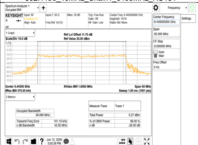
802.11be 40MHz Chain1 6445MHz RU484
