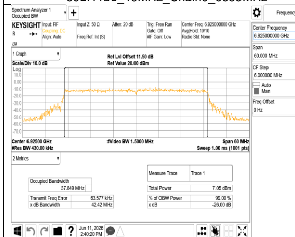
802.11be 40MHz Chain0 6925MHz
