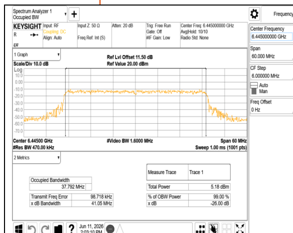
802.11be_40MHz_Chain0_6445MHz
