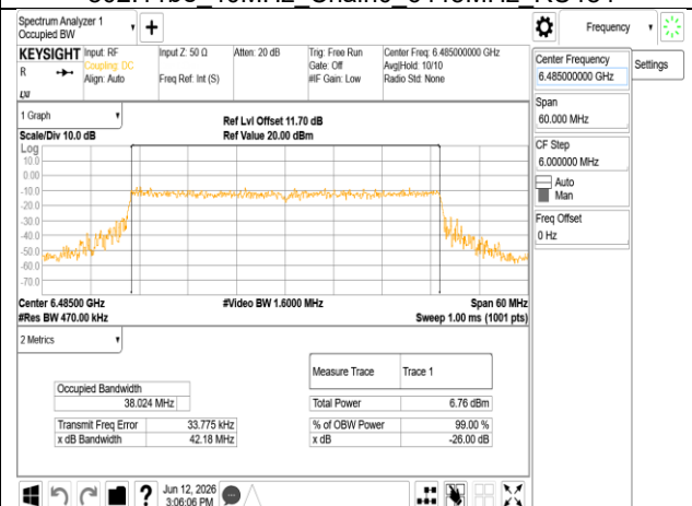
802.11be_40MHz_Chain0_6485MHz RU484
