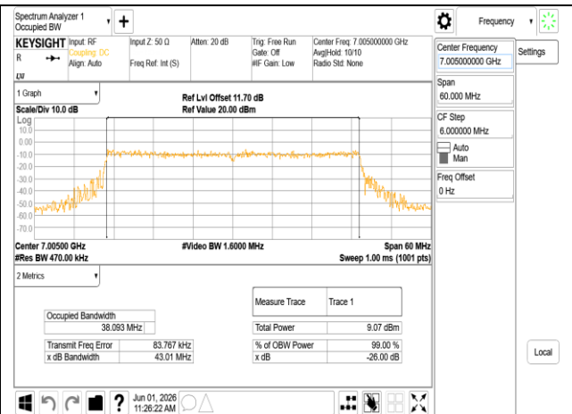
802.11be 40MHz Chain1 7005MHz RU484
