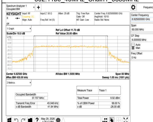
802.11be 40MHz Chain1 6925MHz
