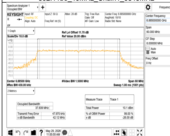
802.11be 40MHz Chain1 6885MHz
