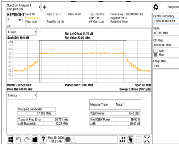
802.11be 40MHz Chain1 7085MHz
