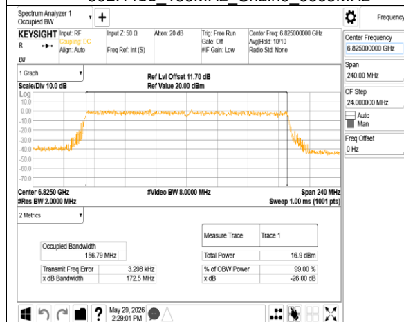
802.11be 160MHz Chain0 6825MHz
