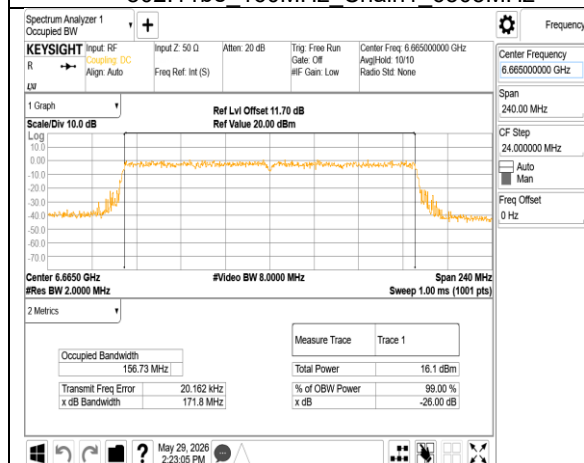
802.11be 160MHz Chain1 6665MHz
