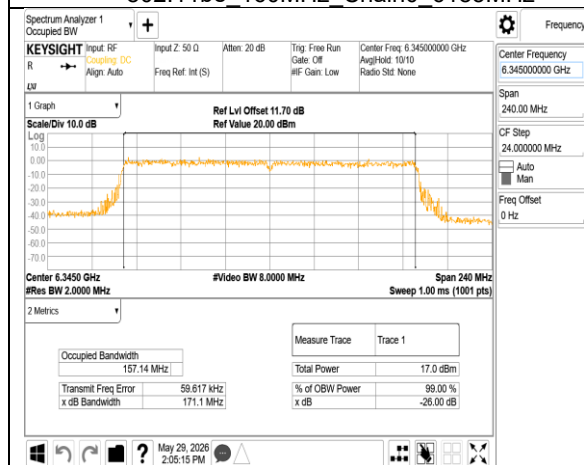
802.11be 160MHz Chain0 6345MHz
