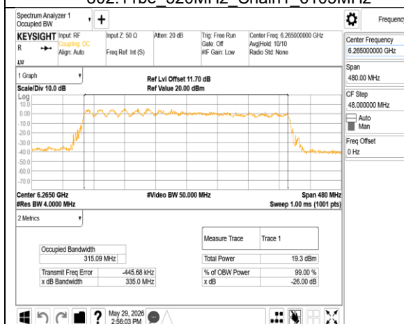
802.11be 320MHz Chain1 6265MHz
