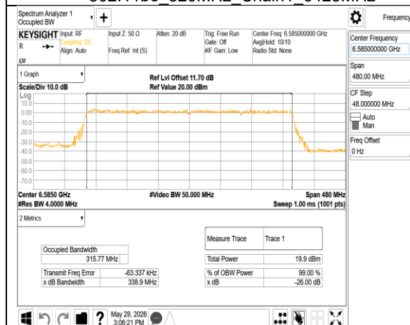
802.11be 320MHz Chain1 6585MHz
