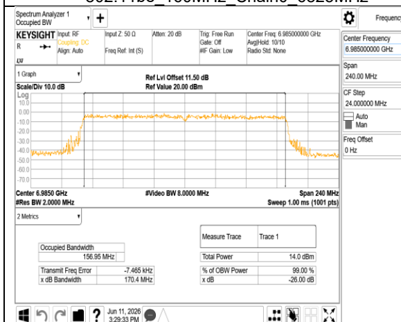
802.11be 160MHz Chain0 6985MHz
