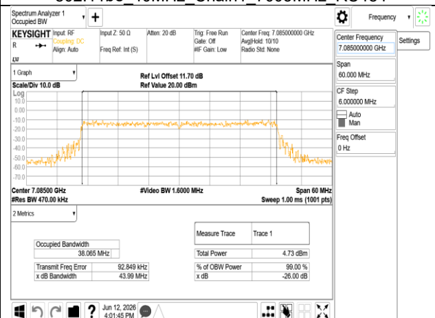
802.11be 40MHz Chain1 7085MHz RU484
