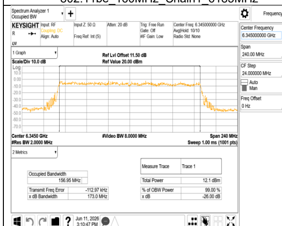
802.11be 160MHz Chain1 6345MHz
