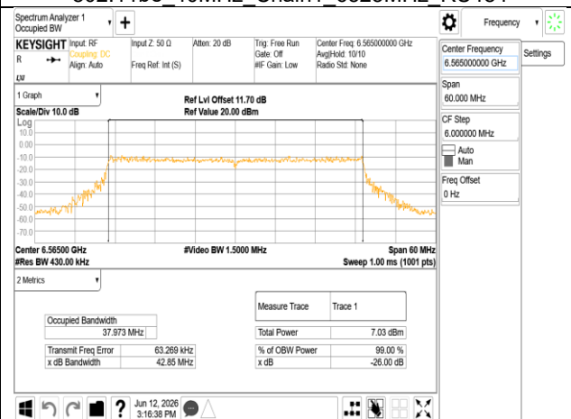
802.11be 40MHz Chain1 6565MHz RU484
