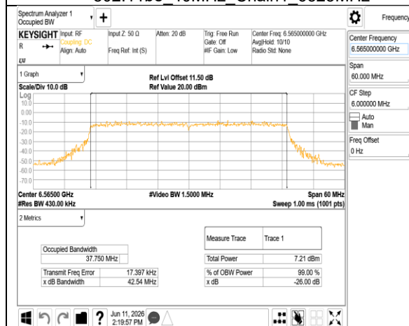
802.11be 40MHz Chain1 6565MHz
