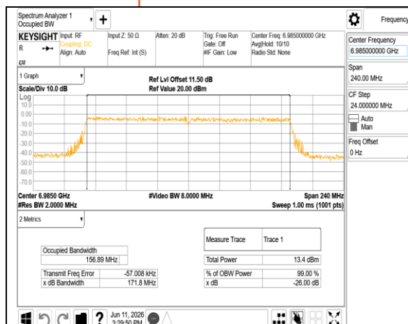
802.11be 160MHz Chain1 6985MHz
