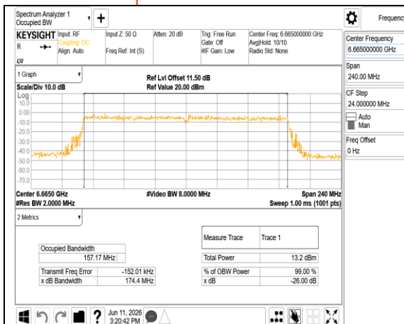
802.11be 160MHz Chain0 6665MHz
