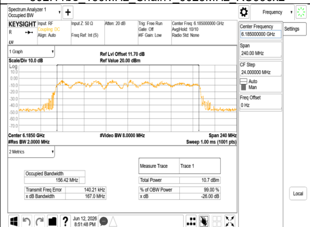
802.11be 160MHz Chain1 6185MHz RU996x2
