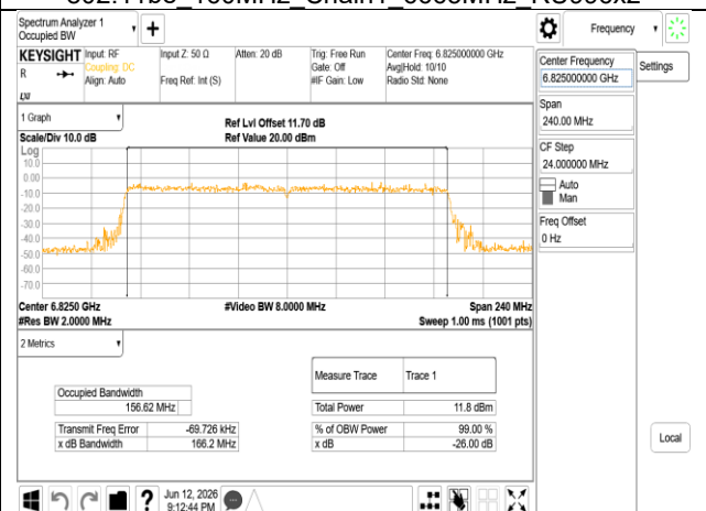
802.11be 160MHz Chain1 6825MHz RU996x2
