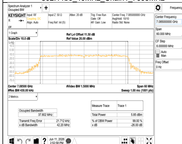
802.11be 40MHz Chain1 7085MHz
