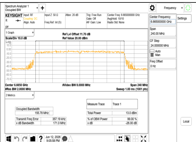
802.11be 160MHz Chain0 6665MHz RU996x2
