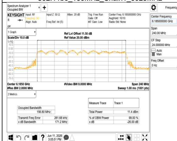
802.11be 160MHz Chain1 6185MHz
