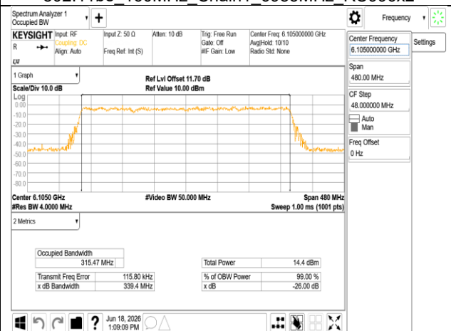
802.11be 320MHz Chain0 6105MHz RU996x4
