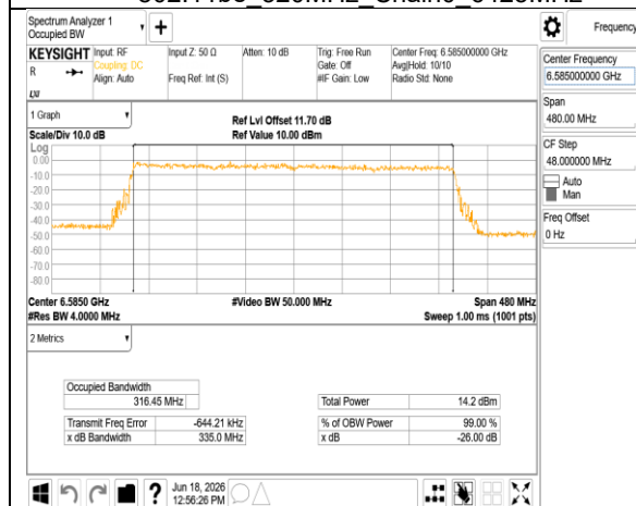
802.11be 320MHz Chain0 6585MHz
