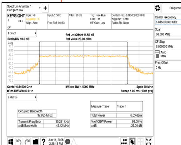
802.11be 40MHz Chain1 6845MHz
