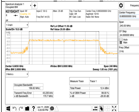
802.11be 160MHz Chain1 6665MHz
