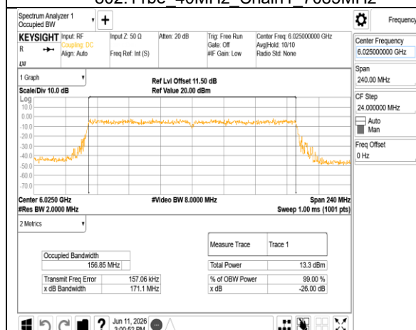
802.11be 160MHz Chain0 6025MHz
