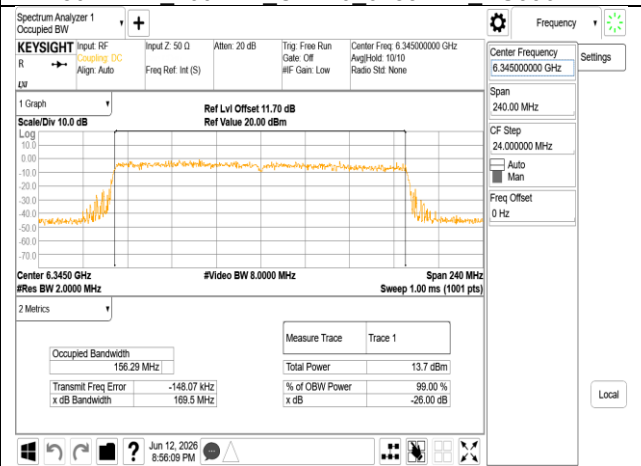
802.11be 160MHz Chain0 6345MHz RU996x2
