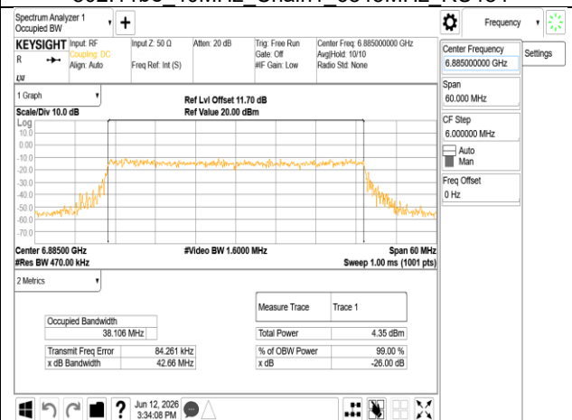
802.11be 40MHz Chain1 6885MHz RU484
