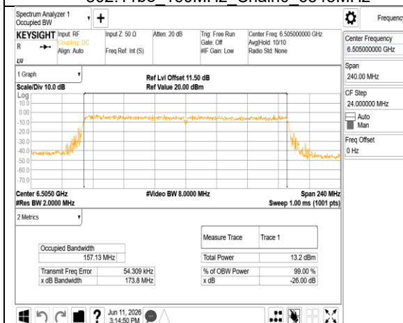
802.11be 160MHz Chain0 6505MHz
