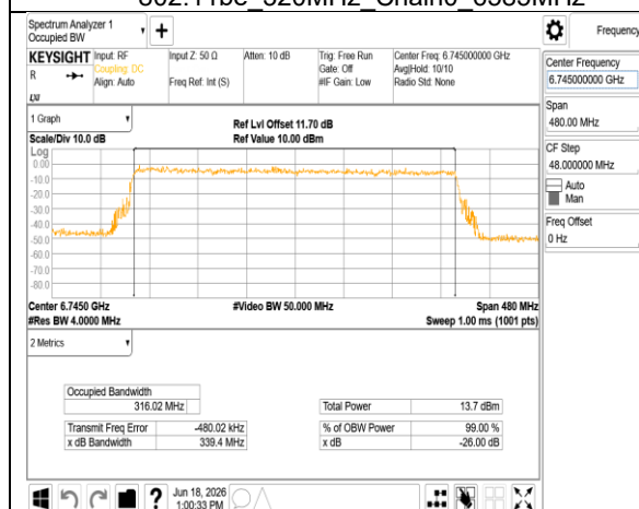
802.11be 320MHz Chain0 6745MHz
