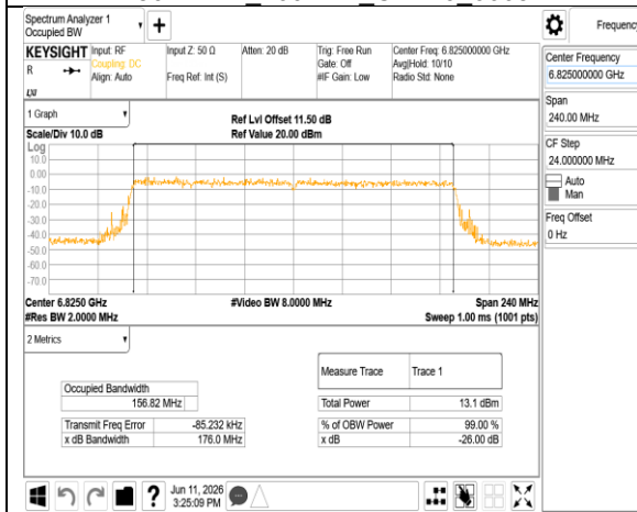
802.11be 160MHz Chain0 6825MHz
