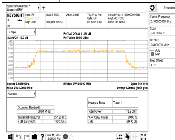
802.11be 160MHz Chain0 6185MHz
