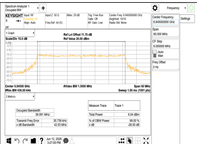
802.11be 40MHz Chain1 6845MHz RU484
