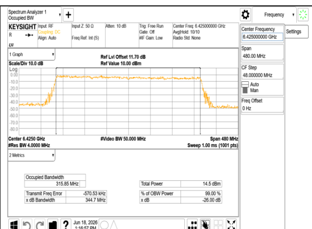
802.11be 320MHz Chain0 6425MHz RU996x4
