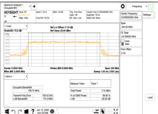
802.11be 160MHz Chain1 6505MHz RU996x2
