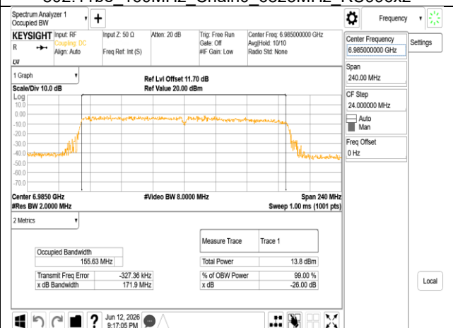
802.11be 160MHz Chain0 6985MHz RU996x2
