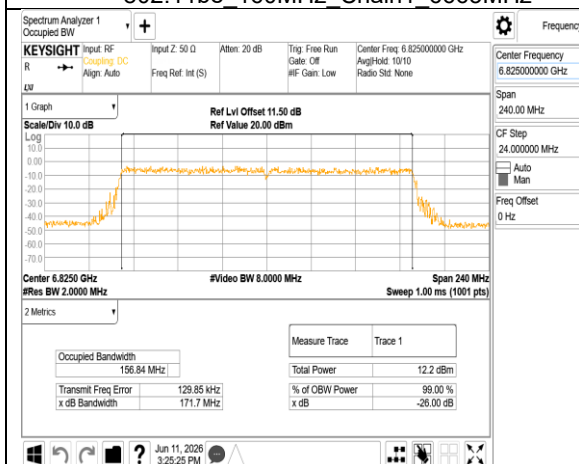
802.11be 160MHz Chain1 6825MHz
