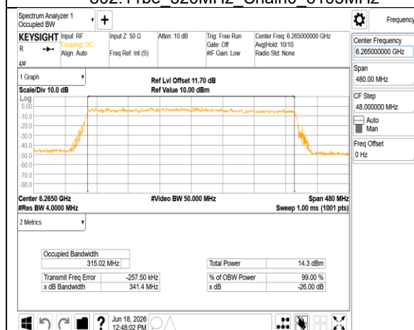
802.11be 320MHz Chain0 6265MHz
