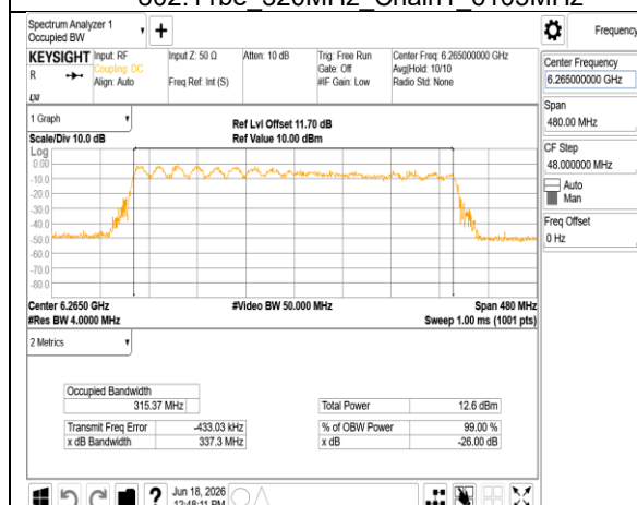
802.11be 320MHz Chain1 6265MHz
