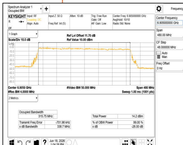
802.11be 320MHz Chain0 6905MHz
