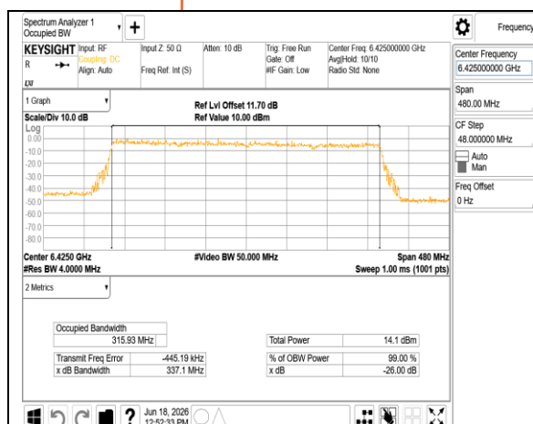
802.11be 320MHz Chain0 6425MHz
