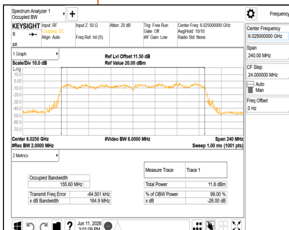
802.11be 160MHz Chain1 6025MHz
