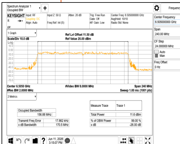
802.11be 160MHz Chain1 6505MHz
