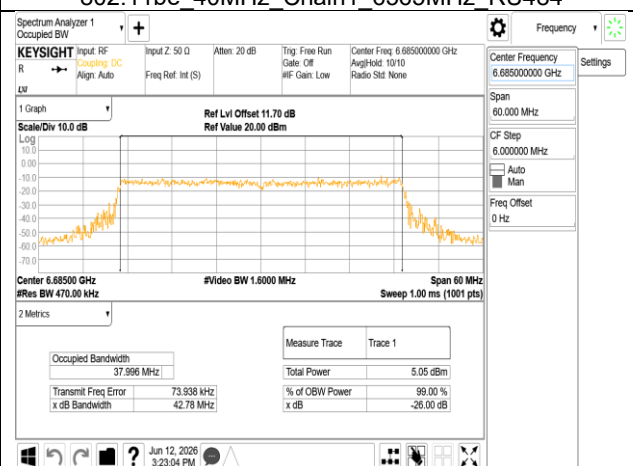
802.11be 40MHz Chain1 6685MHz RU484
