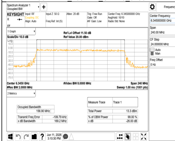
802.11be 160MHz Chain0 6345MHz
