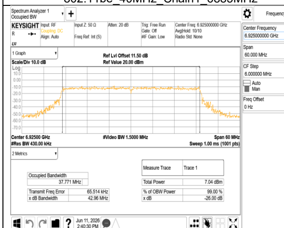
802.11be 40MHz Chain1 6925MHz
