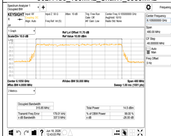
802.11be 320MHz Chain0 6105MHz
