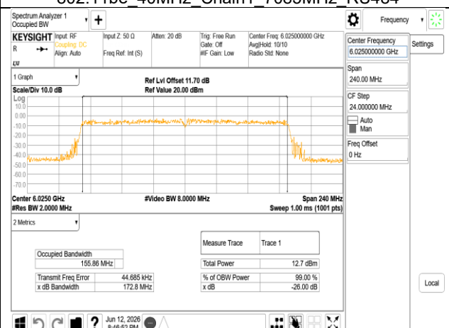
802.11be 160MHz Chain0 6025MHz RU996x2
