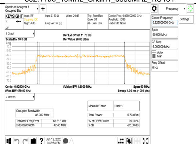
802.11be 40MHz Chain1 6925MHz RU484
