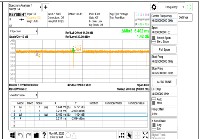
802.11ax 160MHz Chain0 6025MHz RU996x2
