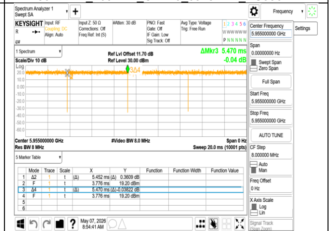
802.11be 20MHz Chain0 5955MHz
