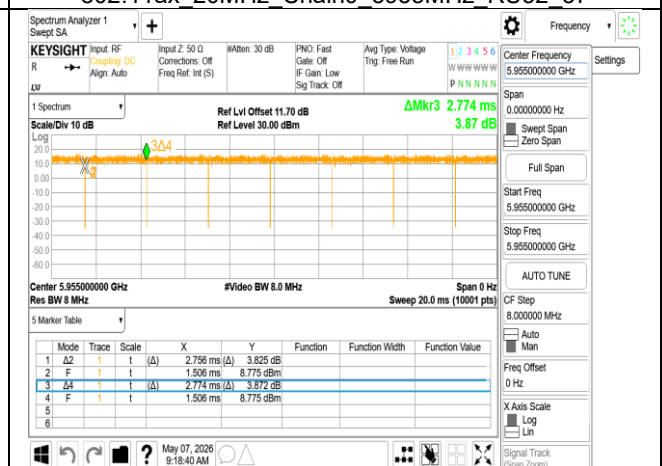
802.11ax 20MHz Chain0 5955MHz RU242
