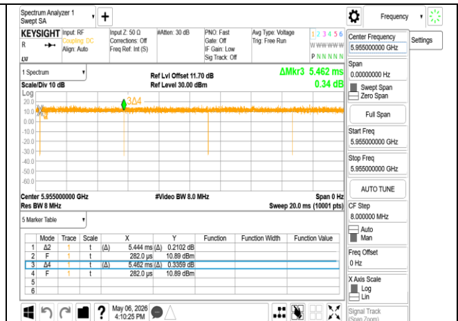
802.11ax 20MHz Chain0 5955MHz
