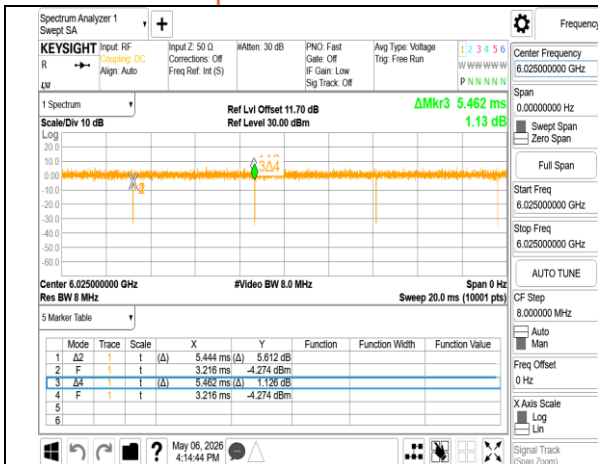
802.11ax 160MHz Chain0 6025MHz
