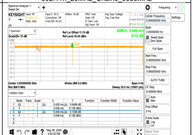
802.11ac_20MHz_Chain0_5955MHz
