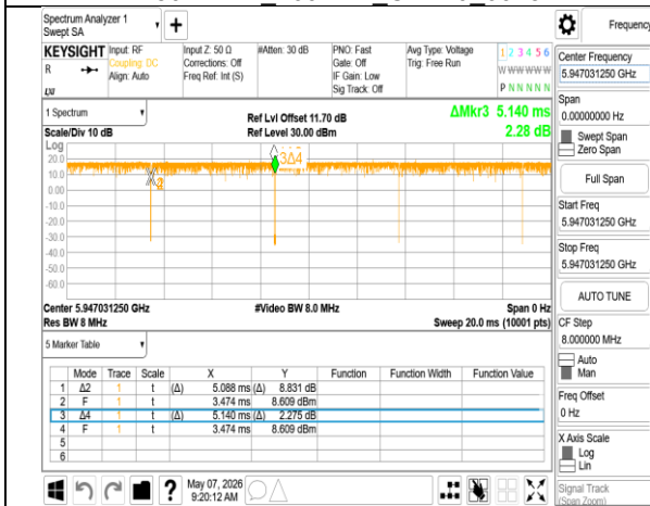
802.11ax 20MHz Chain0 5955MHz RU26 0
