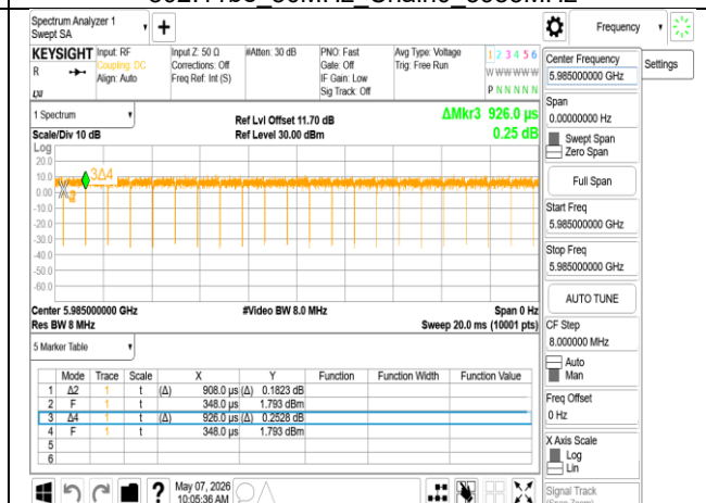
802.11be_80MHz_Chain0_5985MHz_RU996
