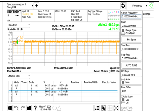
802.11be 320MHz Chain0 6105MHz 2x996+484 MRU6
