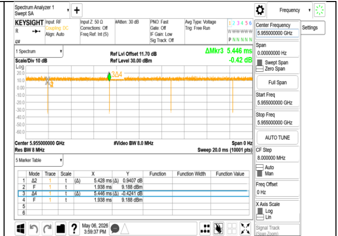
802.11n_20MHz_Chain0_5955MHz
