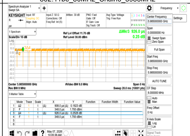
802.11be_80MHz_Chain0_5985MHz_RU996
