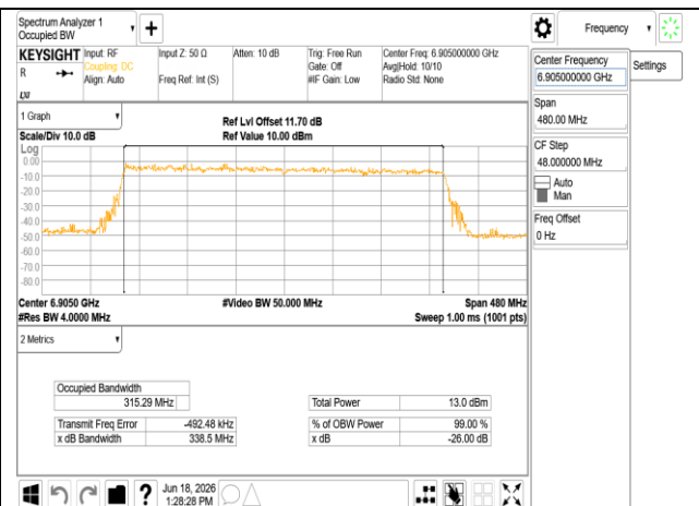
802.11be_320MHz_Chain1_6905MHz_RU996x4
