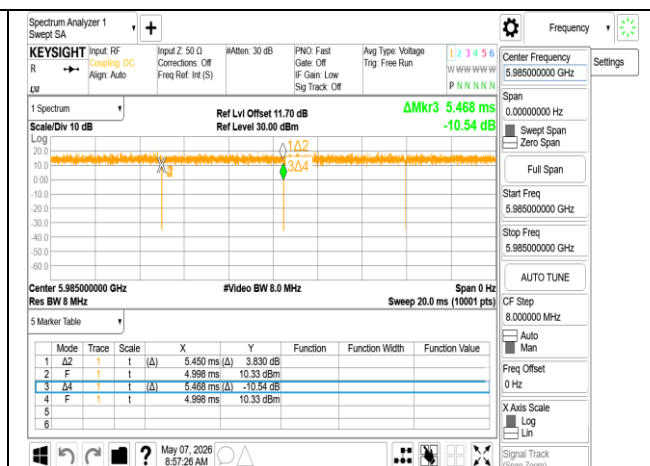
802.11be_80MHz_Chain0_5985MHz
