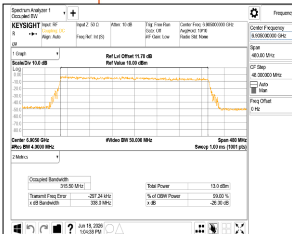
802.11be_320MHz_Chain1_6905MHz
