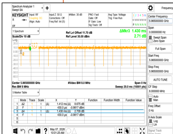
802.11be_40MHz_Chain0_5965MHz_RU484
