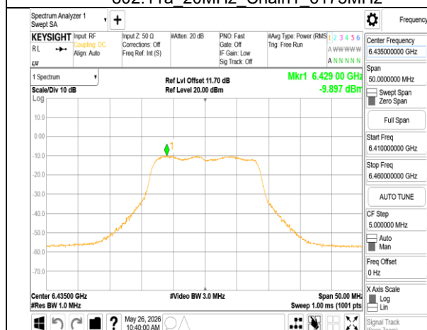
802.11a_20MHz_Chain1_6435MHz
