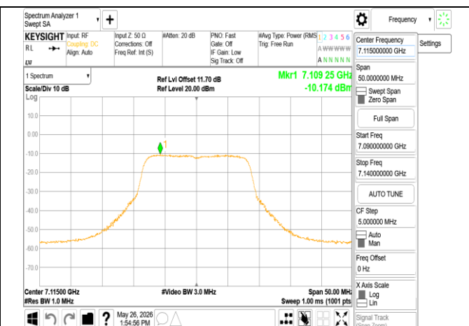
802.11a_20MHz_Chain1_7115MHz
