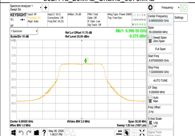
802.11a_20MHz_Chain0_6995MHz
