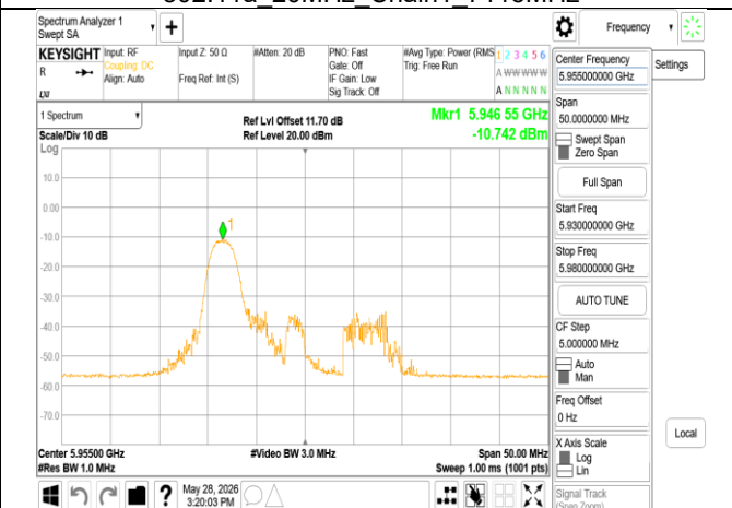
802.11ax_20MHz_Chain0_5955MHz_RU26_0
