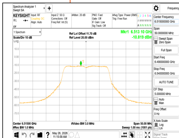
802.11a_20MHz_Chain1_6515MHz
