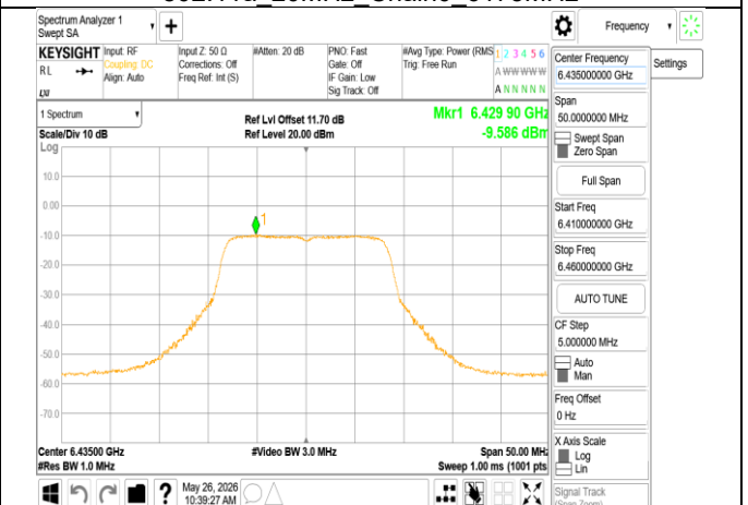
802.11a_20MHz_Chain0_6435MHz
