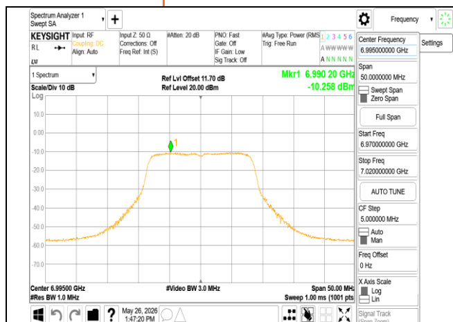
802.11a_20MHz_Chain1_6995MHz
