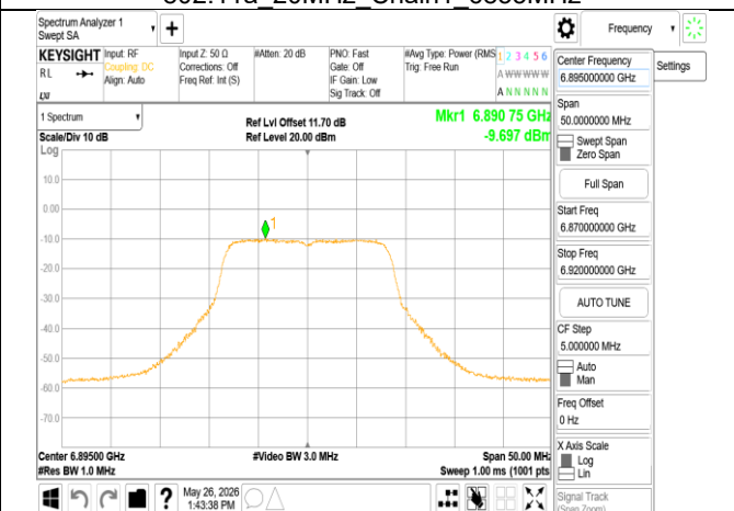
802.11a_20MHz_Chain1_6895MHz
