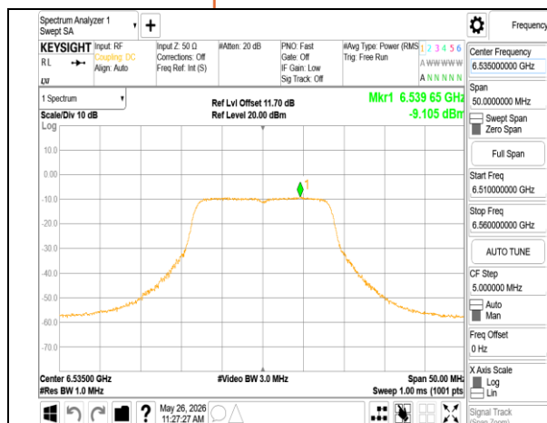
802.11a_20MHz_Chain0_6535MHz
