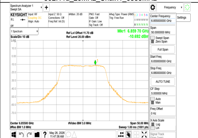
802.11a_20MHz_Chain1_6855MHz
