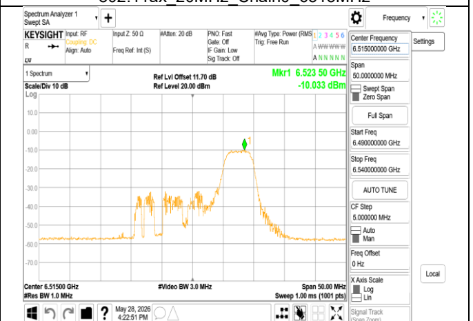
802.11ax 20MHz Chain0 6515MHz RU52_40
