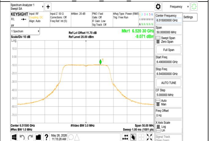
802.11a_20MHz_Chain0_6515MHz
