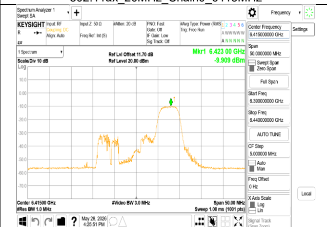
802.11ax 20MHz Chain0 6415MHz RU52_40
