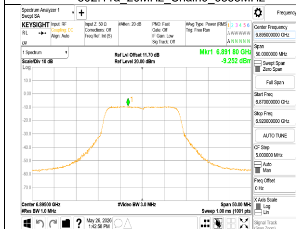
802.11a_20MHz_Chain0_6895MHz
