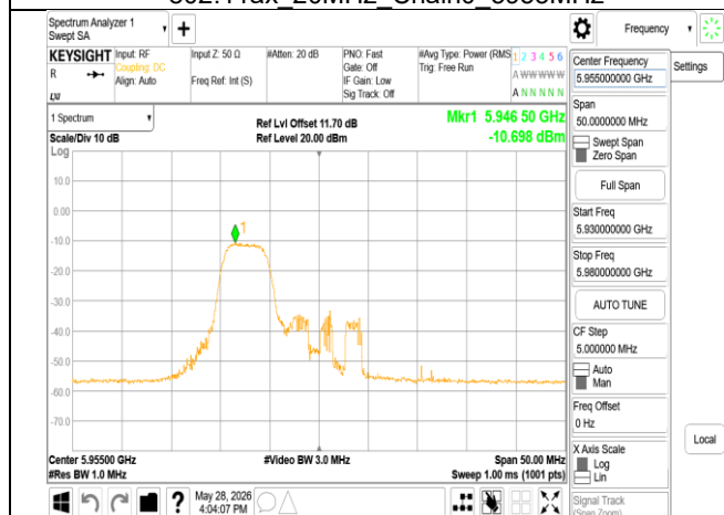
802.11ax_20MHz_Chain0_5955MHz_RU52_37
