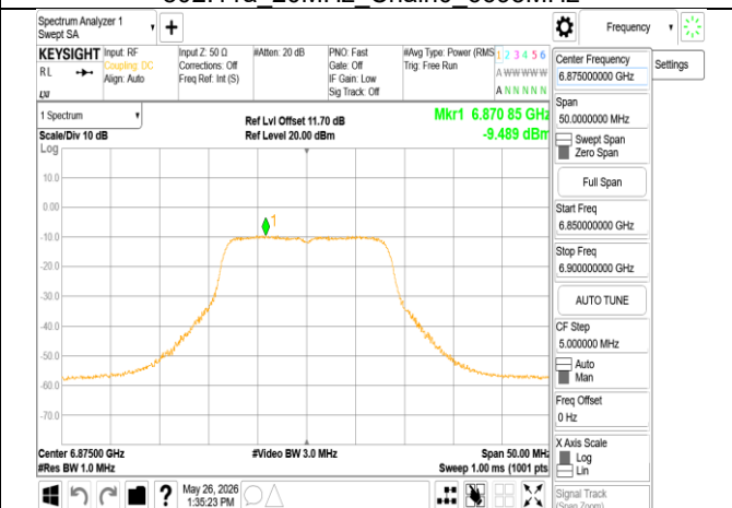
802.11a_20MHz_Chain0_6875MHz
