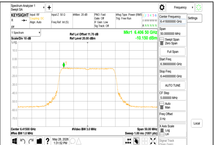
802.11ax 20MHz Chain0 6415MHz RU242
