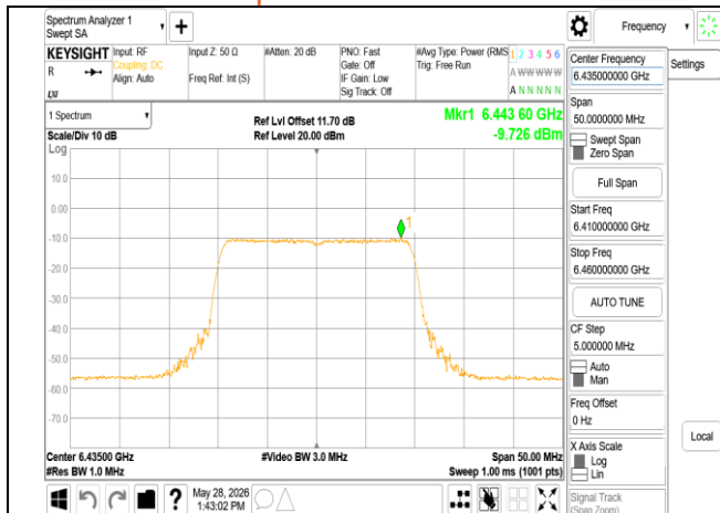
802.11ax 20MHz Chain0 6435MHz RU242
