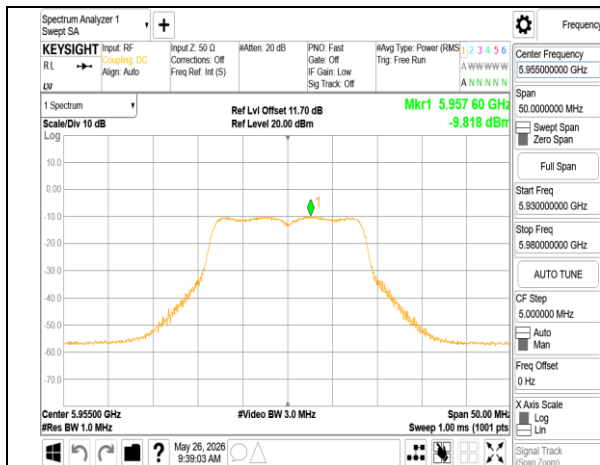
802.11a_20MHz_Chain0_5955MHz
