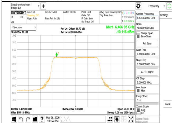
802.11ax 20MHz Chain0 6475MHz RU242
