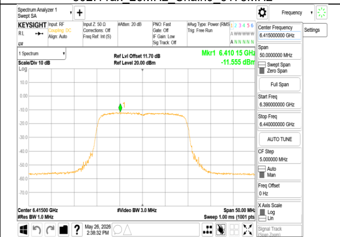
802.11ax 20MHz Chain0 6415MHz
