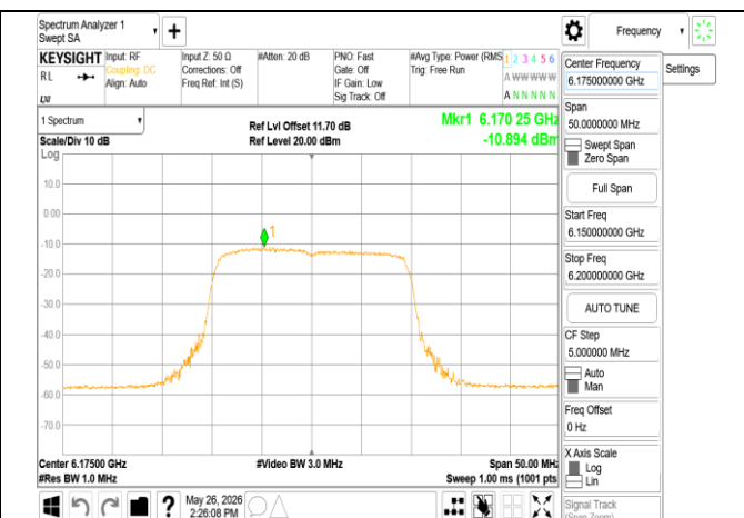
802.11ax 20MHz Chain0 6175MHz
