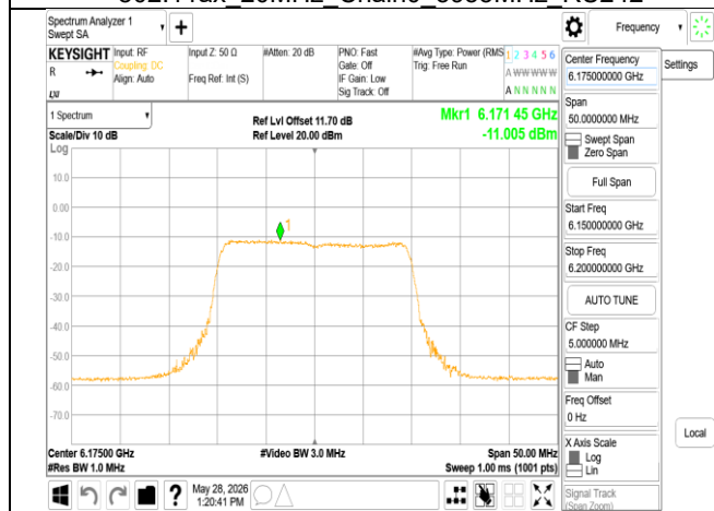
802.11ax 20MHz Chain0 6175MHz RU242
