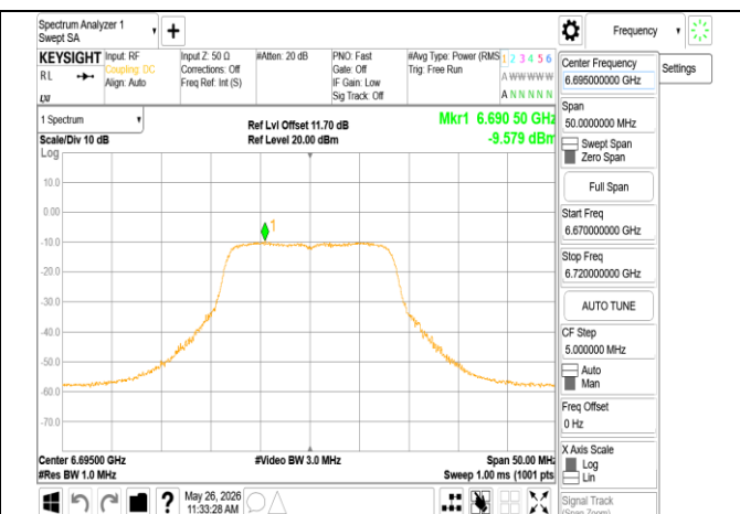
802.11a_20MHz_Chain0_6695MHz
