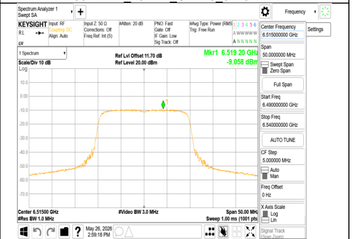
802.11ax 20MHz Chain0 6515MHz
