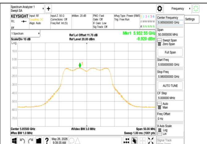
802.11a_20MHz_Chain1_5955MHz
