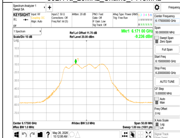
802.11a_20MHz_Chain1_6175MHz
