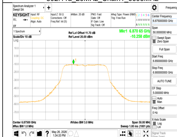
802.11a_20MHz_Chain1_6875MHz
