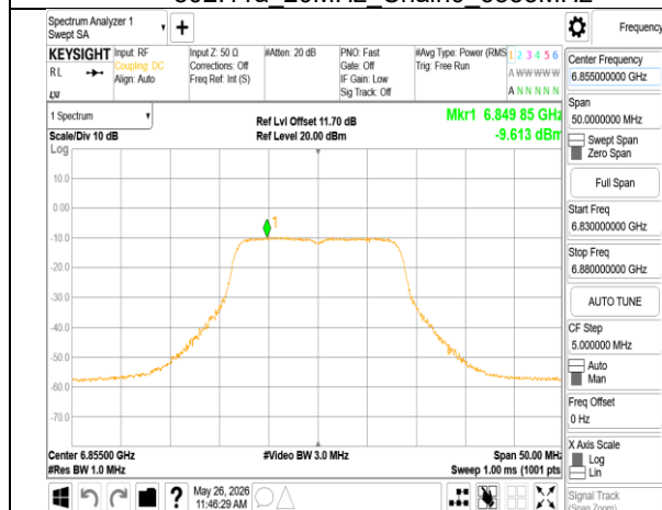
802.11a_20MHz_Chain0_6855MHz
