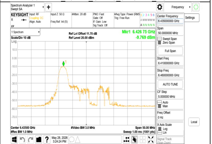
802.11ax 20MHz Chain0 6435MHz RU26_0
