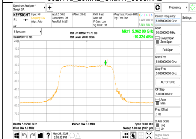
802.11ax_20MHz_Chain0_5955MHz
