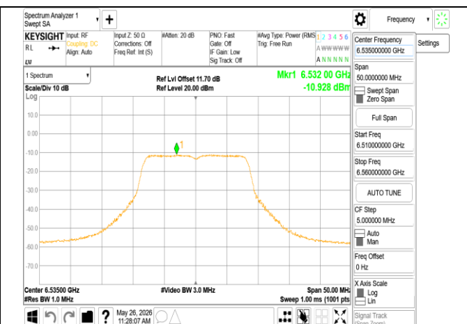
802.11a_20MHz_Chain1_6535MHz
