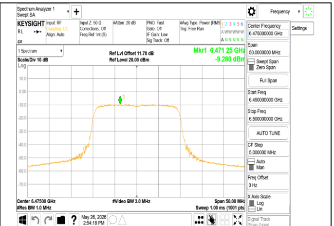
802.11ax 20MHz Chain0 6475MHz
