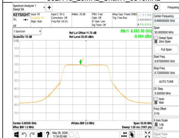
802.11a_20MHz_Chain1_6695MHz
