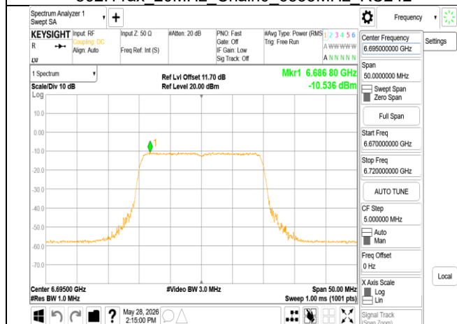
802.11ax 20MHz Chain0 6695MHz RU242
