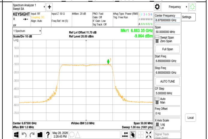
802.11ax 20MHz Chain0 6875MHz RU242
