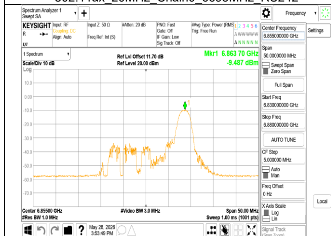
802.11ax 20MHz Chain0 6855MHz RU26_8
