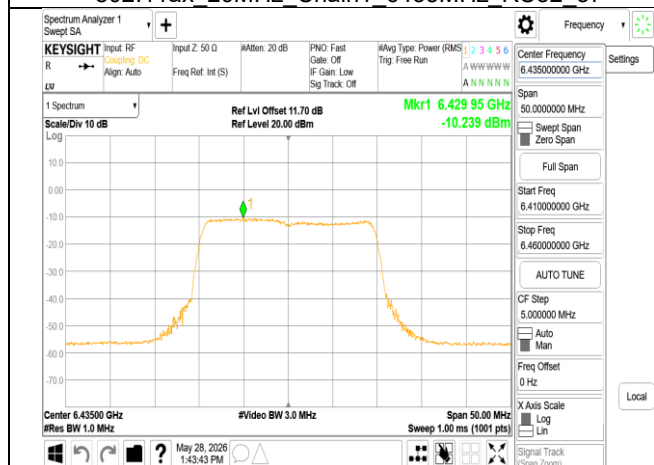
802.11ax 20MHz Chain1 6435MHz RU242
