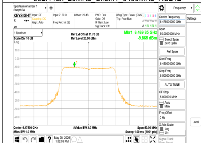
802.11ax 20MHz Chain1 6475MHz RU242
