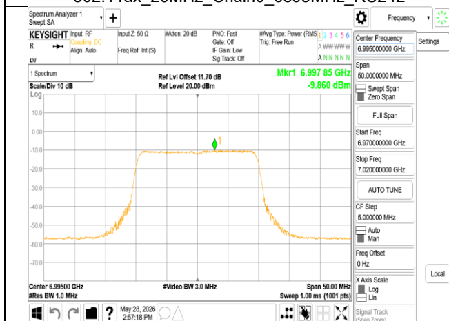
802.11ax 20MHz Chain0 6995MHz RU242
