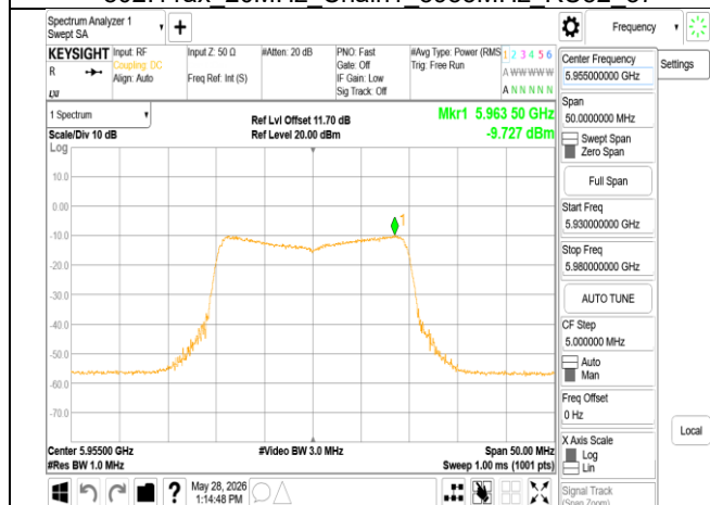
802.11ax 20MHz Chain1 5955MHz RU242
