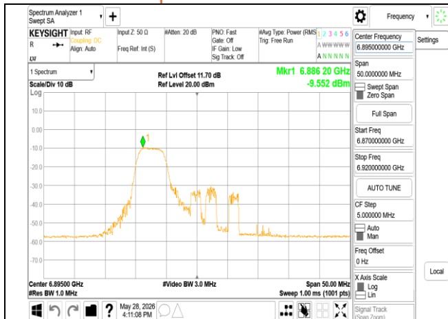
802.11ax 20MHz Chain0 6895MHz RU52 37
