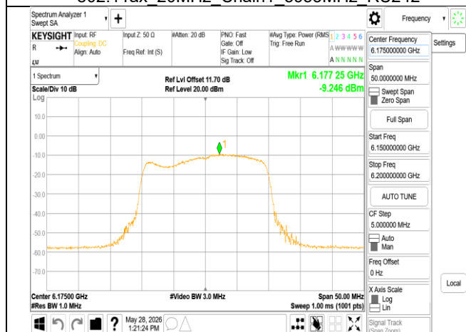
802.11ax 20MHz Chain1 6175MHz RU242
