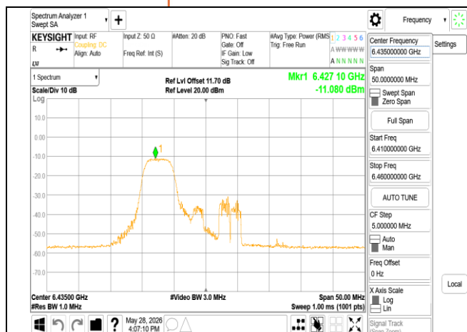
802.11ax 20MHz Chain1 6435MHz RU52 37
