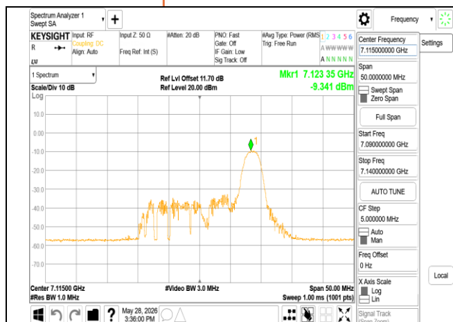
802.11ax 20MHz Chain0 7115MHz RU26 8
