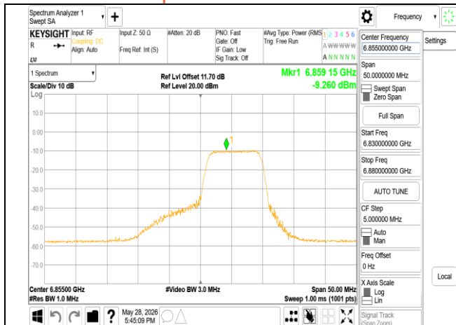
802.11ax 20MHz Chain0 6855MHz RU106_54
