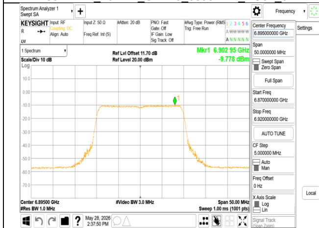
802.11ax 20MHz Chain0 6895MHz RU242
