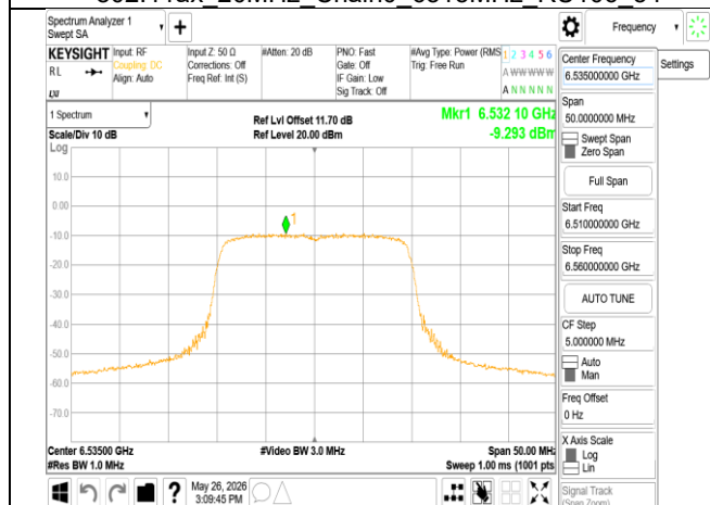
802.11ax 20MHz Chain0 6535MHz
