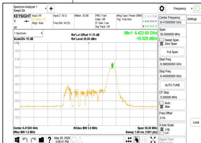
802.11ax 20MHz Chain1 6415MHz RU26 8
