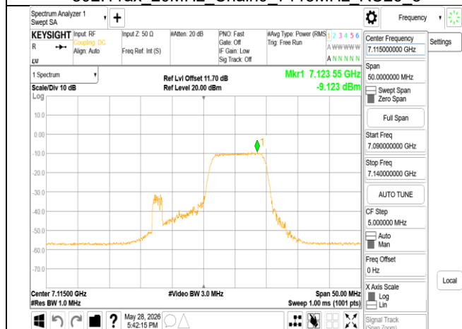
802.11ax 20MHz Chain0 7115MHz RU106 54
