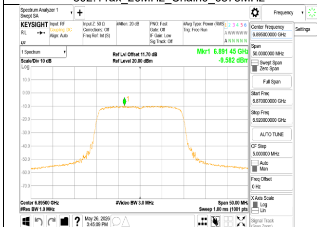
802.11ax 20MHz Chain0 6895MHz
