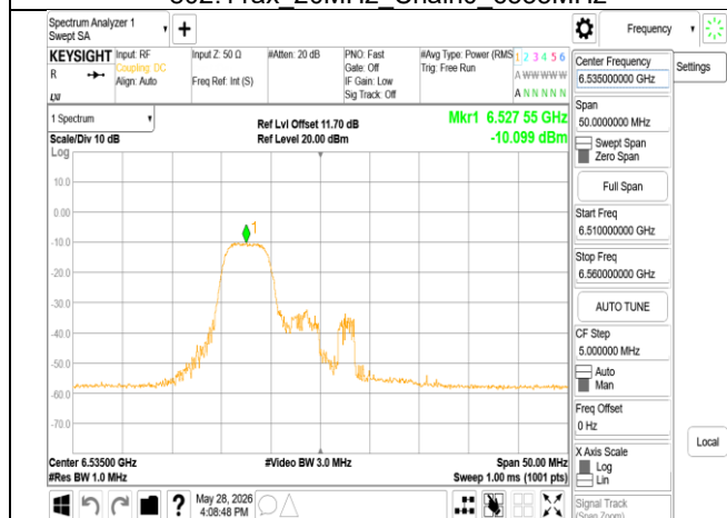
802.11ax 20MHz Chain0 6535MHz RU52_37
