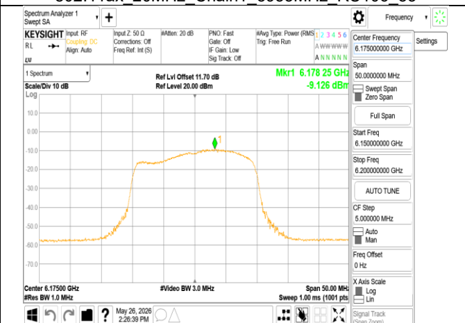
802.11ax 20MHz Chain1 6175MHz
