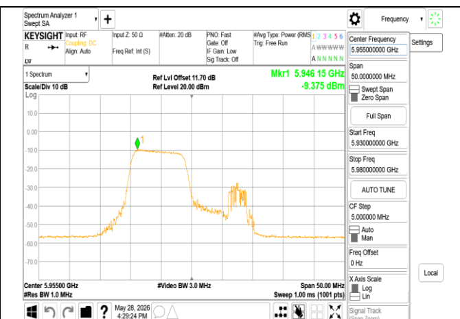
802.11ax 20MHz Chain1 5955MHz RU106 53
