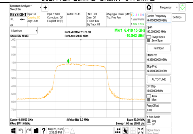
802.11ax 20MHz Chain1 6415MHz
