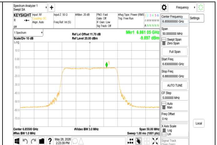
802.11ax 20MHz Chain0 6855MHz RU242
