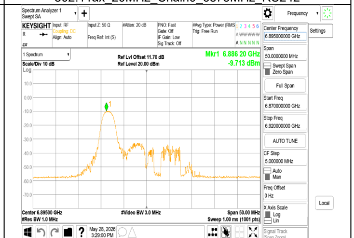
802.11ax 20MHz Chain0 6895MHz RU26_0
