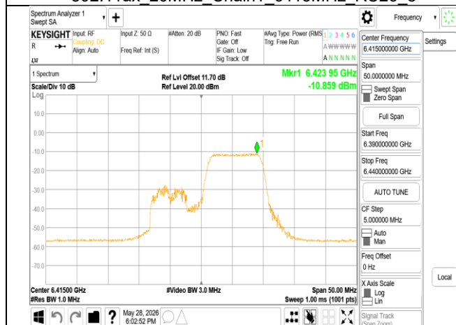
802.11ax 20MHz Chain1 6415MHz RU106 54
