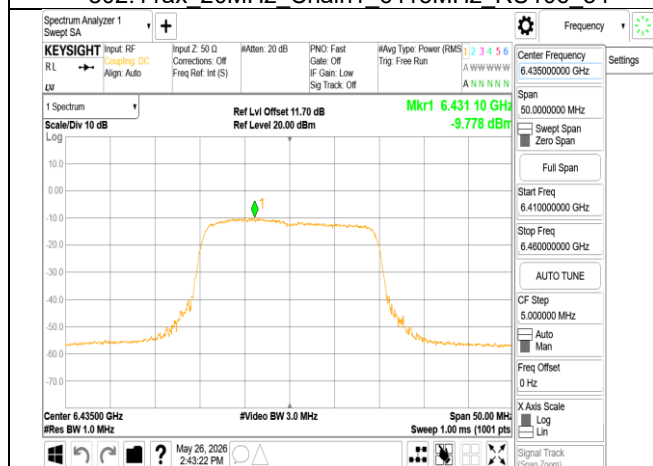
802.11ax 20MHz Chain1 6435MHz
