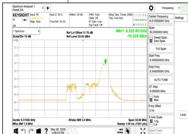
802.11ax 20MHz Chain1 6515MHz RU26_8
