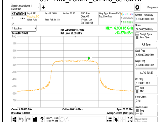
802.11ax 20MHz Chain0 6895MHz
