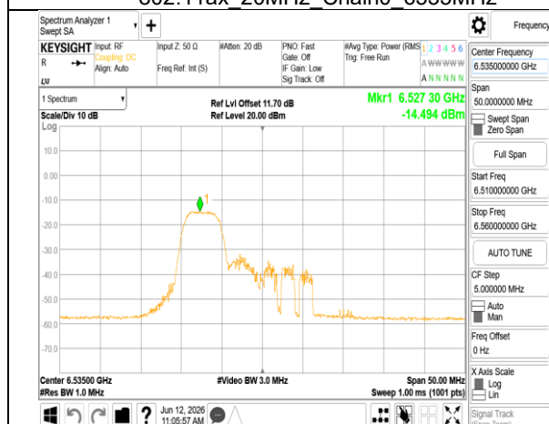
802.11ax 20MHz Chain0 6535MHz RU52_37
