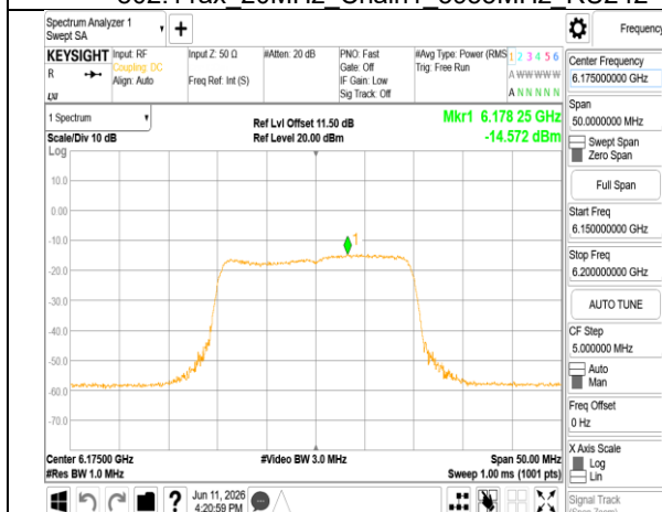
802.11ax 20MHz Chain1 6175MHz RU242
