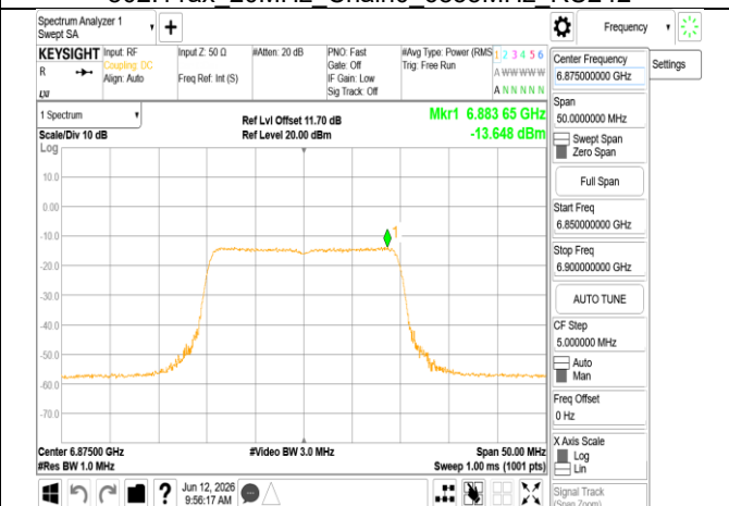
802.11ax 20MHz Chain0 6875MHz RU242
