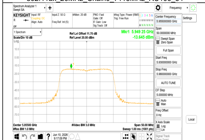
802.11ax 20MHz Chain1 5955MHz
