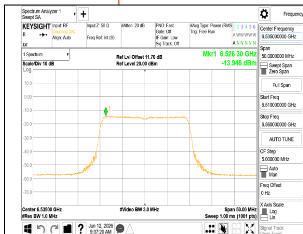
802.11ax 20MHz Chain0 6535MHz RU242
