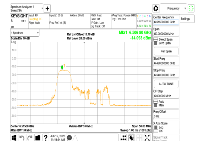
802.11ax 20MHz Chain1 6515MHz RU52_40
