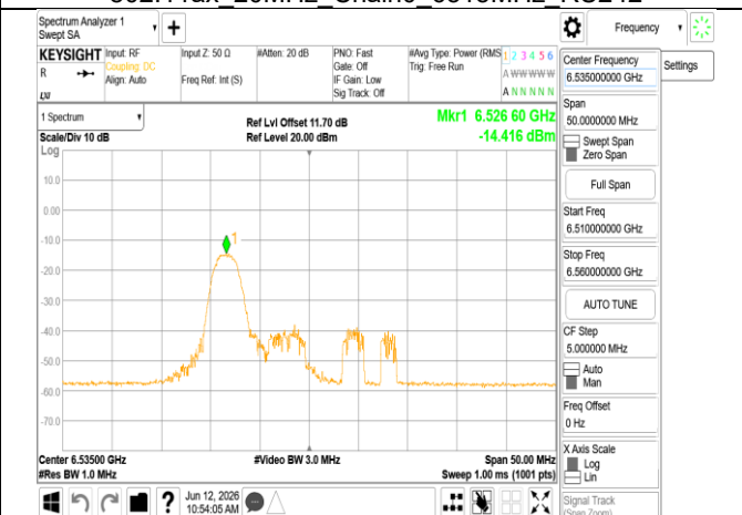
802.11ax 20MHz Chain0 6535MHz RU26_0
