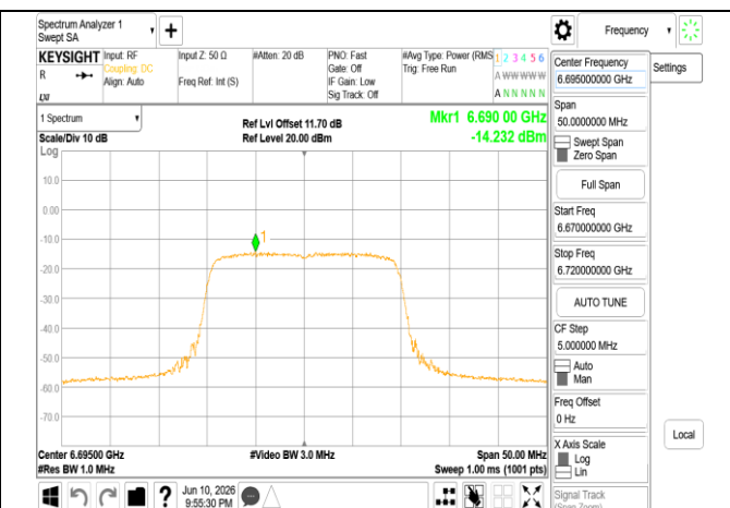
802.11ax 20MHz Chain0 6695MHz
