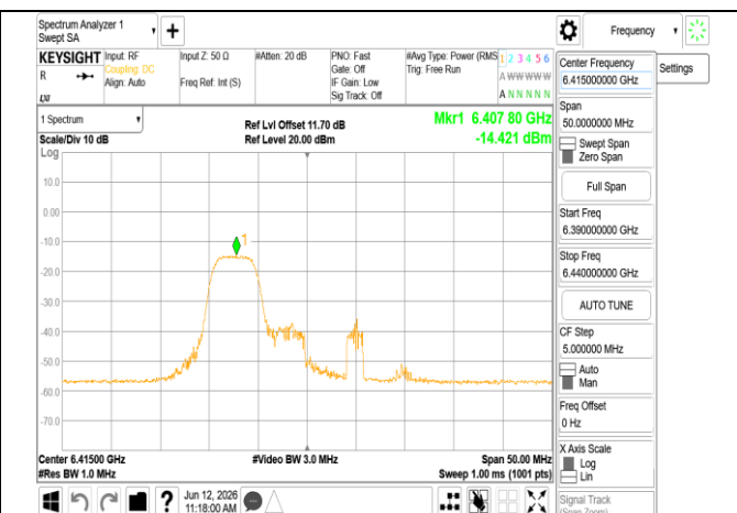
802.11ax 20MHz Chain1 6415MHz RU52 40
