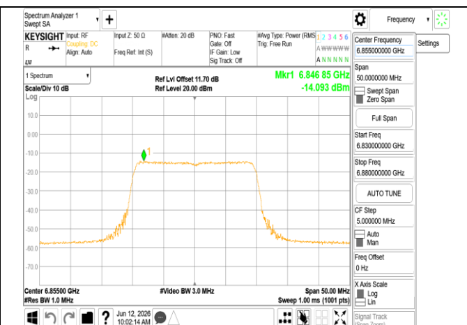
802.11ax 20MHz Chain0 6855MHz RU242
