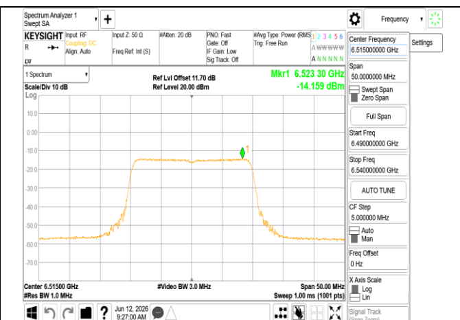
802.11ax 20MHz Chain0 6515MHz RU242
