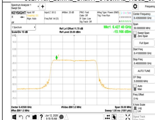
802.11ax 20MHz Chain1 6435MHz RU242
