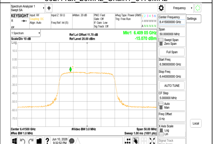
802.11ax 20MHz Chain1 6415MHz
