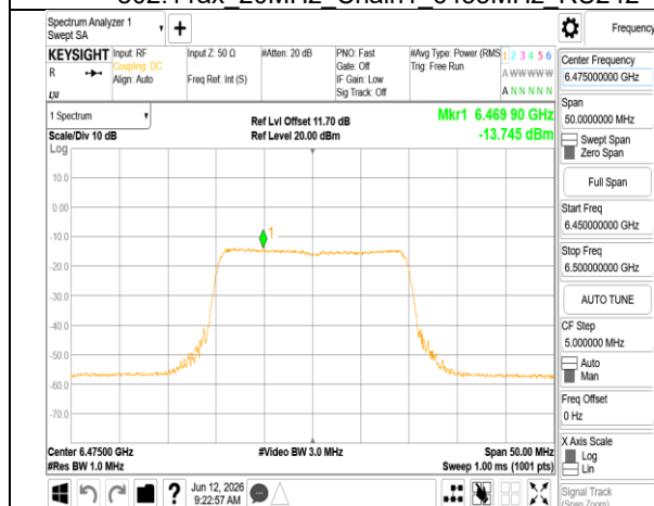
802.11ax 20MHz Chain1 6475MHz RU242
