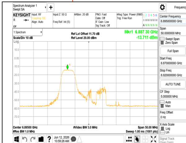
802.11ax 20MHz Chain0 6895MHz RU52 37
