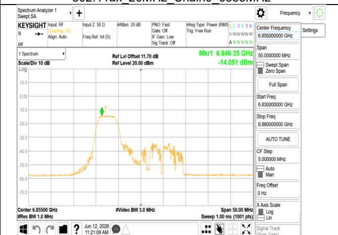
802.11ax 20MHz Chain0 6855MHz RU52_40
