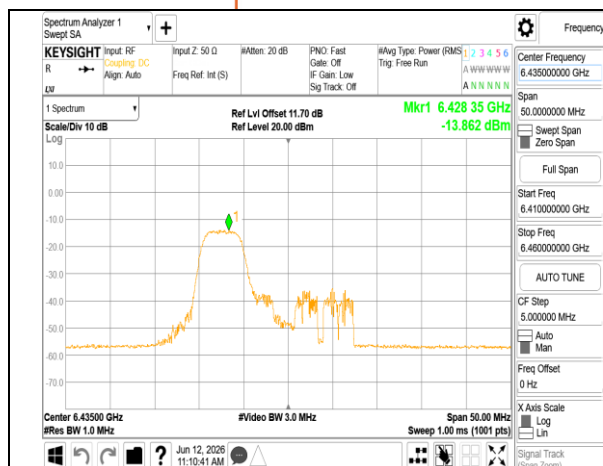
802.11ax 20MHz Chain1 6435MHz RU52 37
