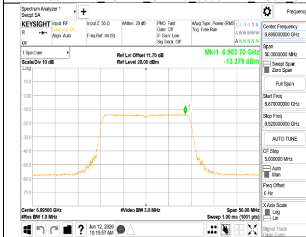
802.11ax 20MHz Chain0 6895MHz RU242
