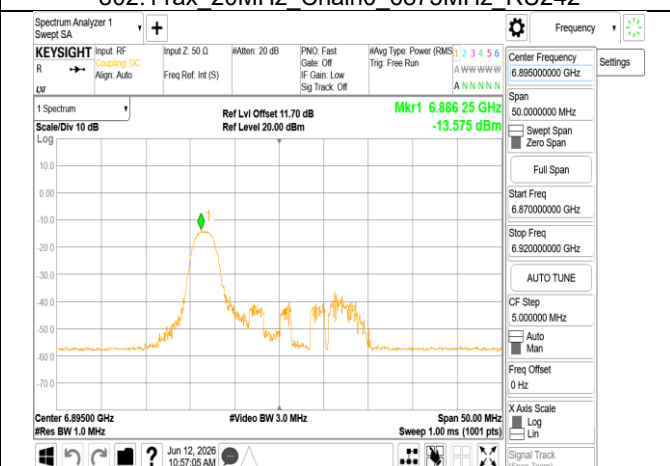
802.11ax 20MHz Chain0 6895MHz RU26_0
