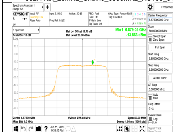
802.11ax 20MHz Chain0 6875MHz
