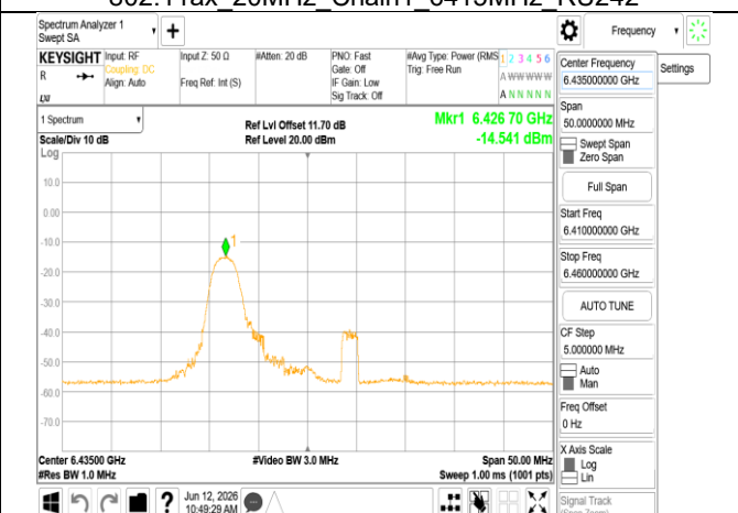
802.11ax 20MHz Chain1 6435MHz RU26 0
