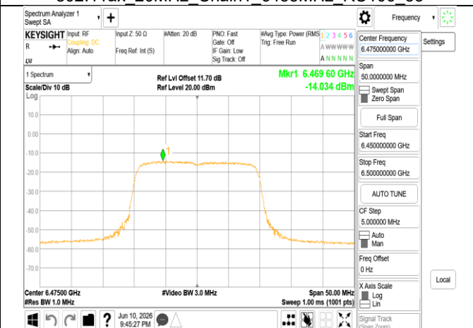
802.11ax 20MHz Chain1 6475MHz
