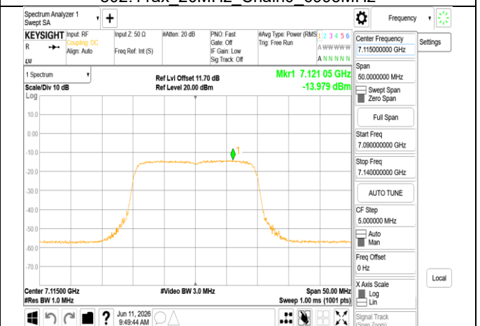
802.11ax 20MHz Chain0 7115MHz
