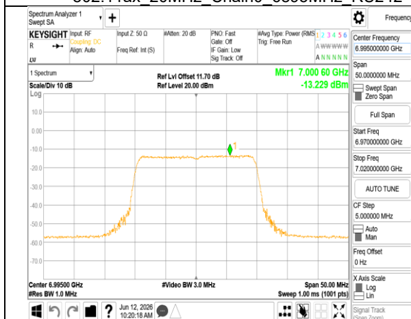
802.11ax 20MHz Chain0 6995MHz RU242
