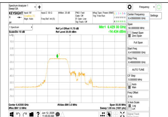
802.11ax 20MHz Chain1 6435MHz RU106 53
