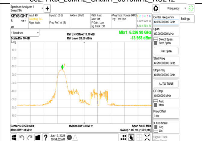
802.11ax 20MHz Chain1 6535MHz RU26_0
