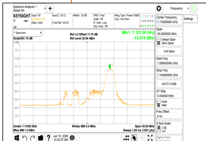
802.11ax 20MHz Chain0 7115MHz RU26 8
