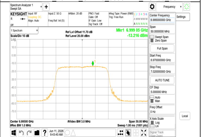
802.11ax 20MHz Chain0 6995MHz
