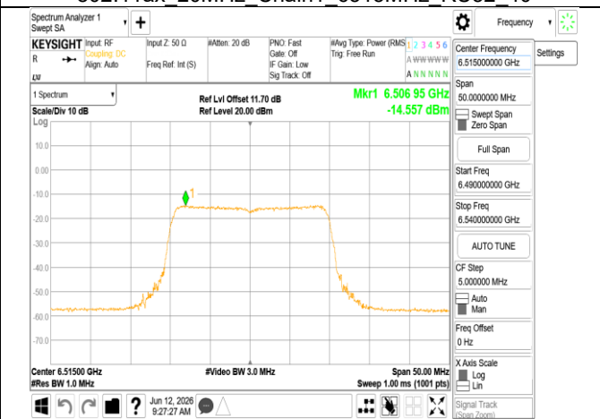
802.11ax 20MHz Chain1 6515MHz RU242
