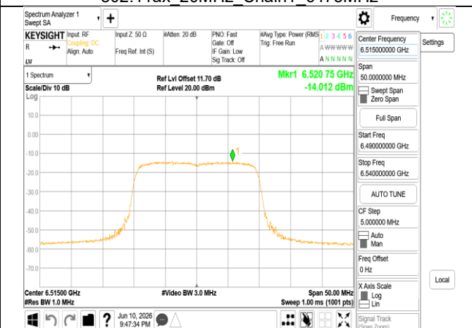
802.11ax 20MHz Chain1 6515MHz
