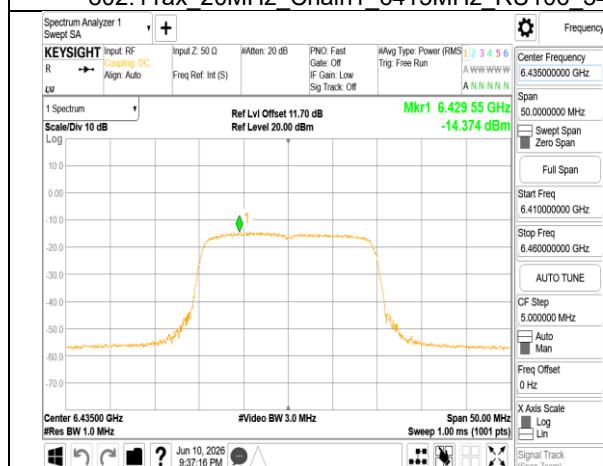
802.11ax 20MHz Chain1 6435MHz
