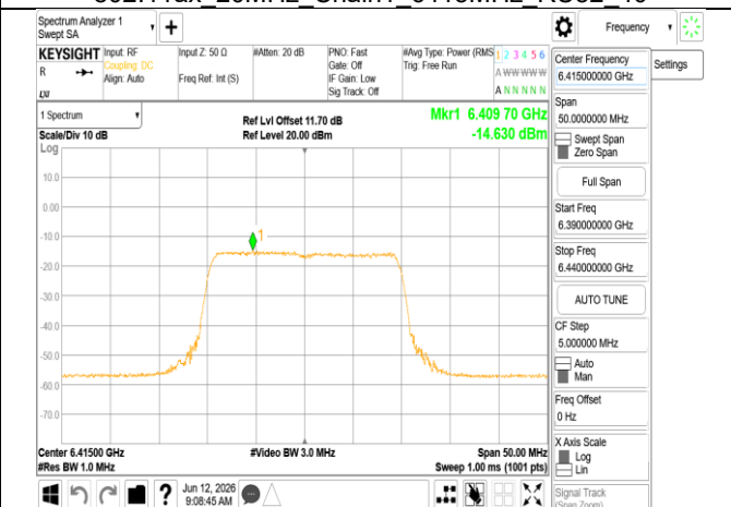
802.11ax 20MHz Chain1 6415MHz RU242
