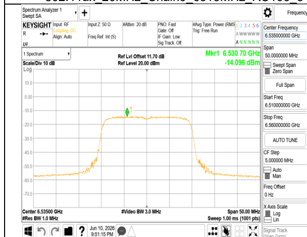
802.11ax 20MHz Chain0 6535MHz
