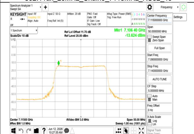
802.11ax 20MHz Chain0 7115MHz RU242
