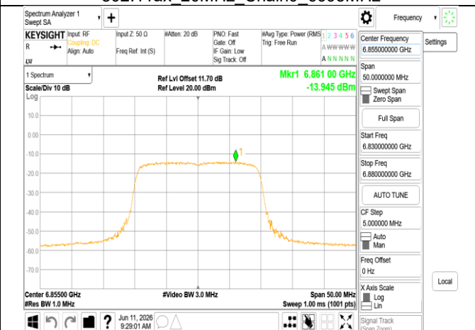
802.11ax 20MHz Chain0 6855MHz
