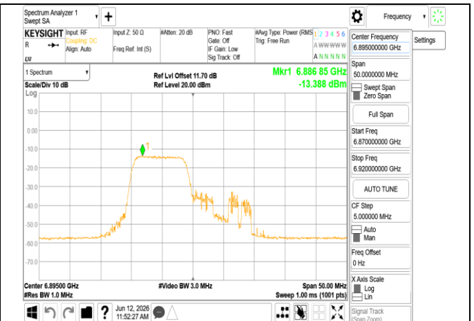
802.11ax 20MHz Chain0 6895MHz RU106 53
