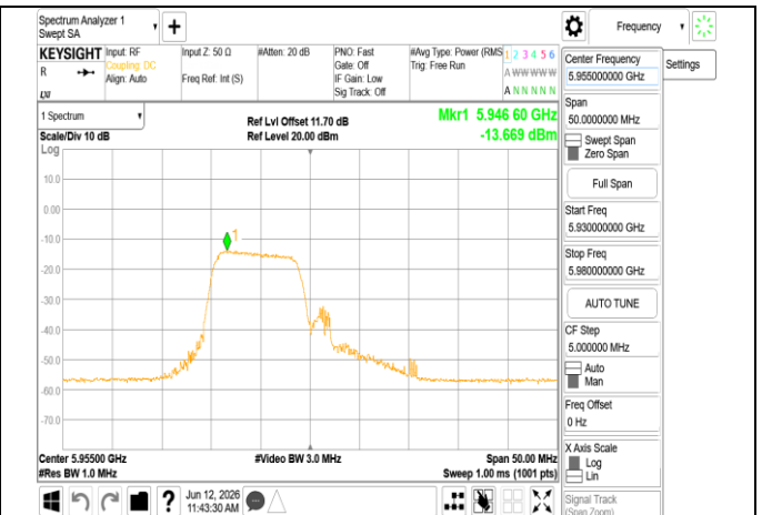
802.11ax 20MHz Chain1 5955MHz RU106 53
