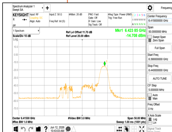
802.11ax 20MHz Chain1 6415MHz RU26 8
