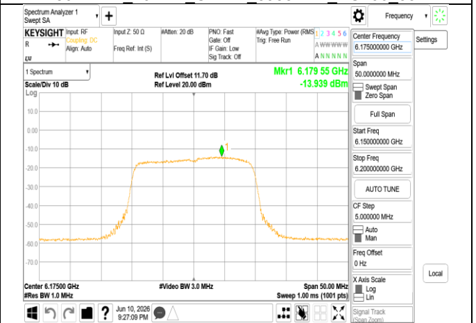
802.11ax 20MHz Chain1 6175MHz
