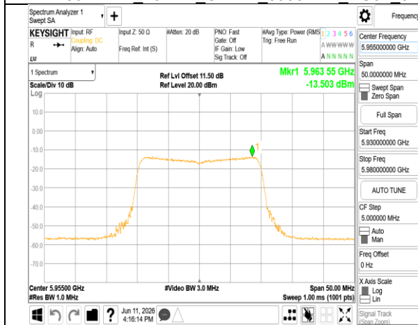
802.11ax 20MHz Chain1 5955MHz RU242
