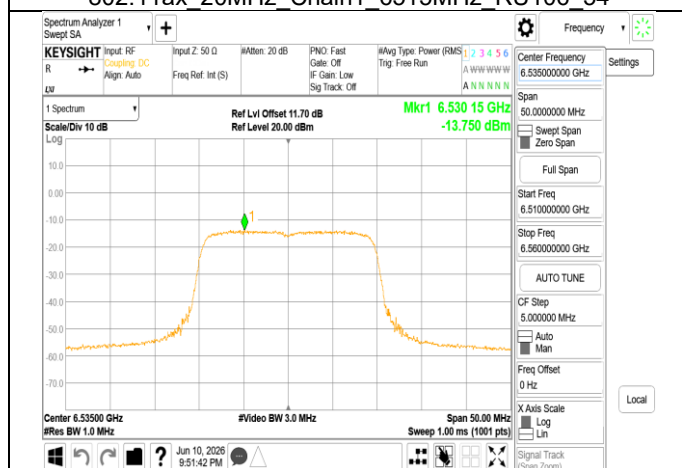
802.11ax 20MHz Chain1 6535MHz
