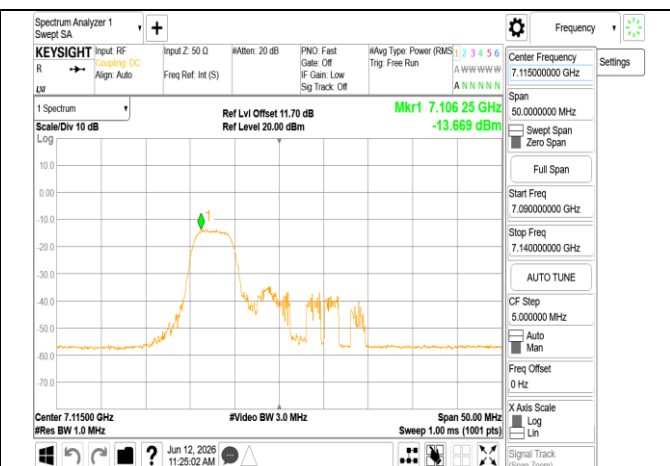
802.11ax 20MHz Chain0 7115MHz RU52 40
