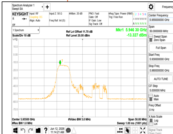
802.11ax 20MHz Chain1 5955MHz RU52 37
