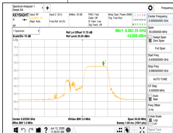
802.11ax 20MHz Chain0 6855MHz RU106_54
