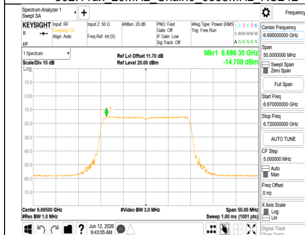
802.11ax 20MHz Chain0 6695MHz RU242
