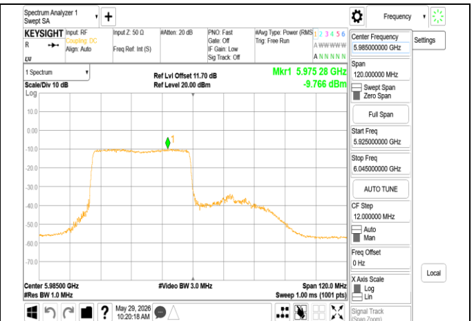
802.11ax 80MHz Chain0 5985MHz RU484 65
