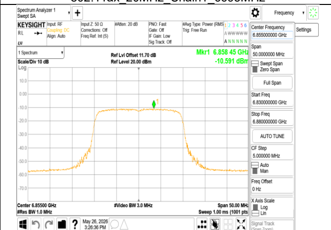
802.11ax 20MHz Chain1 6855MHz
