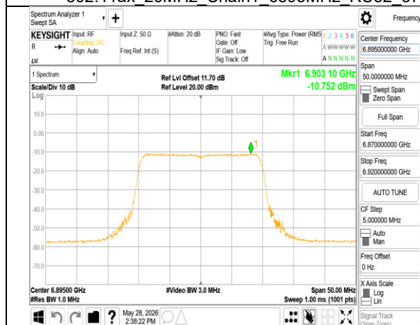
802.11ax 20MHz Chain1 6895MHz RU242
