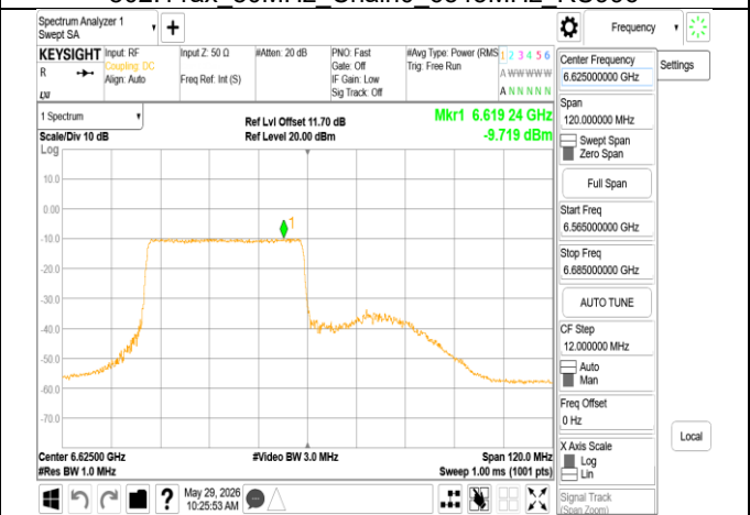
802.11ax 80MHz Chain0 6625MHz RU484 65
