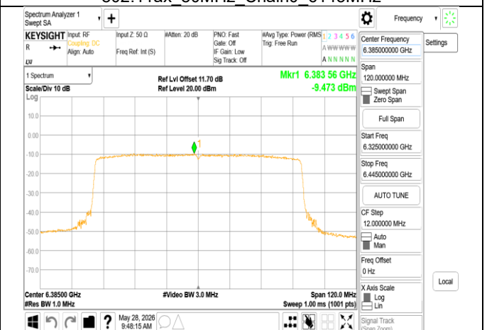
802.11ax 80MHz Chain0 6385MHz
