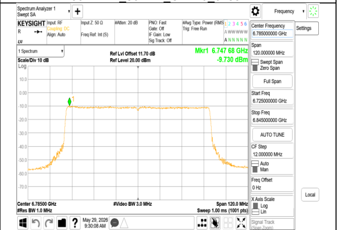
802.11ax 80MHz Chain0 6785MHz RU996
