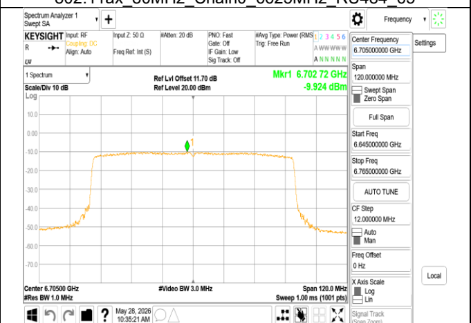
802.11ax 80MHz Chain0 6705MHz
