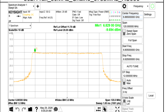
802.11ax 80MHz Chain0 6865MHz RU996
