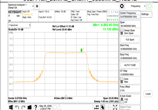
802.11ax 20MHz Chain1 6875MHz RU242
