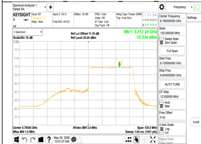
802.11ax 80MHz Chain0 6785MHz RU484 66
