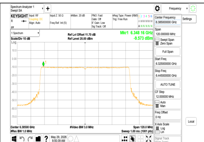
802.11ax 80MHz Chain0 6385MHz RU996
