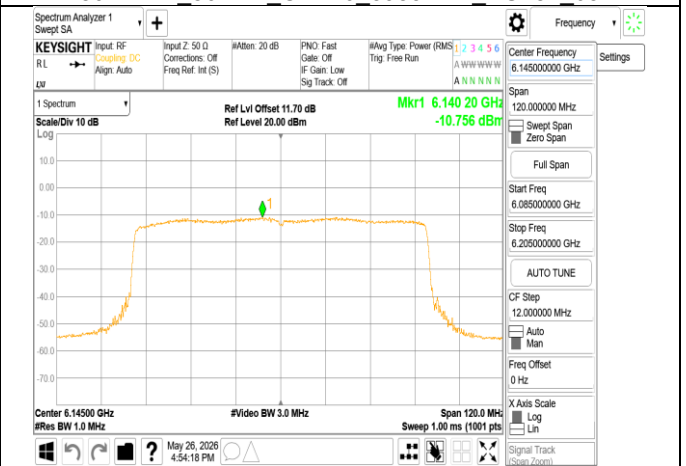
802.11ax 80MHz Chain0 6145MHz
