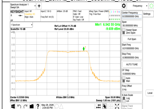
802.11ax 20MHz Chain1 6535MHz RU242
