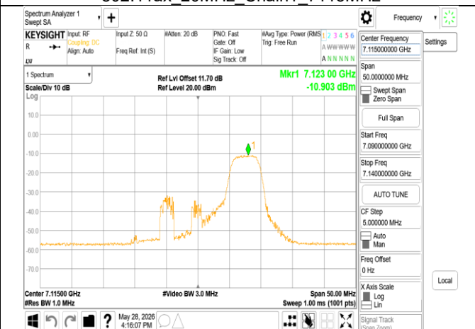
802.11ax 20MHz Chain1 7115MHz RU52_40
