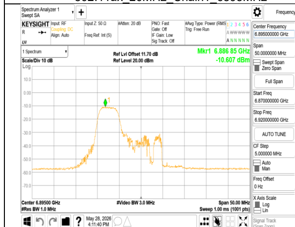
802.11ax 20MHz Chain1 6895MHz RU52 37
