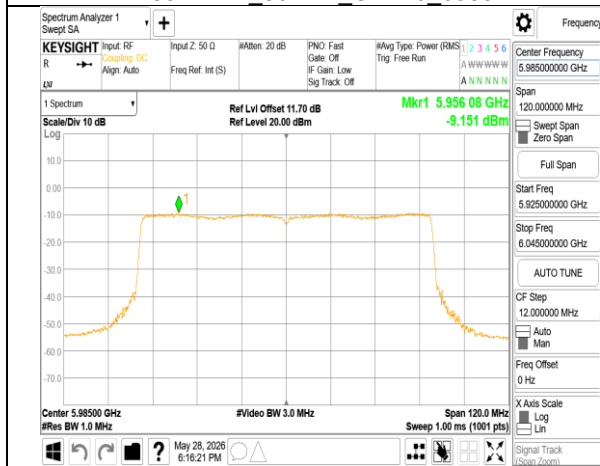
802.11ax 80MHz Chain0 5985MHz RU996
