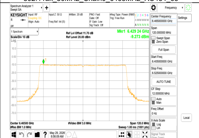
802.11ax 80MHz Chain0 6465MHz RU996
