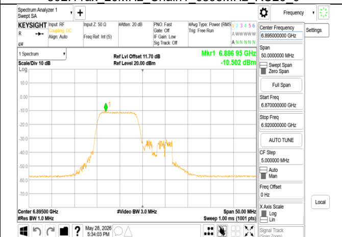
802.11ax 20MHz Chain1 6895MHz RU106 53
