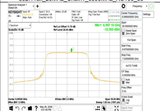
802.11ax 20MHz Chain1 6995MHz
