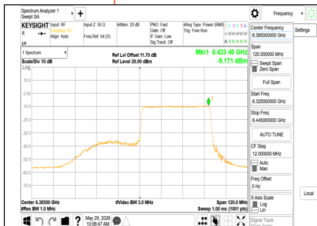
802.11ax 80MHz Chain0 6385MHz RU484 66
