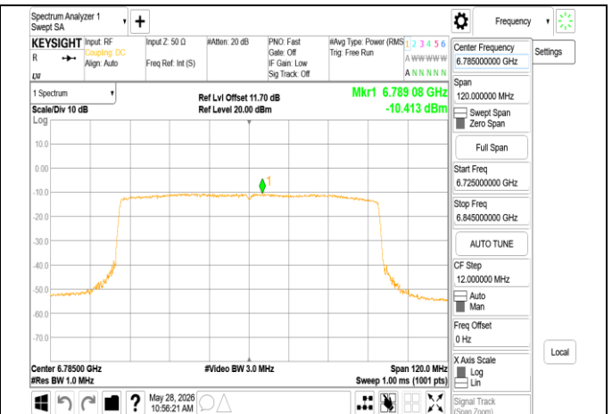
802.11ax 80MHz Chain0 6785MHz
