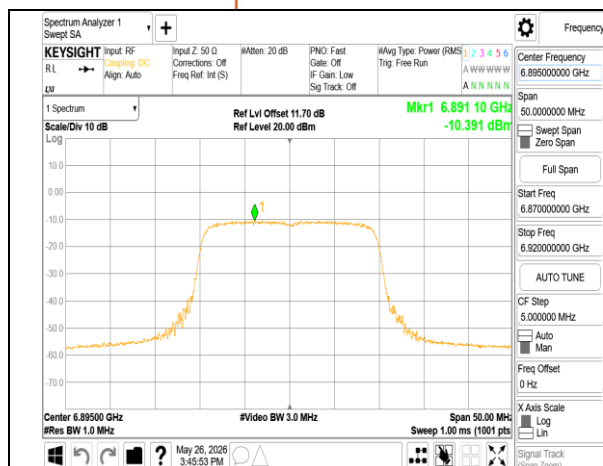
802.11ax 20MHz Chain1 6895MHz
