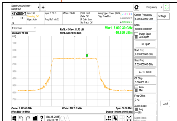
802.11ax 20MHz Chain1 6995MHz RU242
