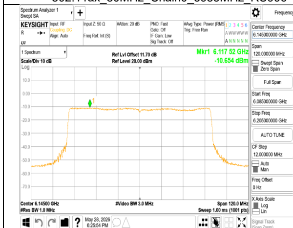
802.11ax 80MHz Chain0 6145MHz RU996
