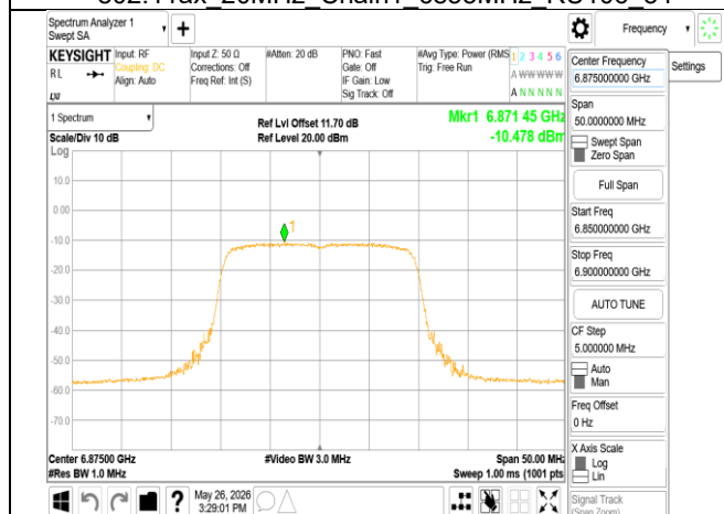
802.11ax 20MHz Chain1 6875MHz
