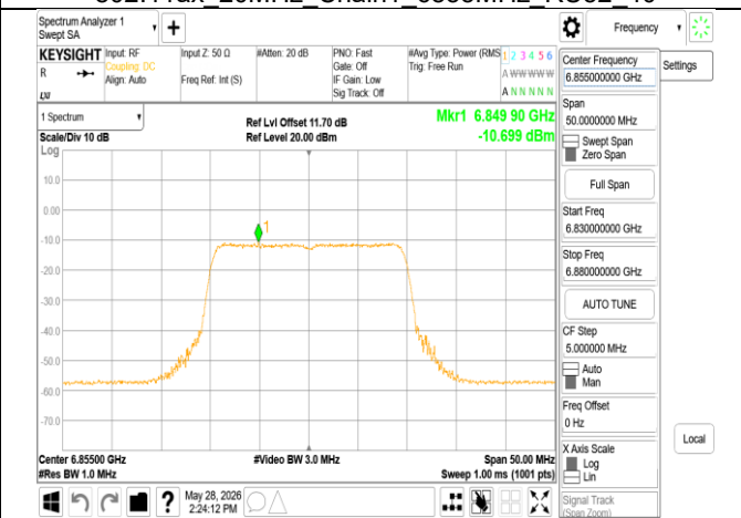
802.11ax 20MHz Chain1 6855MHz RU242
