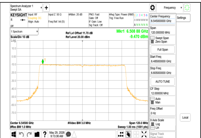
802.11ax 80MHz Chain0 6545MHz RU996
