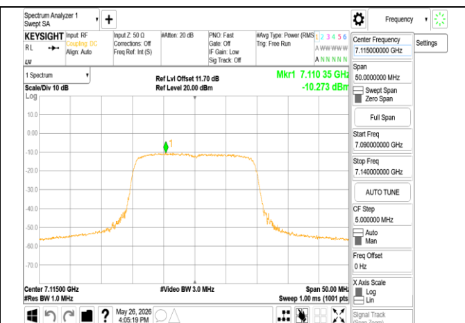
802.11ax 20MHz Chain1 7115MHz
