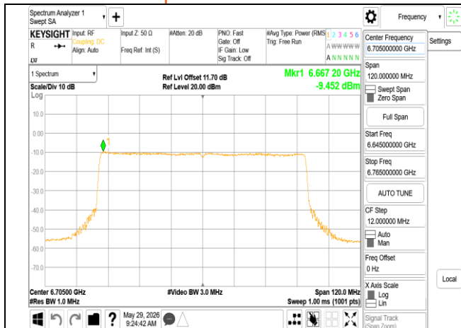
802.11ax 80MHz Chain0 6705MHz RU996
