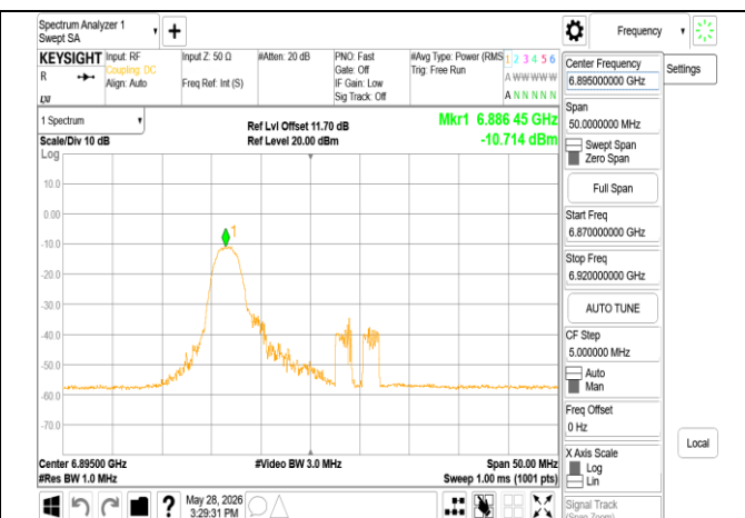
802.11ax 20MHz Chain1 6895MHz RU26 0
