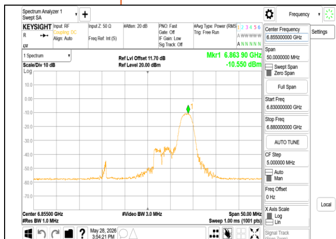
802.11ax 20MHz Chain1 6855MHz RU26_8
