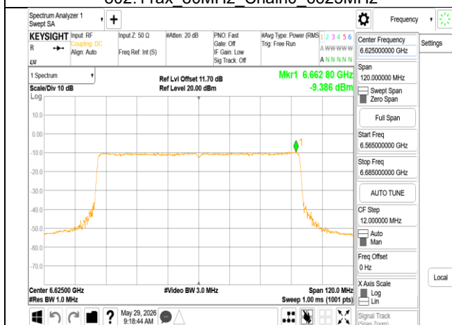
802.11ax 80MHz Chain0 6625MHz RU996
