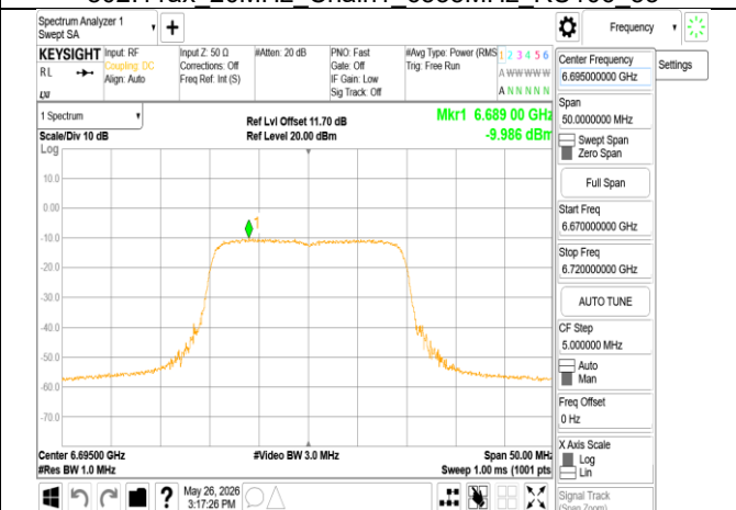
802.11ax 20MHz Chain1 6695MHz
