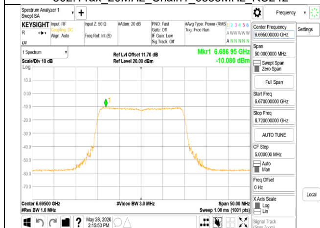
802.11ax 20MHz Chain1 6695MHz RU242
