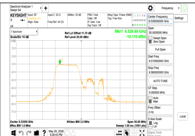
802.11ax 20MHz Chain1 6535MHz RU106 53
