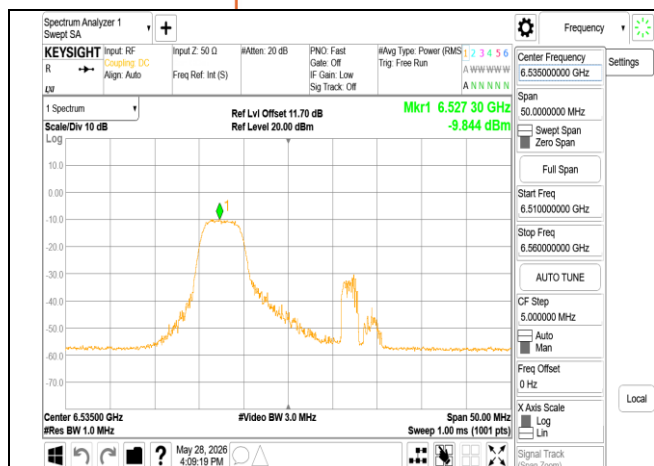
802.11ax 20MHz Chain1 6535MHz RU52 37
