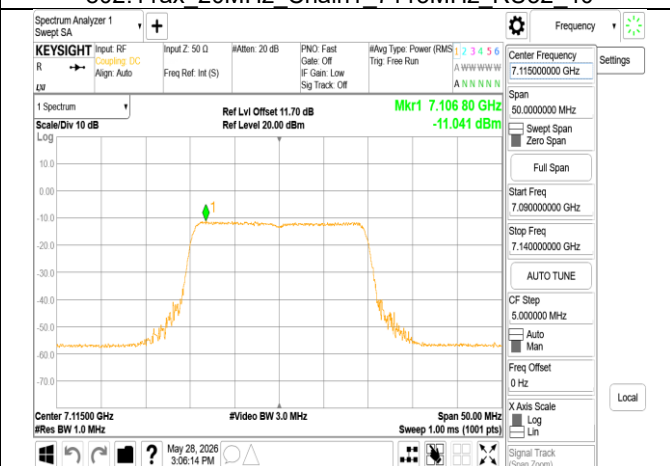
802.11ax 20MHz Chain1 7115MHz RU242
