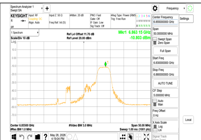
802.11ax 20MHz Chain1 6855MHz RU52_40
