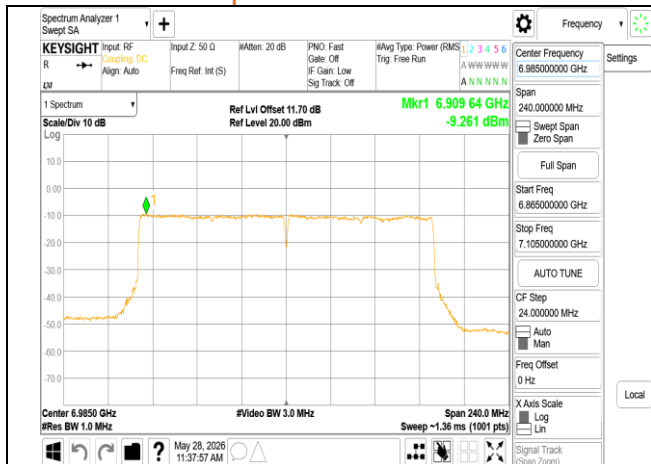
802.11ax_160MHz_Chain0_6985MHz
