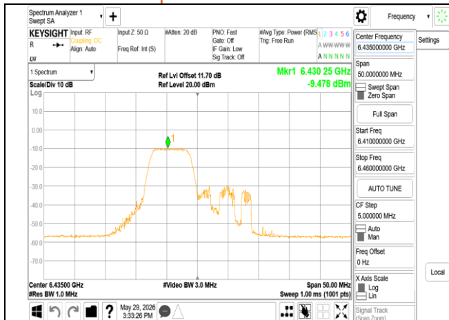
802.11be 20MHz Chain0 6435MHz 52+26 MRU1
