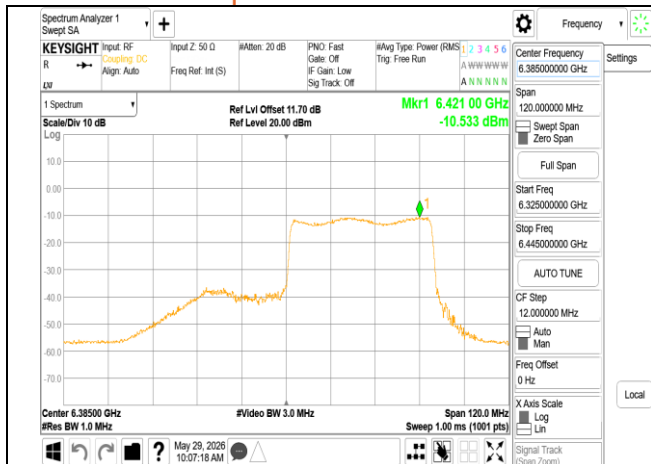
802.11ax 80MHz Chain1 6385MHz RU484 66
