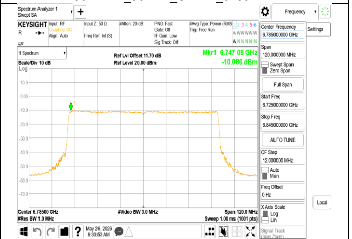
802.11ax 80MHz Chain1 6785MHz RU996
