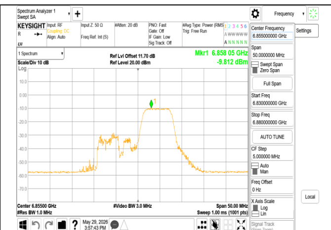
802.11be_20MHz_Chain0_6855MHz_52+26_MR03
