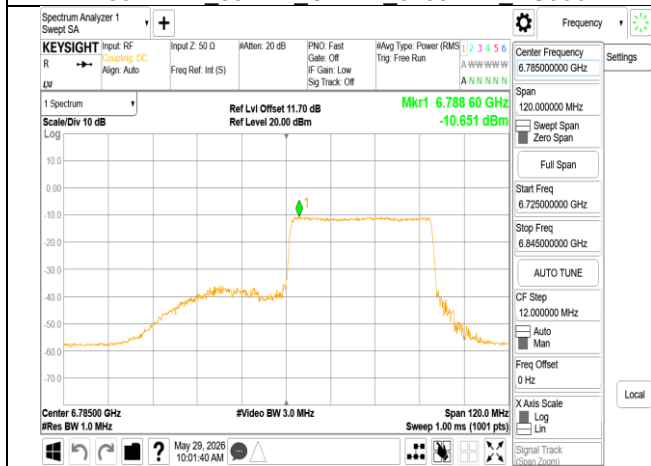
802.11ax 80MHz Chain1 6785MHz RU484 66
