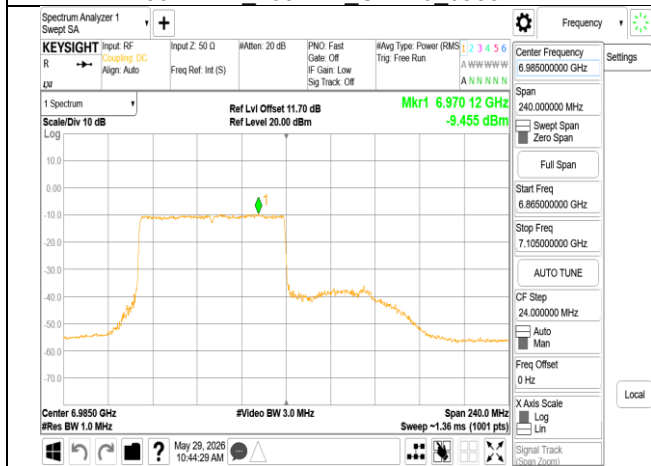
802.11ax_160MHz_Chain0_6985MHz_RU996_67
