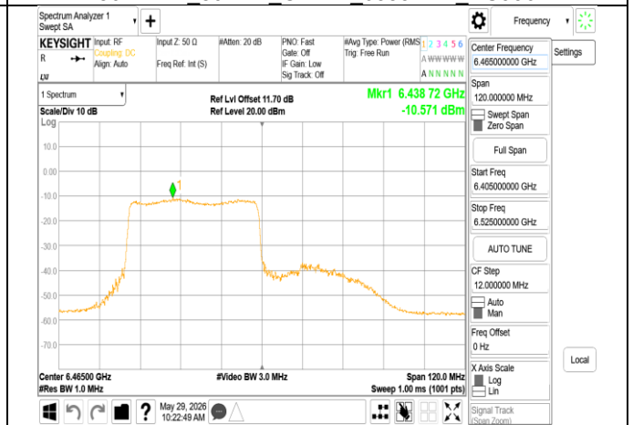
802.11ax 80MHz Chain1 6465MHz RU484 65
