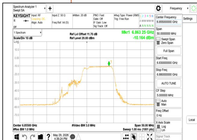
802.11be_20MHz_Chain0_6855MHz_106+26_MR02
