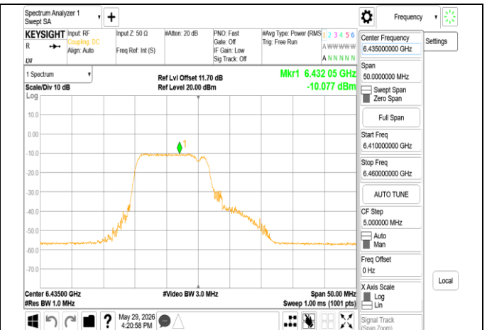
802.11be 20MHz Chain0 6435MHz 106+26 MRU1
