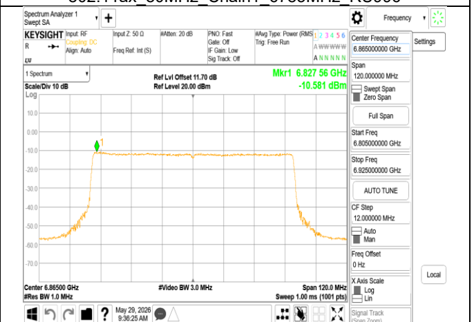
802.11ax 80MHz Chain1 6865MHz RU996
