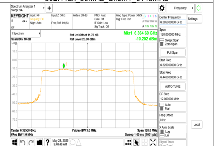
802.11ax_80MHz_Chain1_6385MHz
