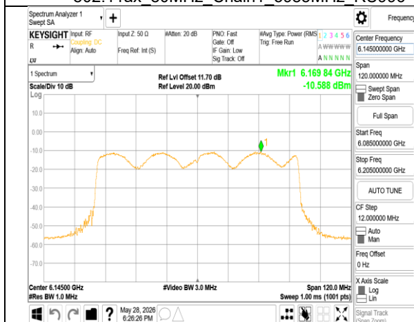
802.11ax_80MHz_Chain1_6145MHz_RU996
