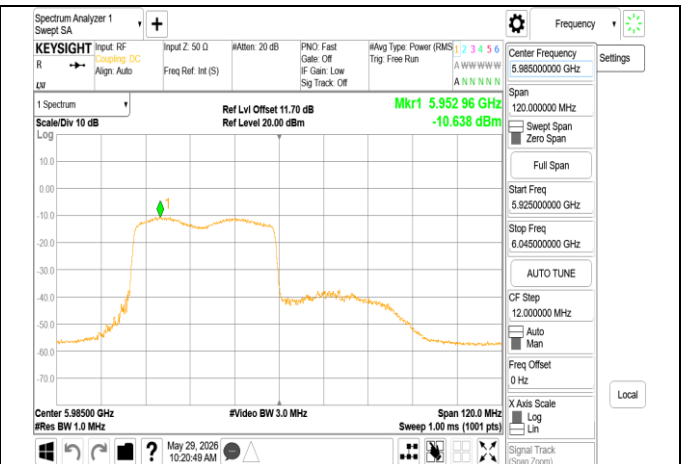
802.11ax_80MHz_Chain1_5985MHz_RU484_65
