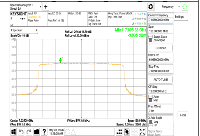
802.11ax 80MHz Chain1 7025MHz
