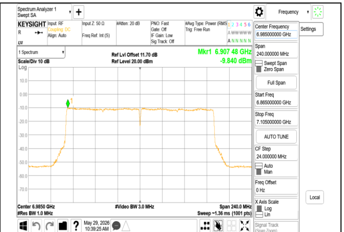
802.11ax_160MHz_Chain0_6985MHz_RU996x2
