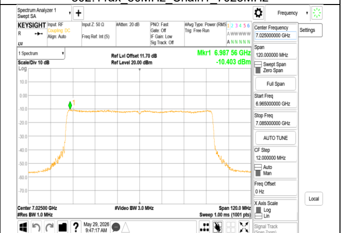
802.11ax 80MHz Chain1 7025MHz RU996
