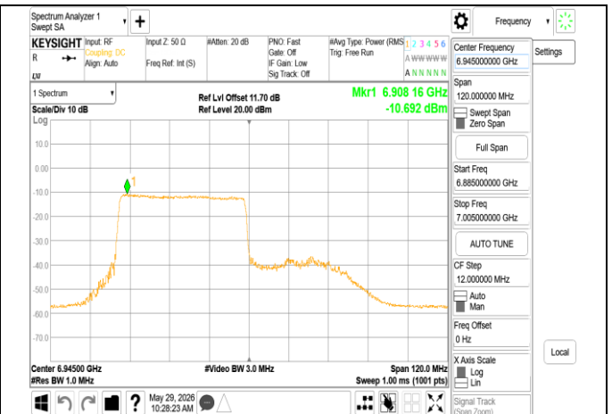
802.11ax 80MHz Chain1 6945MHz RU484 65
