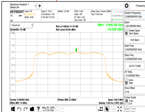
802.11ax_80MHz_Chain1_5985MHz
