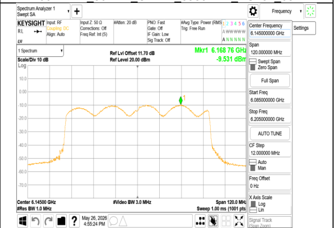
802.11ax_80MHz_Chain1_6145MHz
