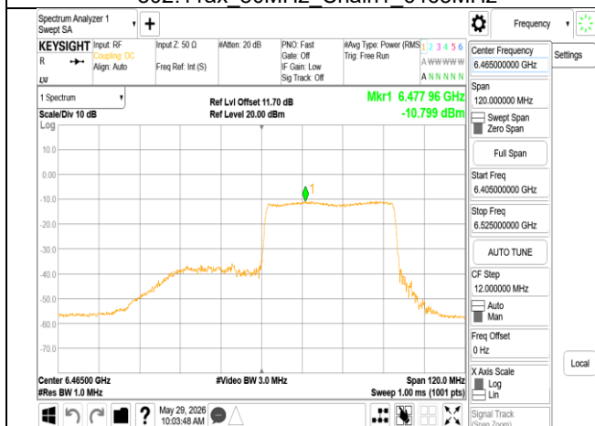
802.11ax 80MHz Chain1 6465MHz RU484 66
