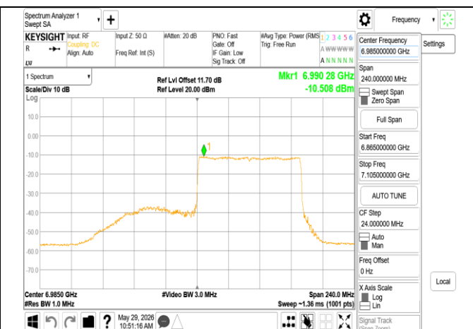
802.11ax 160MHz Chain1 6985MHz RU996 S67
