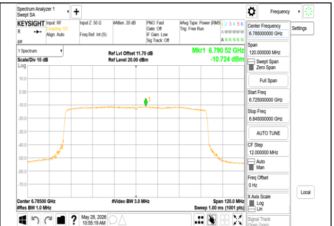
802.11ax 80MHz Chain1 6785MHz
