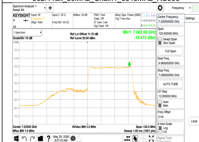
802.11ax 80MHz Chain1 7025MHz RU484 66
