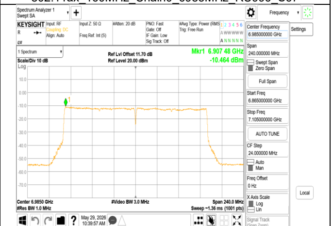
802.11ax_160MHz_Chain1_6985MHz_RU996x2
