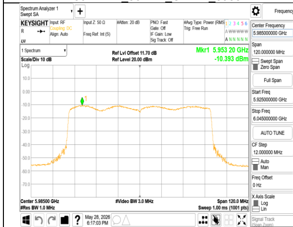
802.11ax_80MHz_Chain1_5985MHz_RU996
