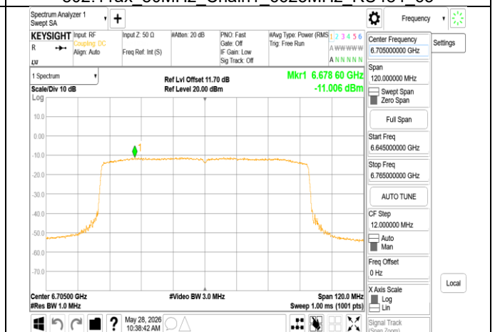
802.11ax 80MHz Chain1_6705MHz
