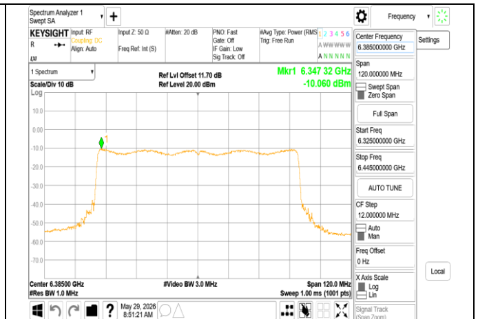
802.11ax 80MHz Chain1 6385MHz RU996
