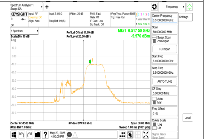
802.11be 20MHz Chain0 6515MHz 52+26 MRU3
