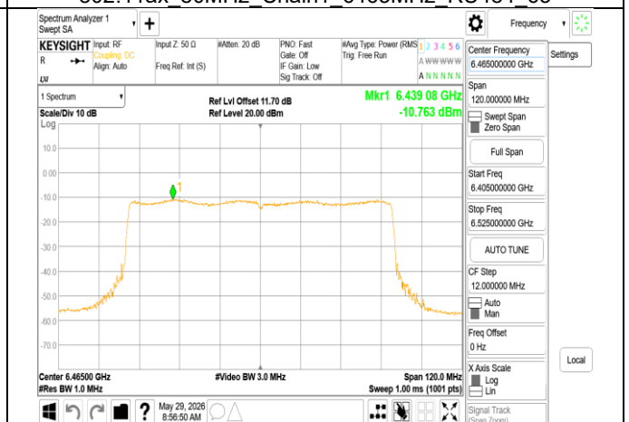
802.11ax 80MHz Chain1 6465MHz RU996
