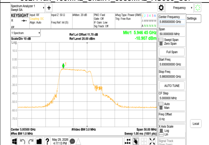
802.11be 20MHz Chain0 5955MHz 106+26 MRU1
