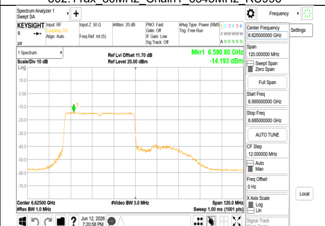
802.11ax 80MHz Chain1 6625MHz RU484 65
