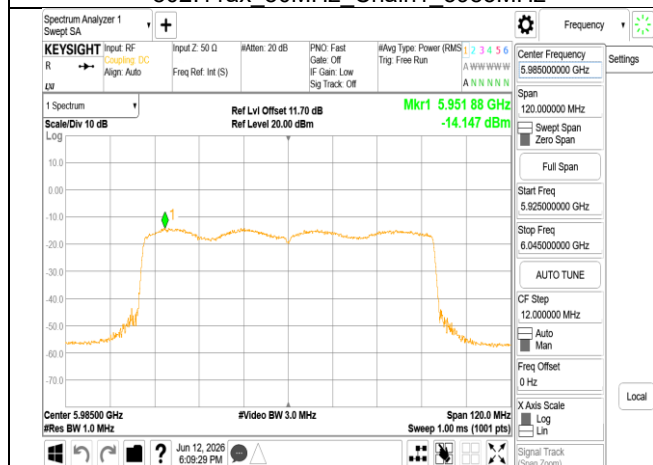
802.11ax_80MHz_Chain1_5985MHz_RU996
