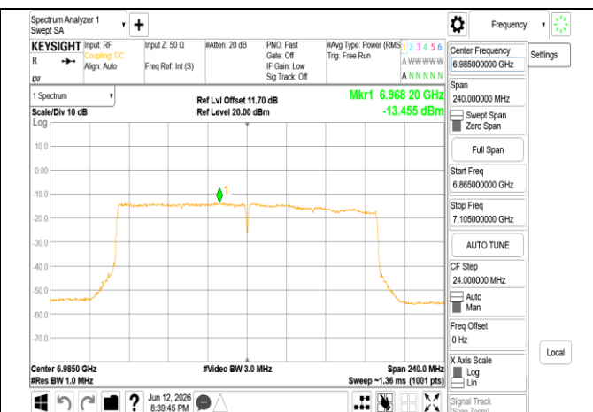
802.11ax_160MHz_Chain0_6985MHz_RU996x2
