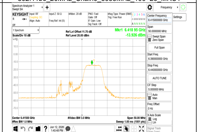
802.11be 20MHz Chain0 6415MHz 52+26 MRU3
