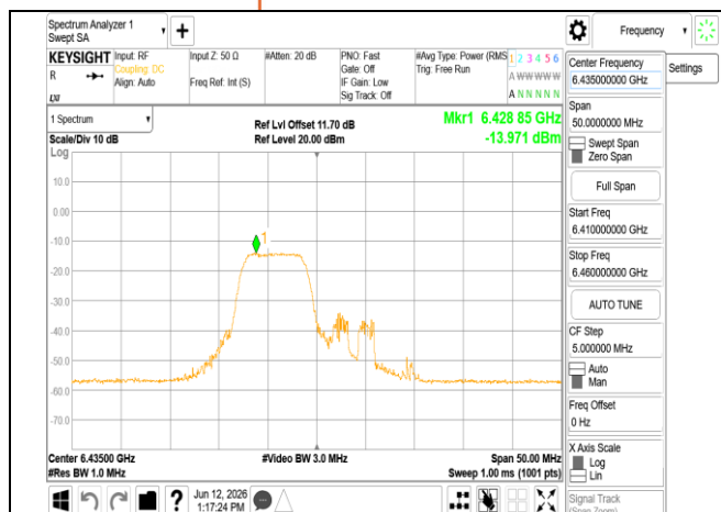
802.11be_20MHz_Chain0_6435MHz_52+26_MRUI
