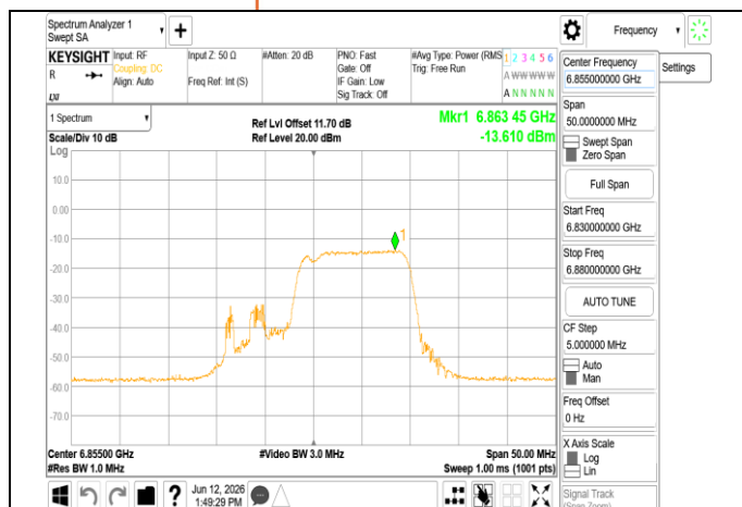
802.11be 20MHz Chain0 6855MHz 106+26 MRU2
