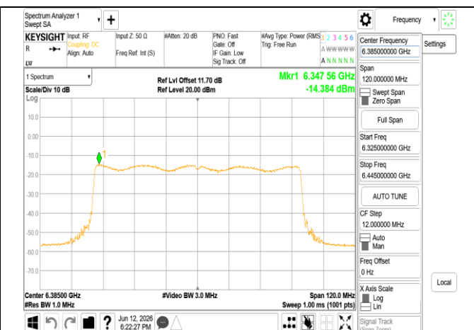
802.11ax 80MHz Chain1 6385MHz RU996
