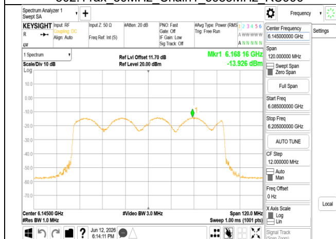
802.11ax_80MHz_Chain1_6145MHz_RU996
