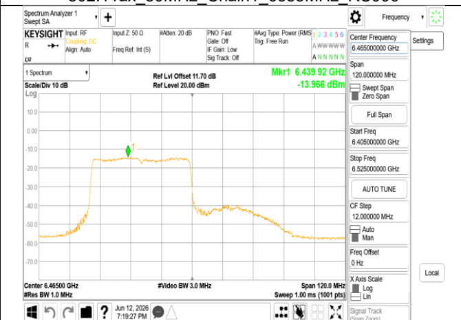
802.11ax 80MHz Chain1 6465MHz RU484 65
