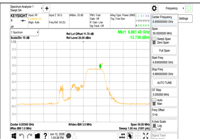
802.11be 20MHz Chain0 6855MHz 52+26 MRU3
