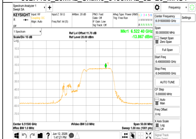
802.11be_20MHz_Chain0_6515MHz_106+26_MRUI
