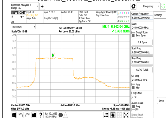
802.11ax_160MHz_Chain0_6985MHz_RU996_67
