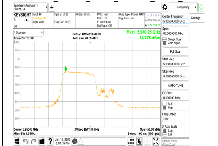
802.11be 20MHz Chain0 5955MHz 106+26 MRU1
