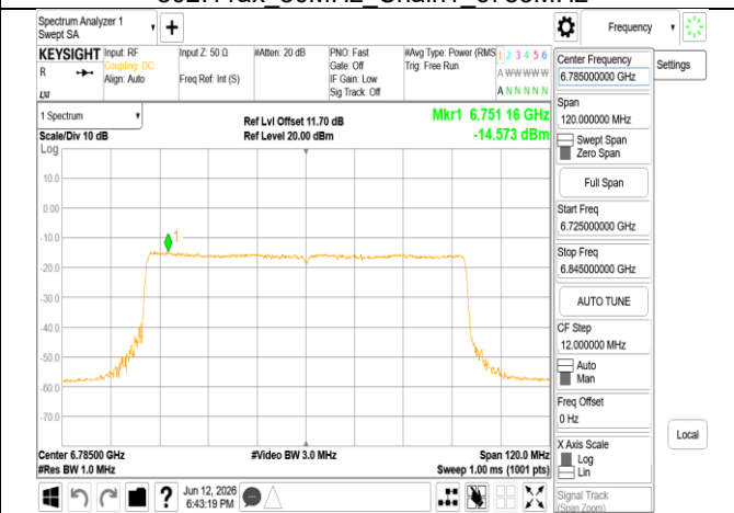
802.11ax 80MHz Chain1 6785MHz RU996
