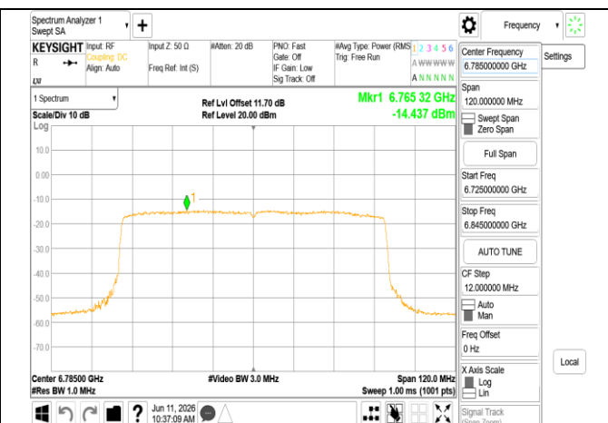
802.11ax 80MHz Chain1 6785MHz
