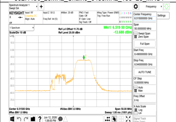
802.11be_20MHz_Chain0_6515MHz_52+26_MRUI
