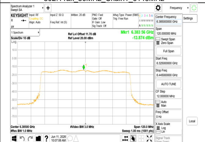
802.11ax_80MHz_Chain1_6385MHz
