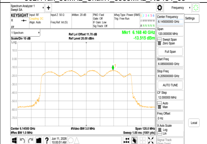
802.11ax_80MHz_Chain1_6145MHz
