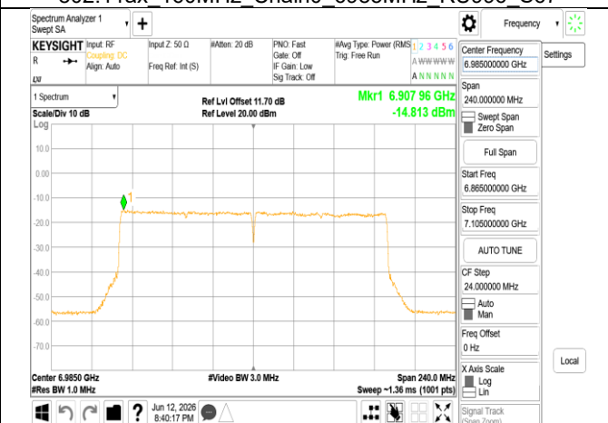
802.11ax_160MHz_Chain1_6985MHz_RU996x2
