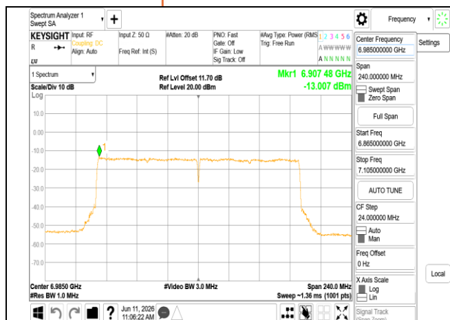
802.11ax_160MHz_Chain0_6985MHz
