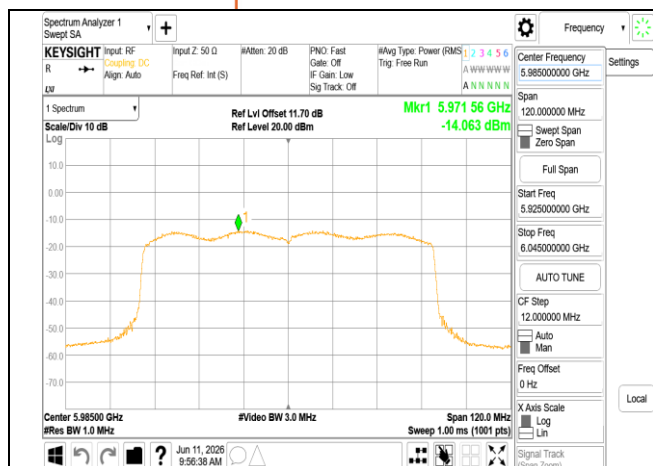
802.11ax_80MHz_Chain1_5985MHz
