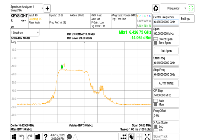
802.11be_20MHz_Chain0_6435MHz_106+26_MRUI
