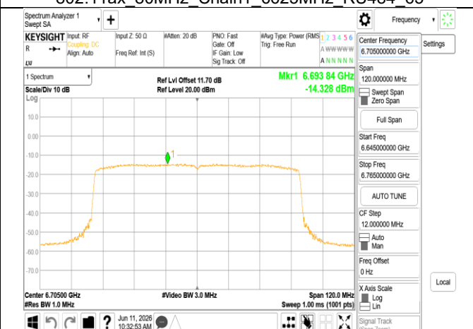
802.11ax 80MHz Chain1 6705MHz
