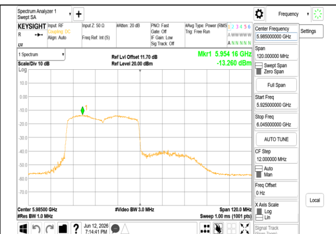
802.11ax_80MHz_Chain1_5985MHz_RU484_65
