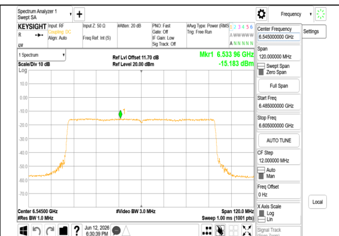
802.11ax 80MHz Chain1 6545MHz RU996
