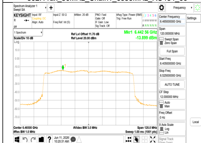
802.11ax 80MHz Chain1 6465MHz
