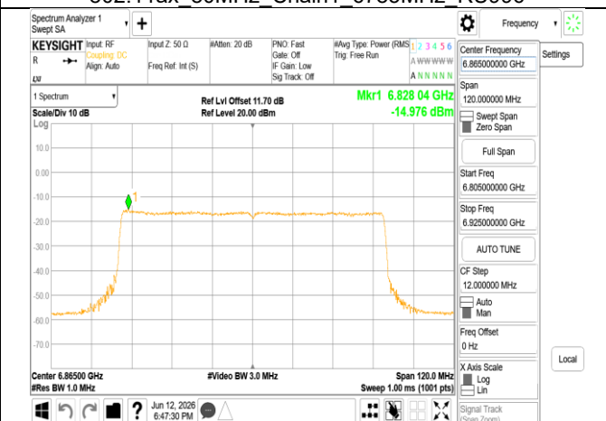
802.11ax 80MHz Chain1 6865MHz RU996
