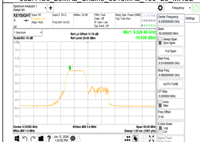
802.11be_20MHz_Chain0_6535MHz_52+26_MRUI
