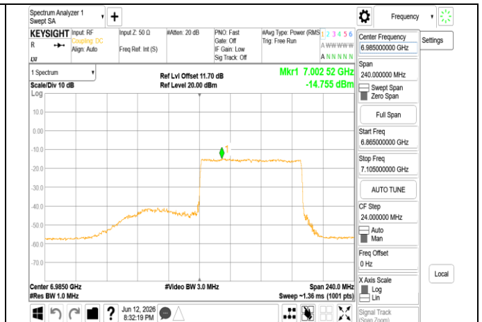
802.11ax 160MHz Chain1 6985MHz RU996 S67
