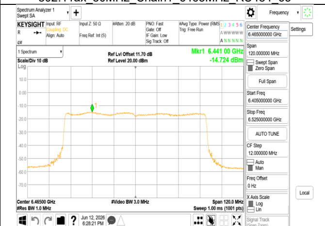
802.11ax 80MHz Chain1 6465MHz RU996
