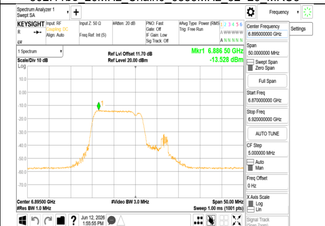
802.11be 20MHz Chain0 6895MHz 106+26 MRU1
