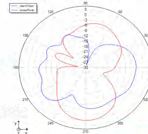
Theta=90 freq=2428MHz
