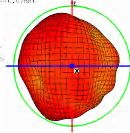
Theta=90 freq=2428MHz
