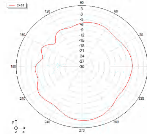
Theta=90 freq=2428MHz
