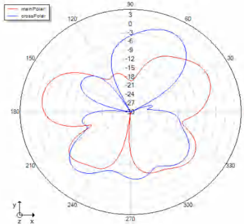
Theta=90 freq=2428MHz
