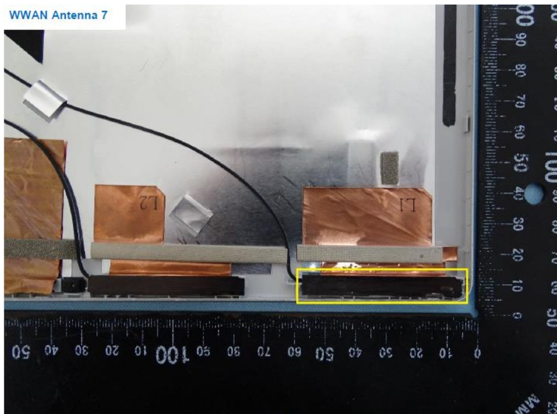
WWAN Antenna 8
