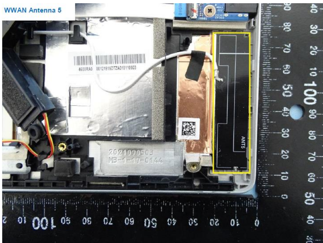
WWAN Antenna 6
