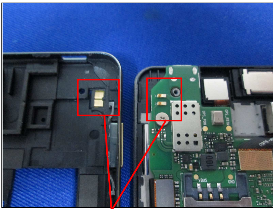
BT/WIFI ANT
