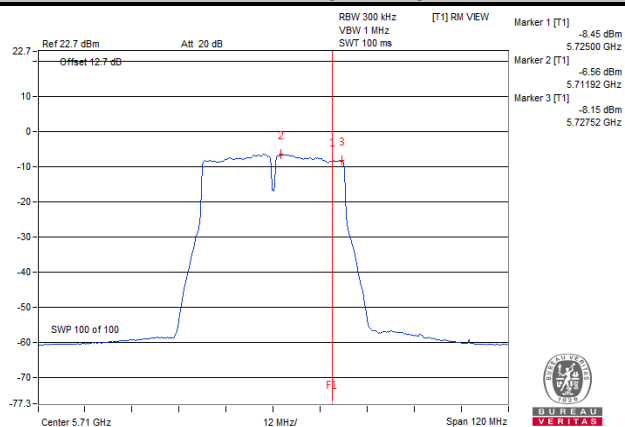
802.11ac (VHT40)
