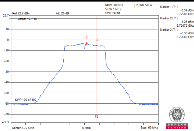
802.11ac (VHT40)
