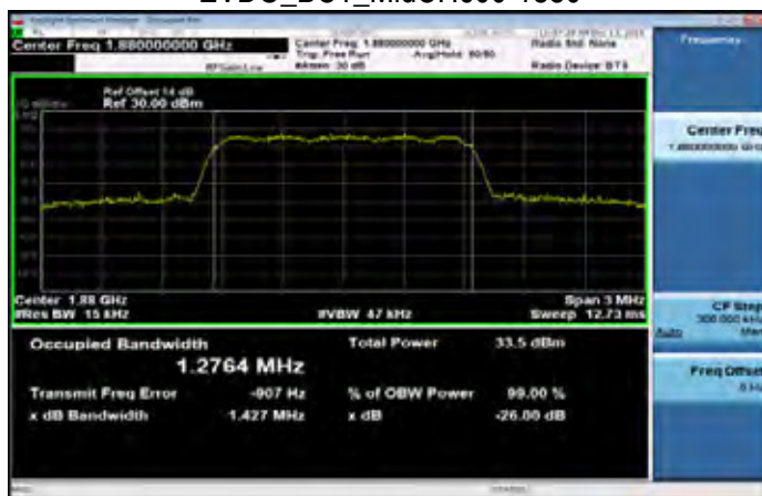
EVDO_BC1_MidCH600-1880
