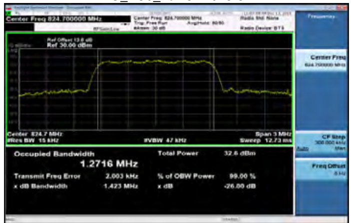
EVDO_BC0_LowCH1013-824.7
