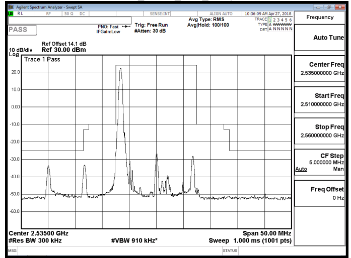
Band 7_QPSK_15M_RB1,74
