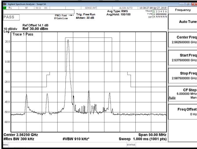
Band 7_QPSK_15M_RB1,74
