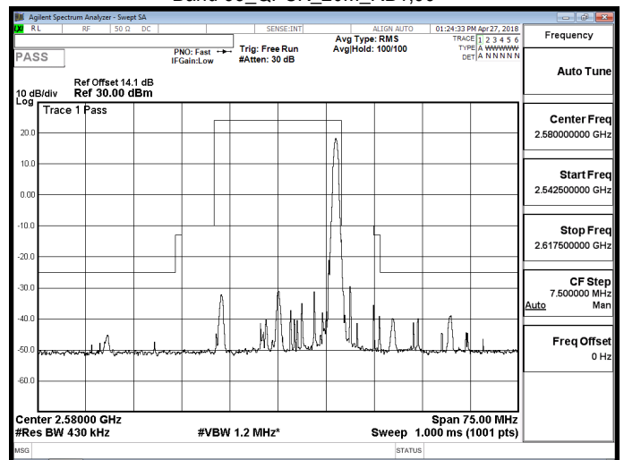
Band 38_QPSK_20M_RB1,99
