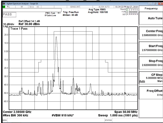
Band 38_QPSK_15M_RB1,74
