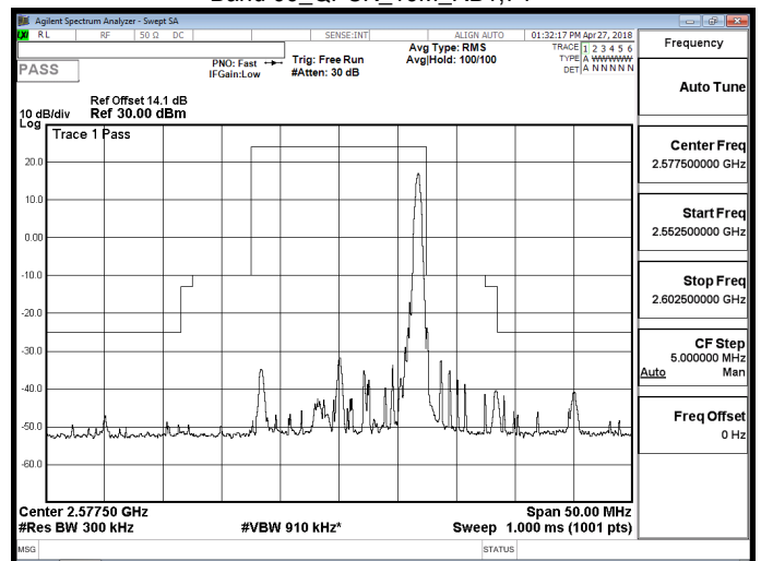
Band 38_QPSK_15M_RB1,74
