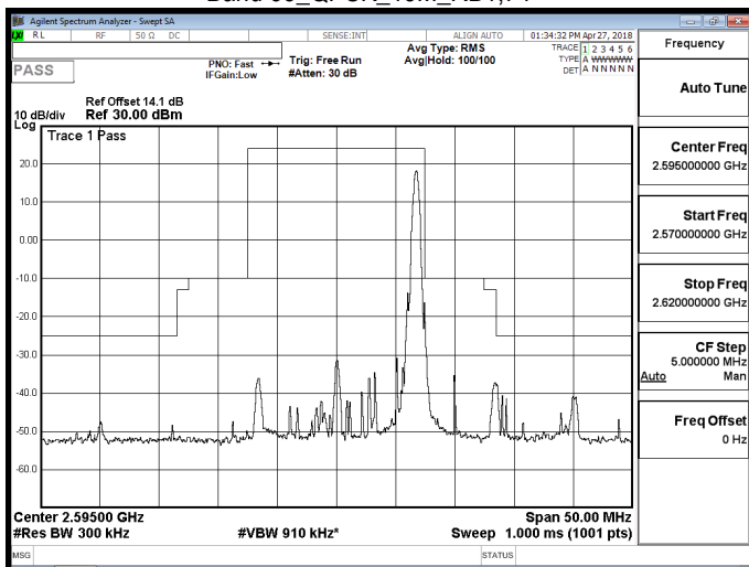
Band 38_QPSK_15M_RB1,74
