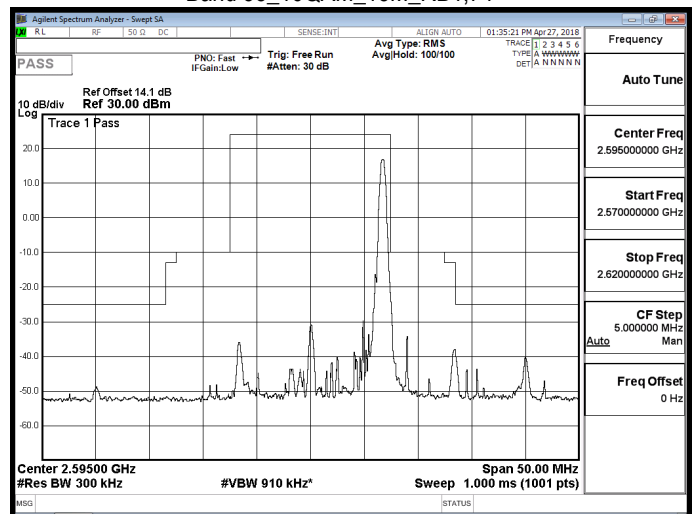
Band 38_16QAM_15M_RB1,74
