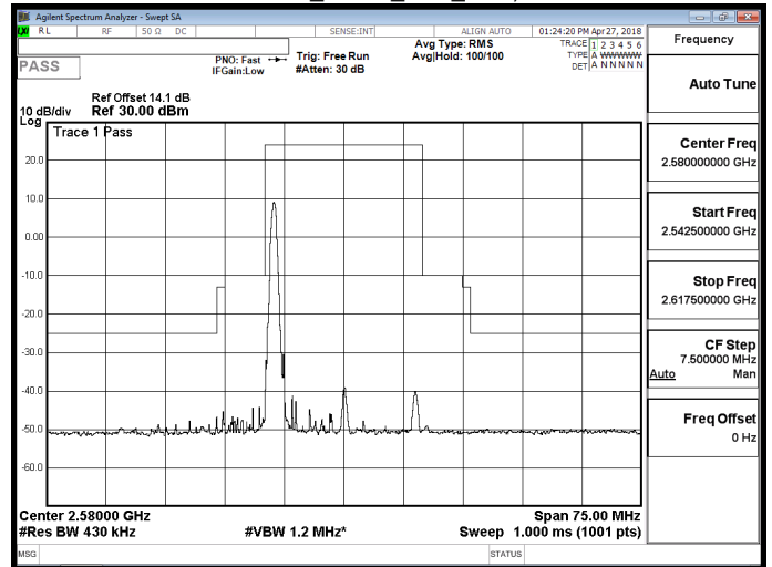
Band 38_QPSK_20M_RB1,99
