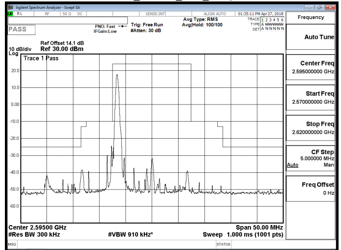
Band 38_16QAM_15M_RB1,74
