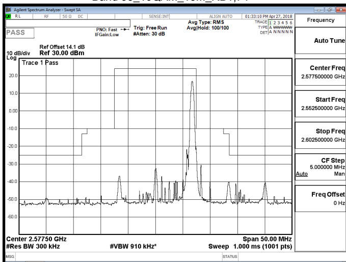
Band 38_16QAM_15M_RB1,74
