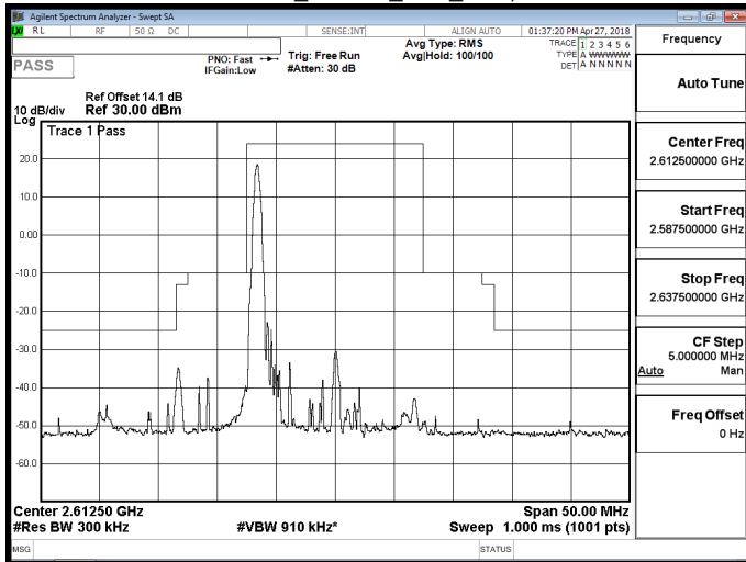
Band 38_16QAM_15M_RB1,74
