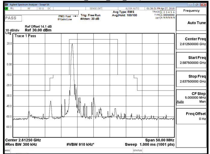
Band 38_QPSK_15M_RB1,74
