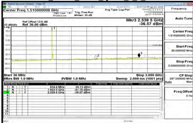
30MHz~3GHz Band5 5MHz QPSK 1 0 MidCH20525
