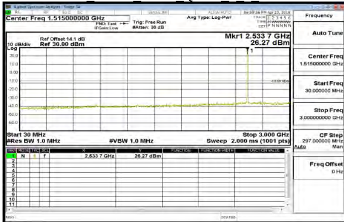
30MHz~3GHz Band7 5MHz QPSK 1 0 MidCH21100
