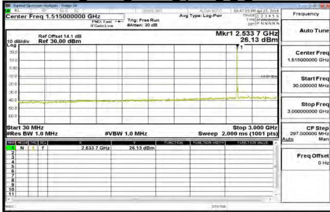
30MHz~3GHz Band7 10MHz QPSK 1 0 MidCH21100
