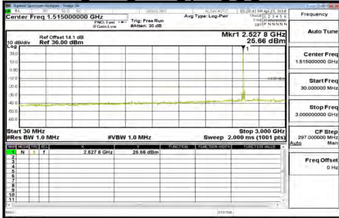
30MHz~3GHz Band7 20MHz QPSK 1 0 MidCH21100
