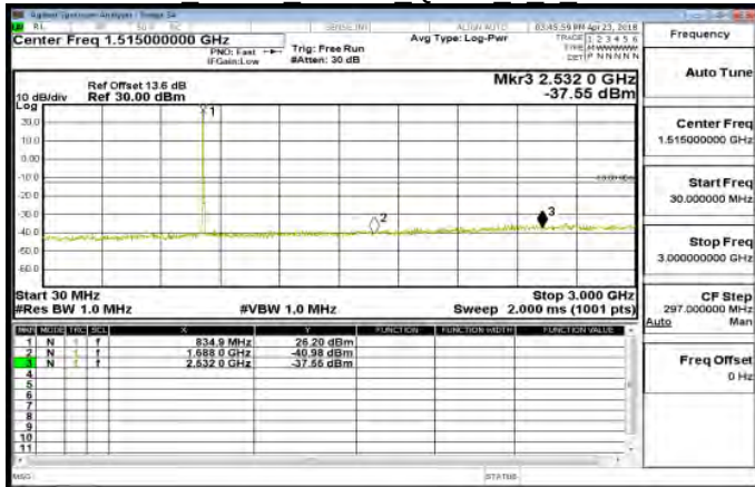
30MHz~3GHz Band5 10MHz QPSK 1 0 MidCH20525
