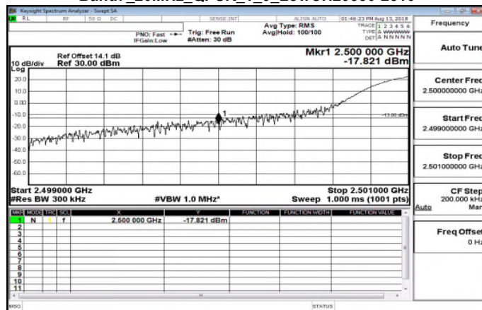
Band7_20MHz_QPSK_1_0_LowCH20850-2510
