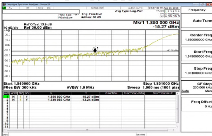
Band25 20MHz QPSK 1 0 LowCH26140
