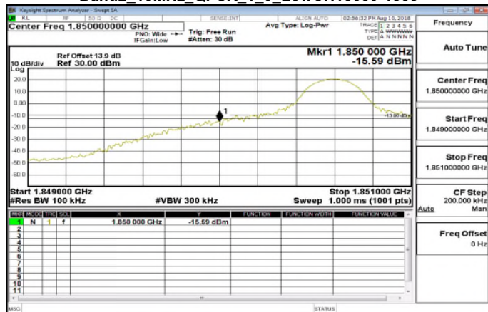
Band2 10MHz QPSK 1 0 LowCH18650-1855
