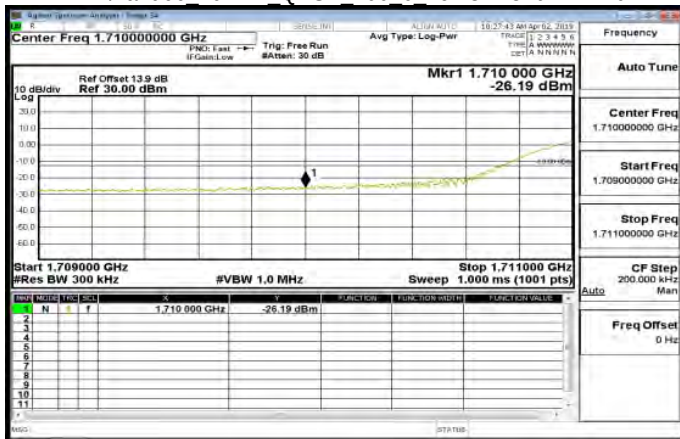
LTE\Band66 20MHz QPSK 100 0 LowCH132072-1720
