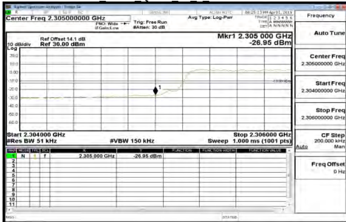
LTE\Band30 5MHz QPSK 25 0 LowCH27685-2307.5
