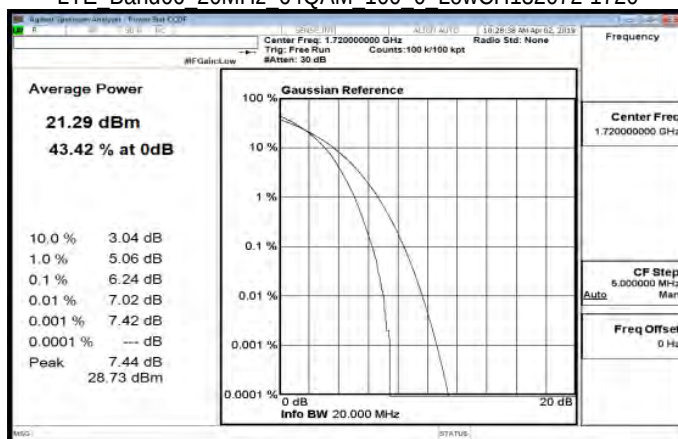
LTE Band66 20MHz 64QAM 100 0 LowCH132072-1720
