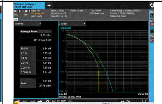
20MHz / 64QAM
