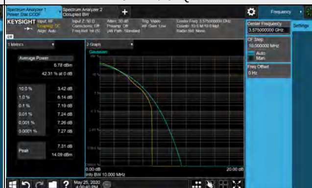
20MHz / 64QAM
