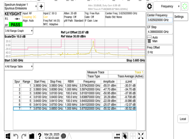
Band48_30MHz_DFT_s_OFDM_SCS30kHz_BPSK_RB1_77_CH641668
