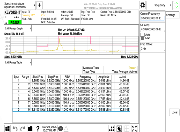
Band48_30MHz_CP_OFDM_SCS30kHz_QPSK_RB78_0_CH637668
