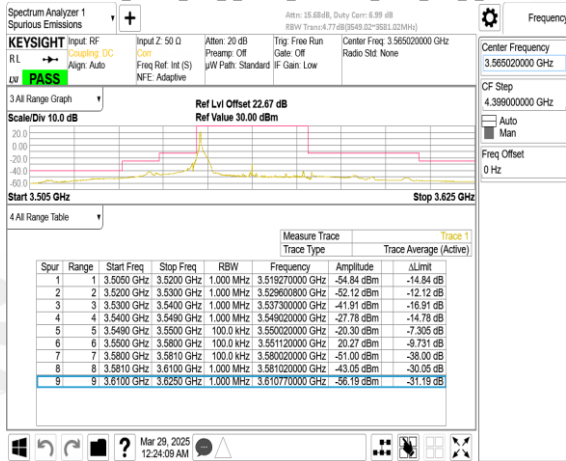
Band48_30MHz_DFT_s_OFDM_SCS30kHz_BPSK_RB1_77_CH637668
