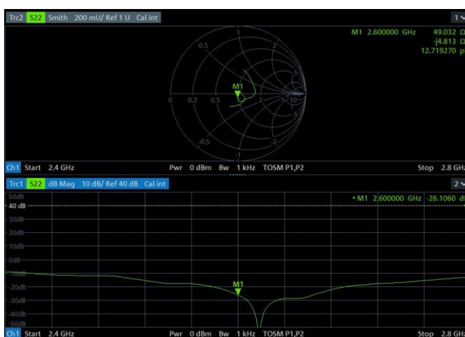
D2600V2_1005
