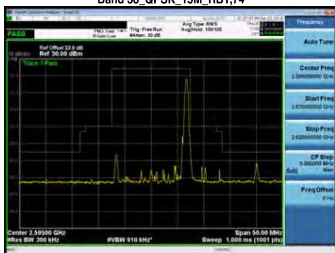
Band 38_QPSK_15M_RB1,74
