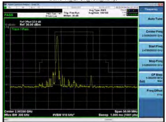
Band 41_QPSK_15M_RB1,74
