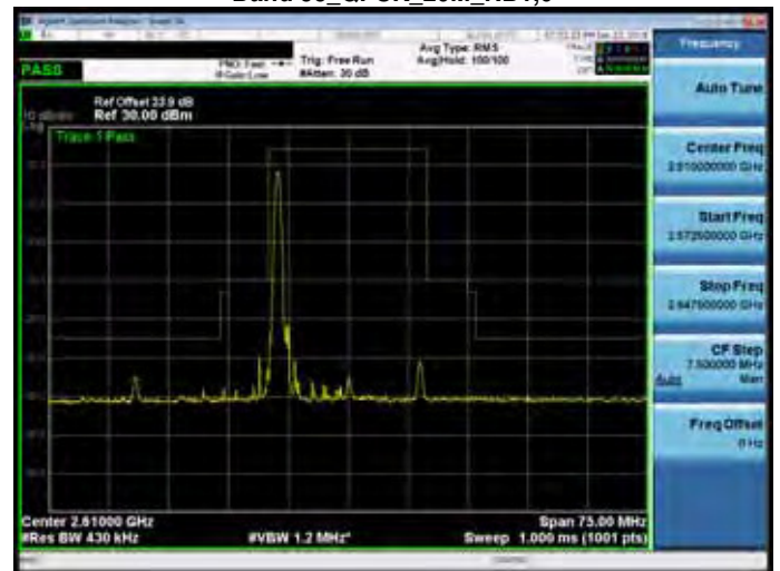
Band 38_QPSK_20M_RB1,99
