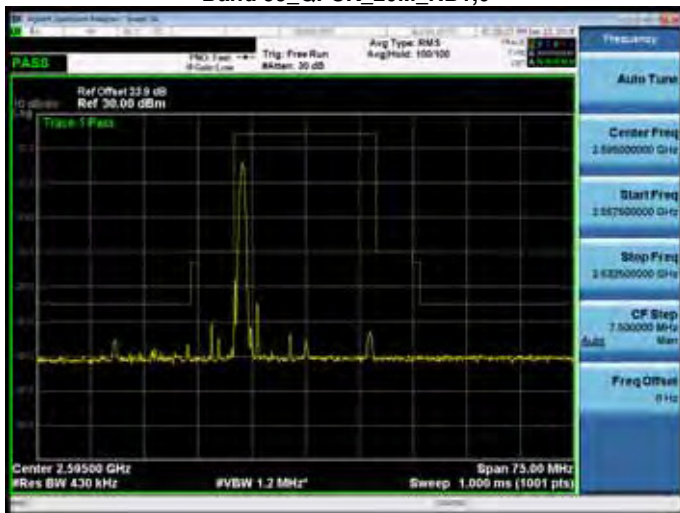
Band 38_QPSK_20M_RB1,99
