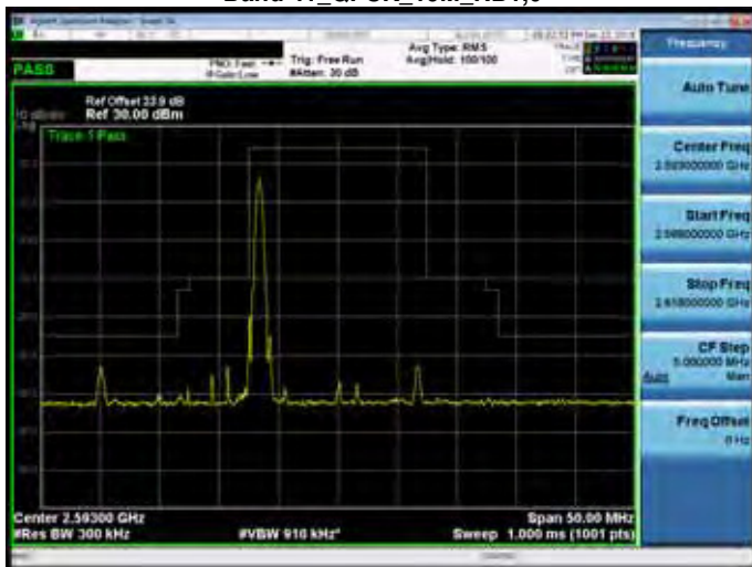
Band 41_QPSK_15M_RB1,74
