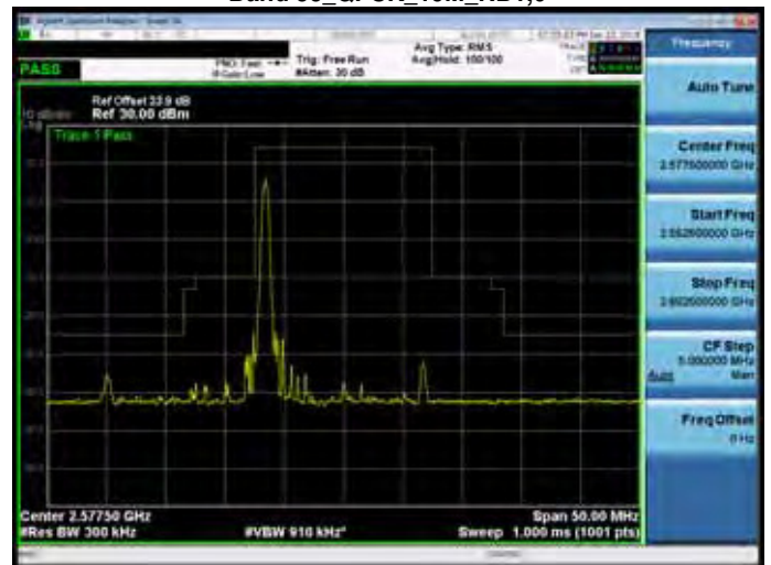
Band 38_QPSK_15M_RB1,74
