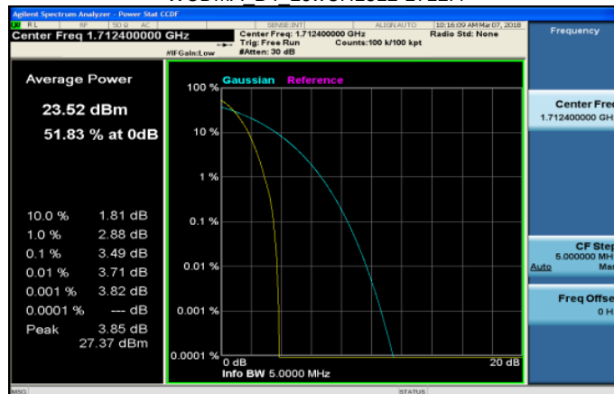
WCDMA_B4_LowCH1312-1712.4
