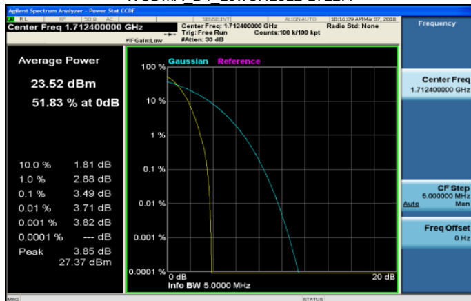
WCDMA_B4_LowCH1312-1712.4
