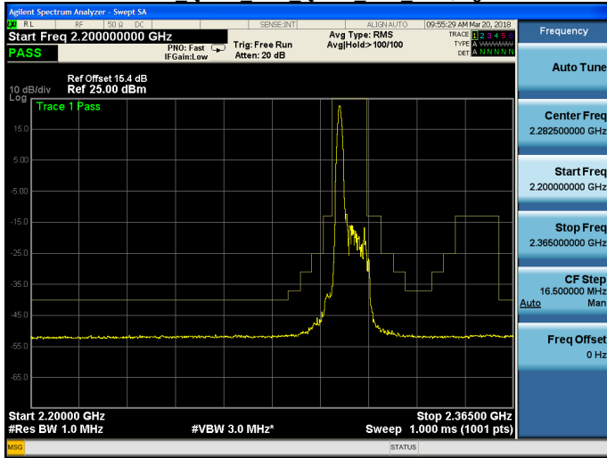
Band 30 QPSK 10M QPSK MID RB1,49.gif
