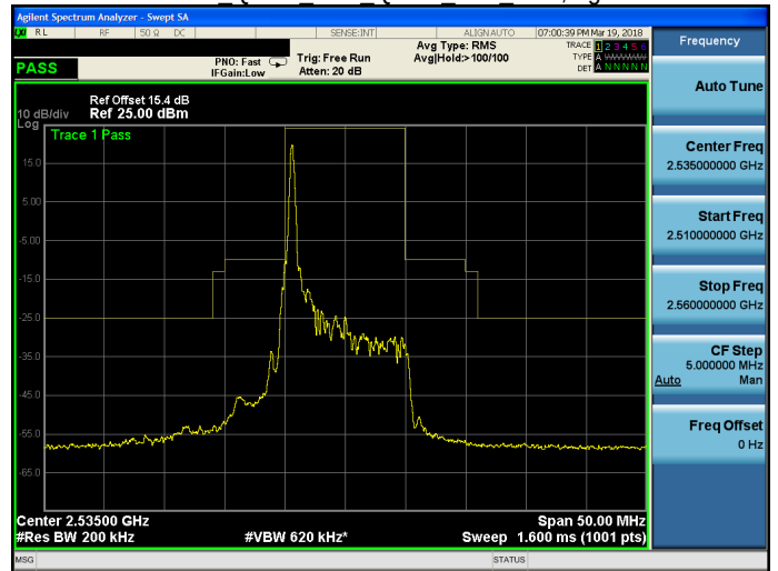
Band 7 QPSK 10M QPSK MID RB1,49.gif
