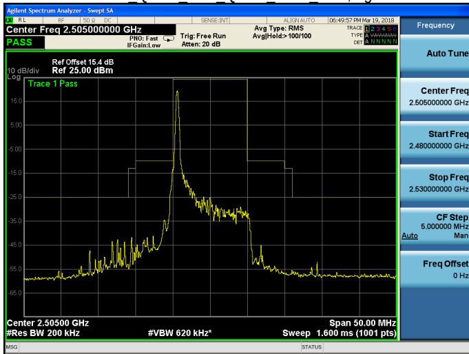
Band 7 QPSK 10M QPSK LOW RB1,49.gif
