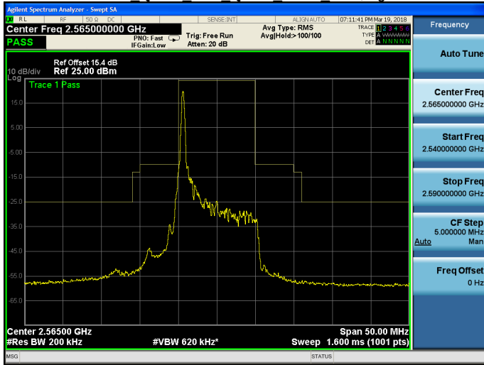
Band 7 QPSK 10M QPSK HIGH RB1,49.gif
