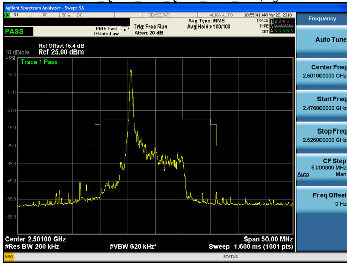
Band 41 QPSK 10M QPSK LOW RB1,49.gif
