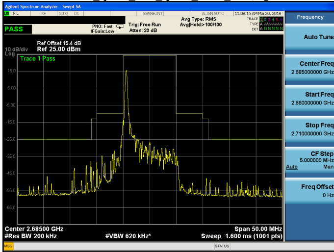
Band 41 QPSK 10M QPSK HIGH RB1,49.gif
