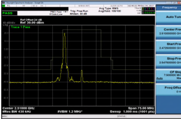
Band 7_20M_QPSK_LOW_RB1,99
