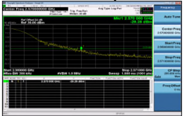
Band7_20MHz_QPSK_1_99_HighCH21350-2560
