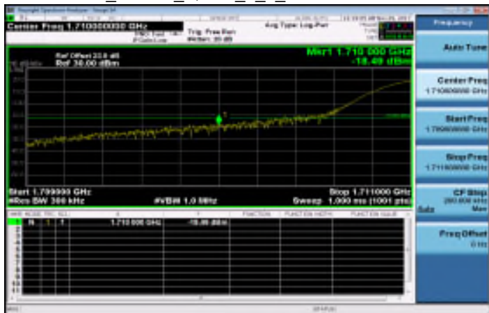
Band4_20MHz_QPSK_1_0_LowCH20050-1720
