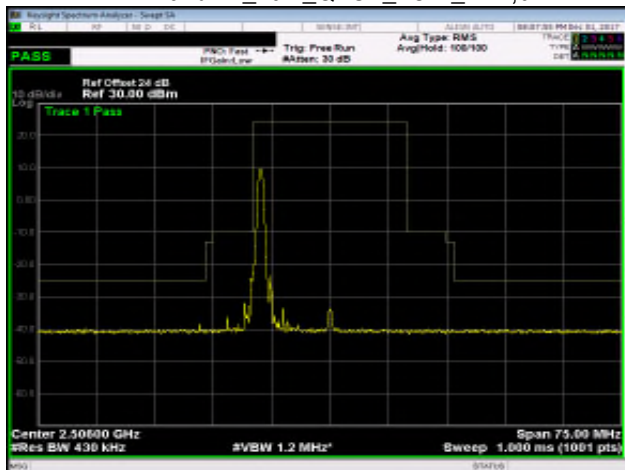
Band 41_20M_QPSK_LOW_RB1,99
