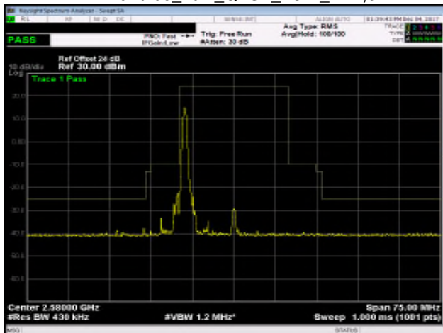
Band 38_20M_QPSK_LOW_RB1,99
