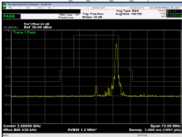
Band 38_20M_QPSK_LOW_RB100,0
