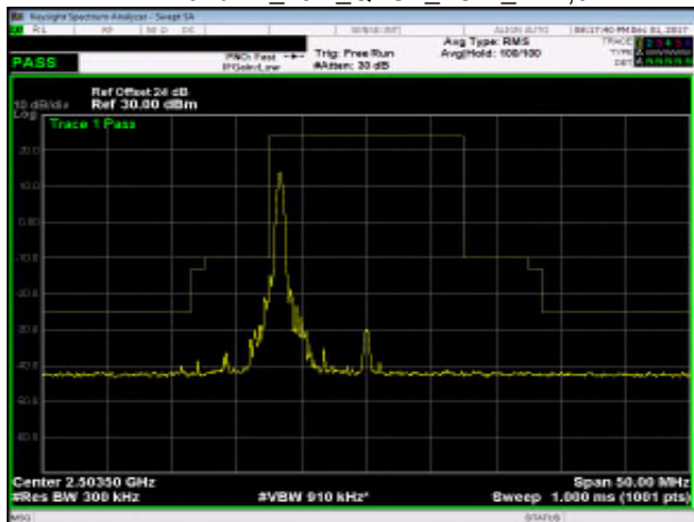
Band 41_15M_QPSK_LOW_RB1,74
