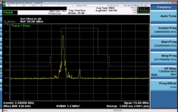
Band 38_20M_16QAM_LOW_RB1,99
