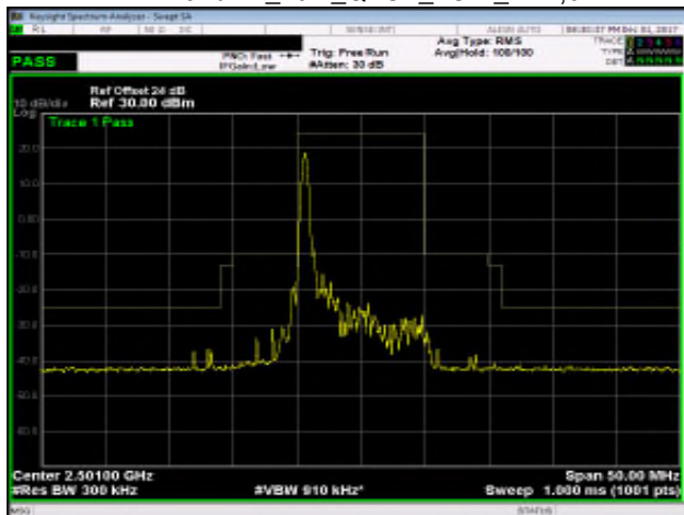
Band 41_10M_QPSK_LOW_RB1,49
