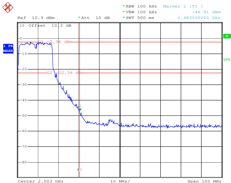
802.11g CH11
