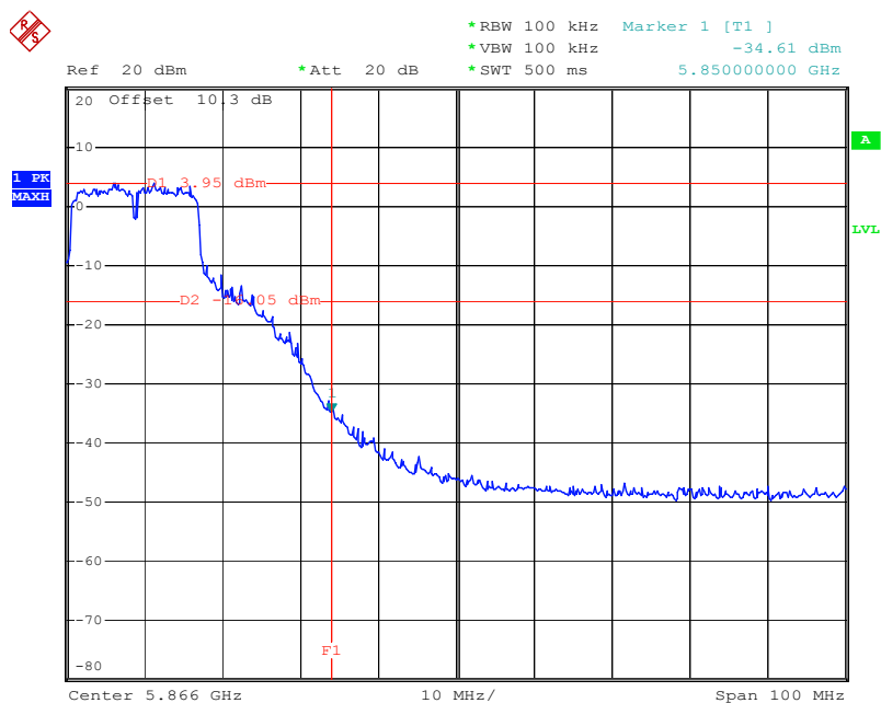
802.11a CH165
