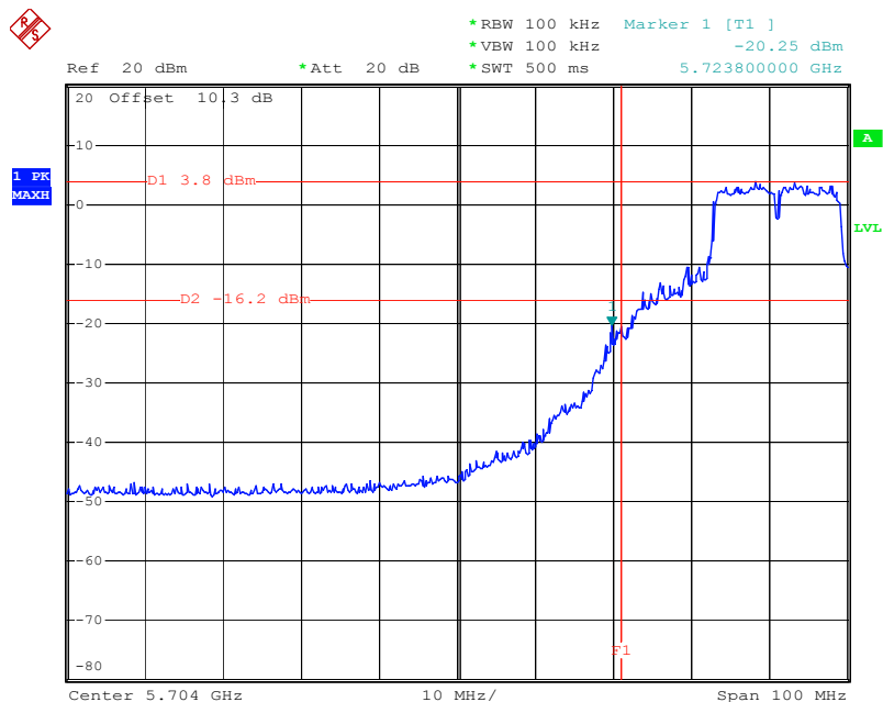
802.11a CH149
