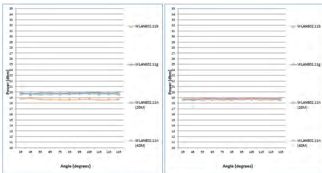
2.4GHz Main(SISO)
