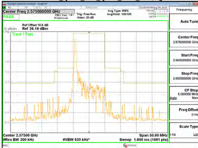
Band 38 QPSK 10M QPSK LOW RB1,49.gif
