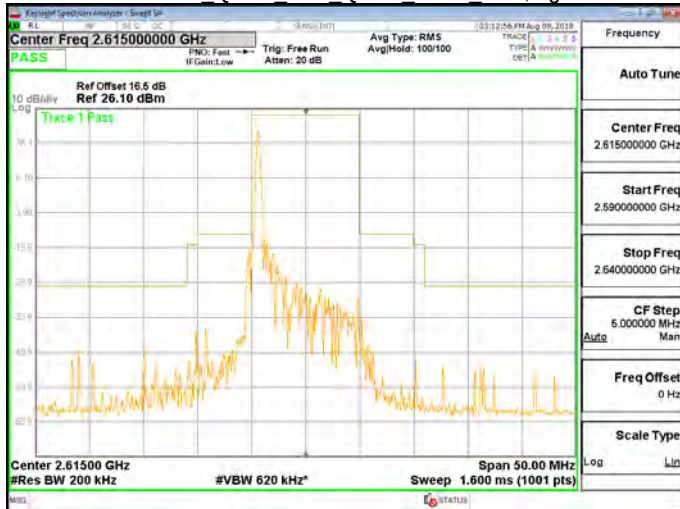
Band 38 QPSK 10M QPSK HIGH RB1,49.gif
