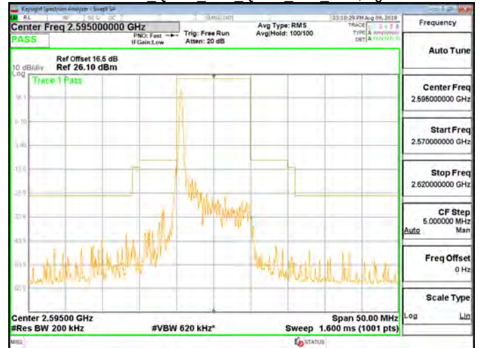
Band 38 QPSK 10M QPSK MID RB1,49.gif
