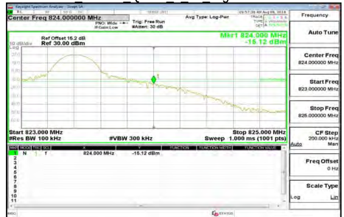
Band26 10MHz QPSK 50 0 LowCH26740-819
