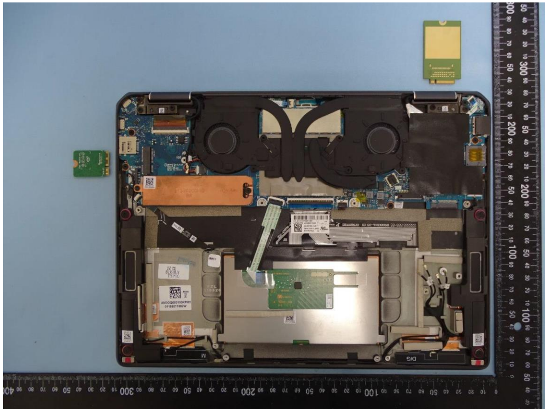
WLAN Module
