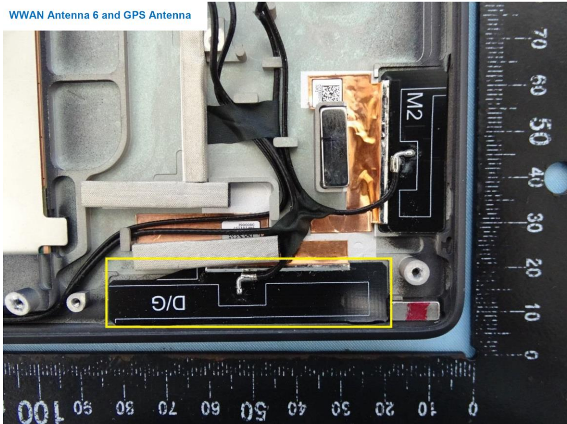
WWAN Antenna 7
