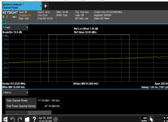
N26(5M)_DFT-s-OFDM_BPSK Edge_1RB_Left_Low_CH_CHP_PASS
