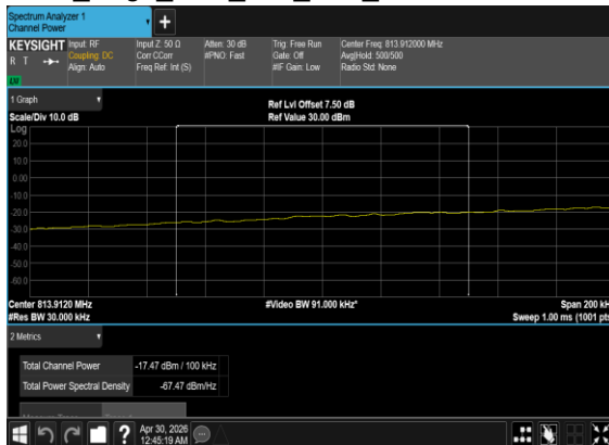
N26(5M)_DFT-s-OFDM_QPSK Edge_1RB_Left_Low_CH_CHP_PASS
