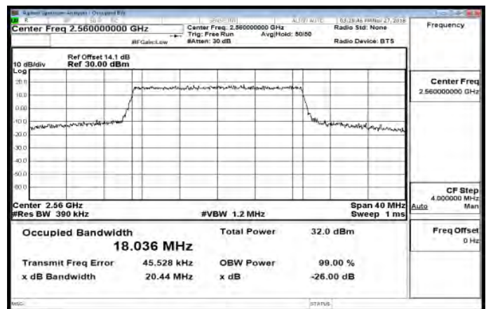
Band7_20MHz_QPSK_100_0_HighCH21350-2560
