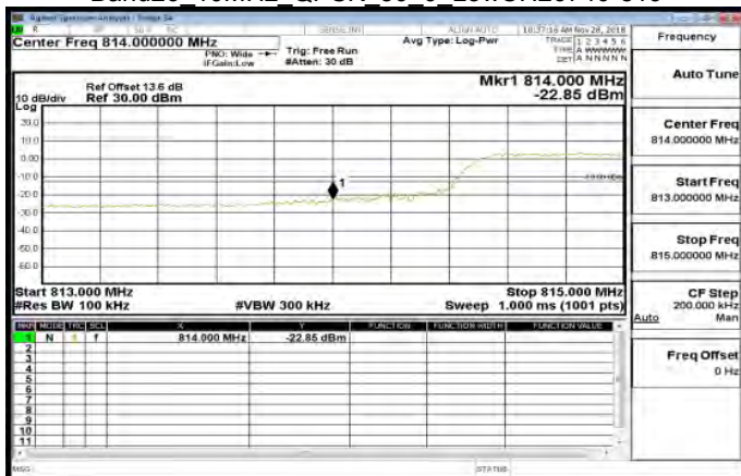
Band26 10MHz QPSK 50 0 LowCH26740-819
