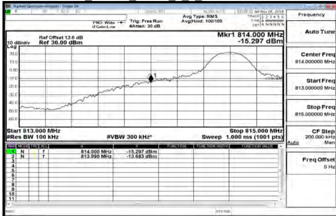
Band26 10MHz QPSK 1 0 LowCH26740-819
