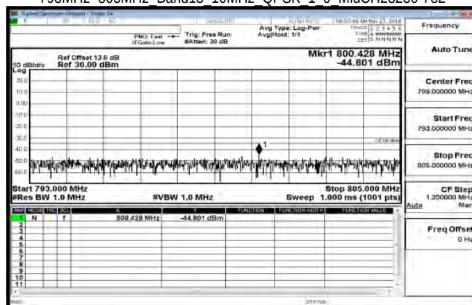
793MHz~805MHz Band13 10MHz QPSK 1 0 MidCH23230-782
