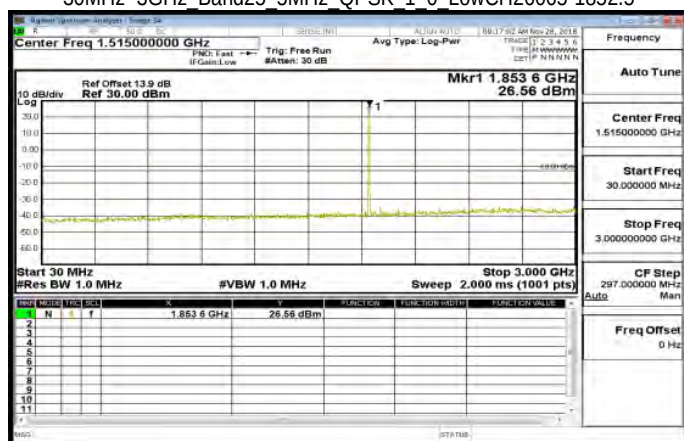
30MHz~3GHz Band25 5MHz QPSK 1 0 LowCH26065-1852.5
