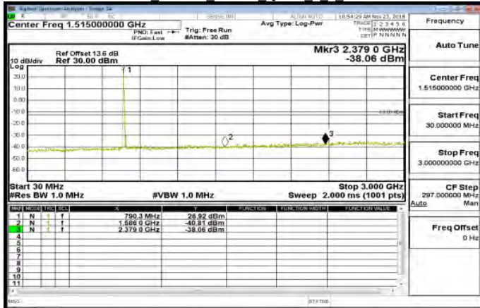
30MHz~3GHz Band14 10MHz QPSK 1 0 MidCH23330
