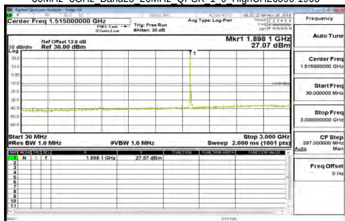
30MHz~3GHz Band25 20MHz QPSK 1 0 HighCH26590-1905
