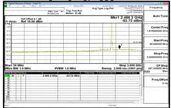
30MHz~3GHz Band30 5MHz QPSK 1 0 MidCH27710-2310
