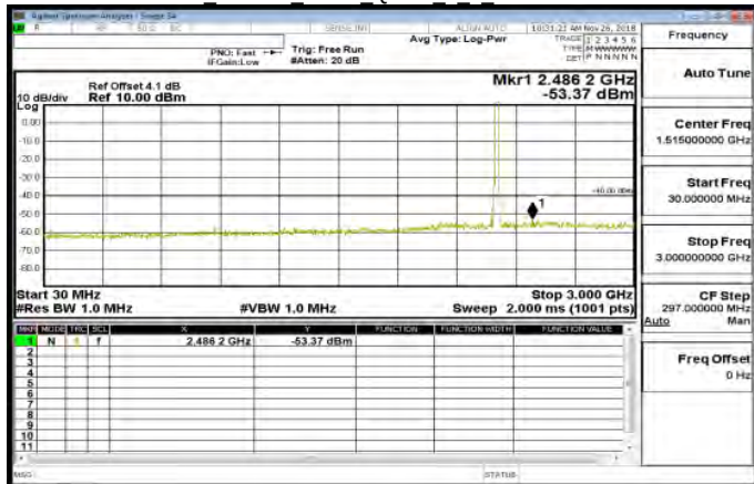
30MHz~3GHz Band30 5MHz QPSK 1 0 LowCH27685-2307.5
