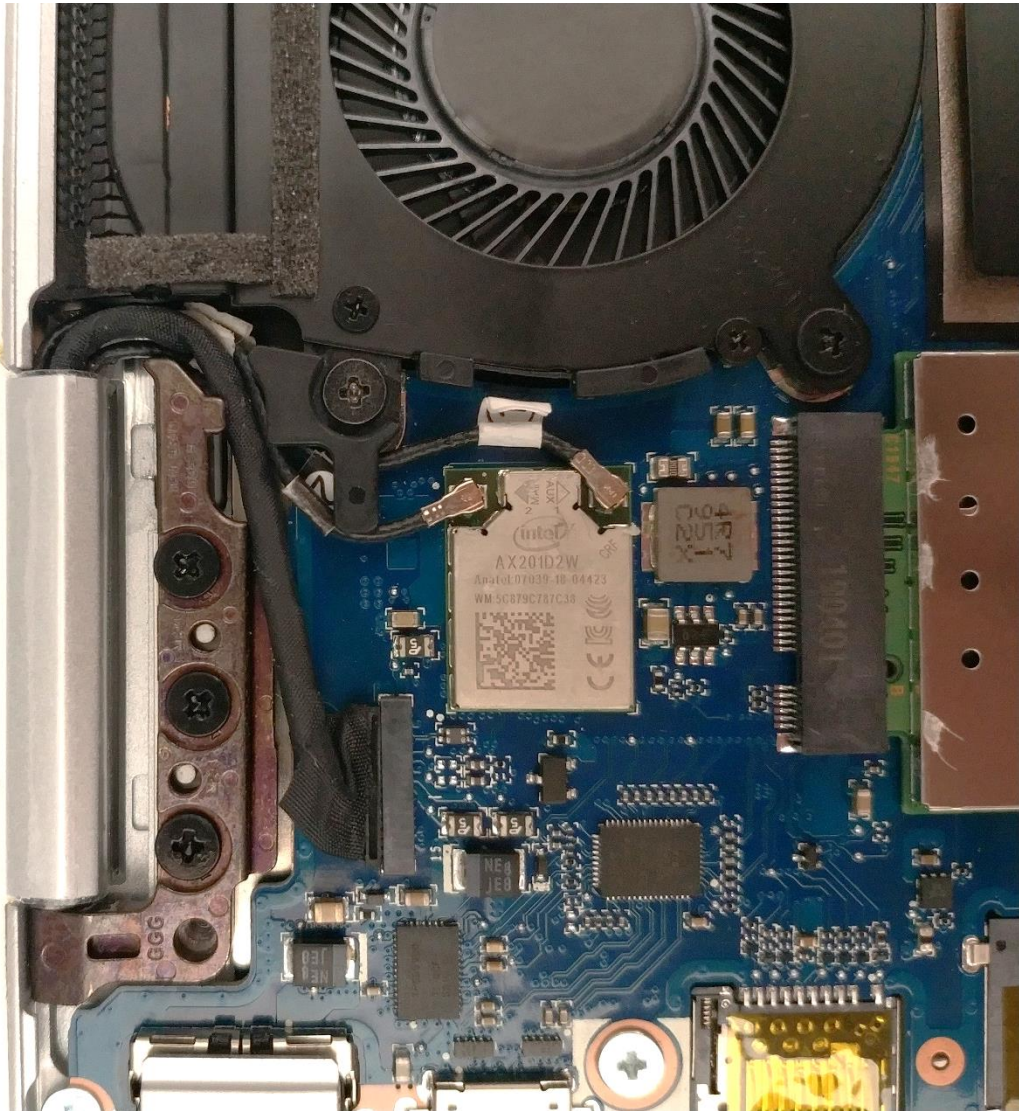
WLAN module:AX201D2W
