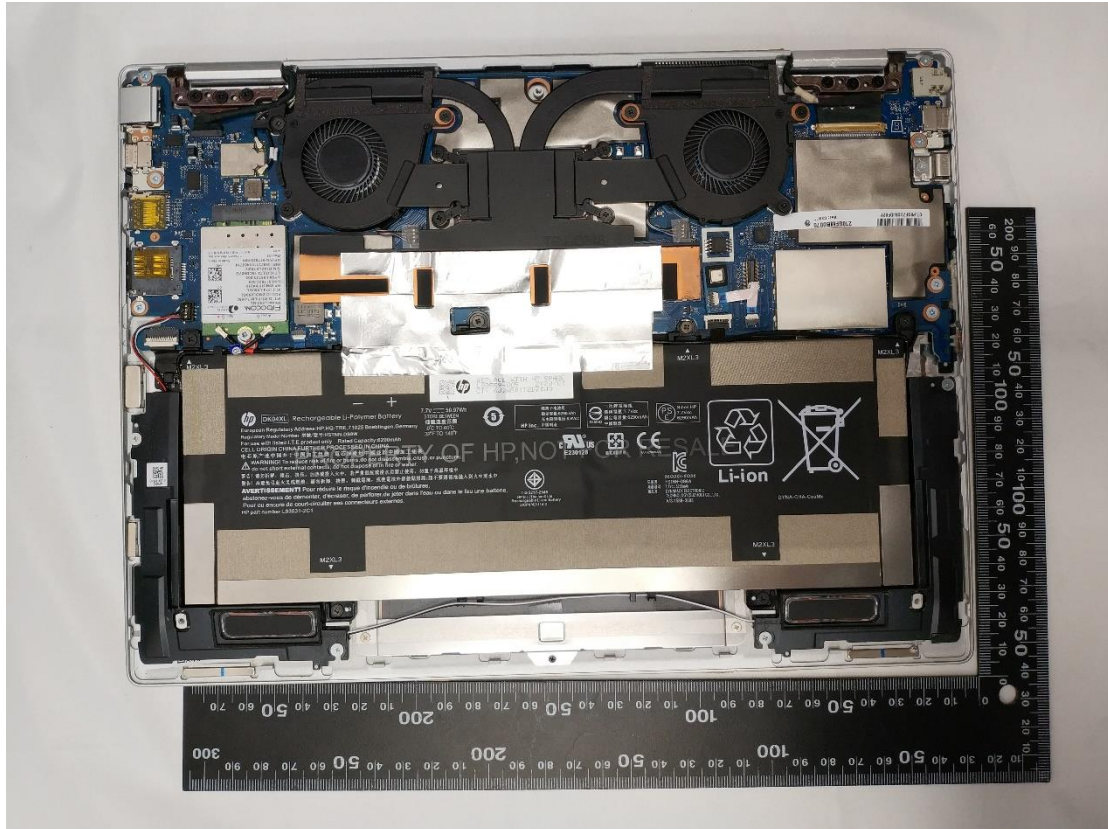
WWAN module:L850-GL
