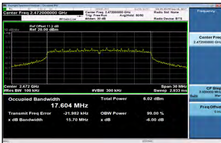
802.11n_20M (AUX1) CH-13
