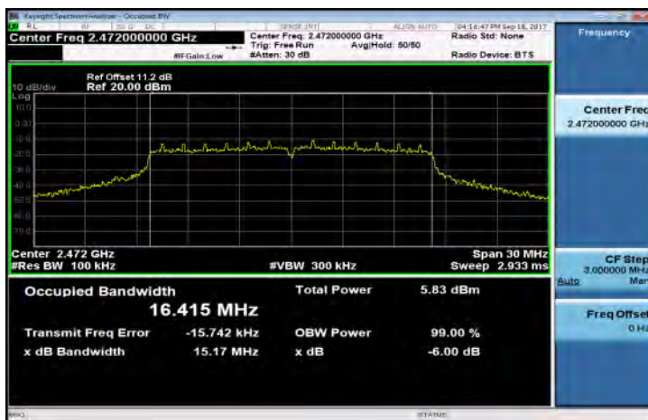
802.11g (AUX1) CH-13
