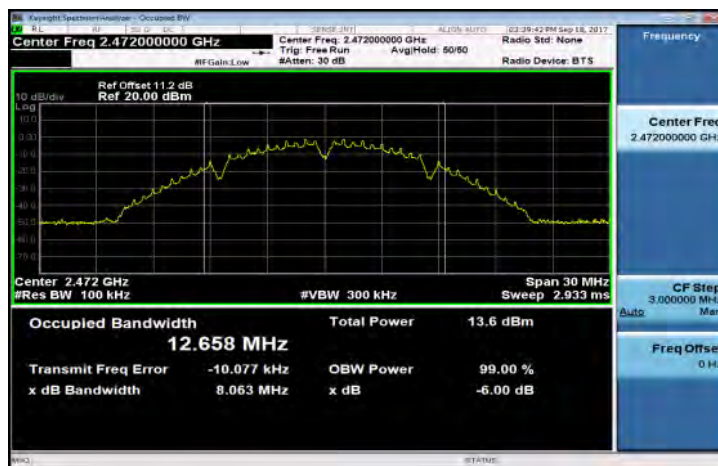
802.11b (AUX1) CH-13
