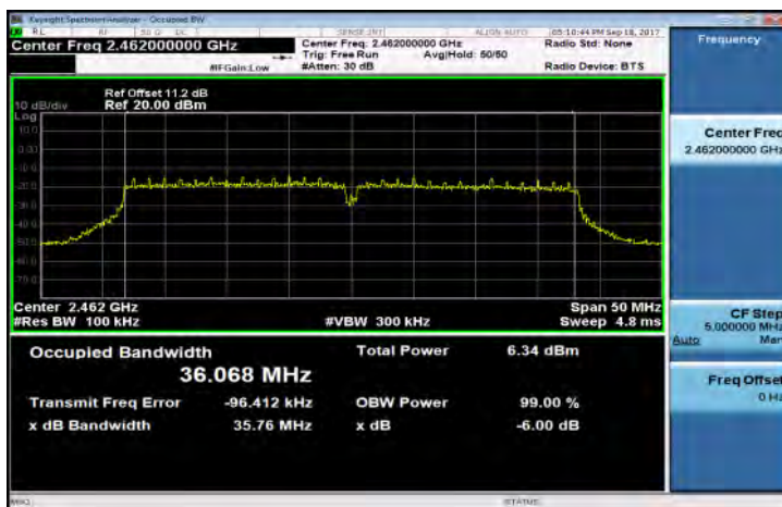
802.11n_40M (AUX1) CH-11
