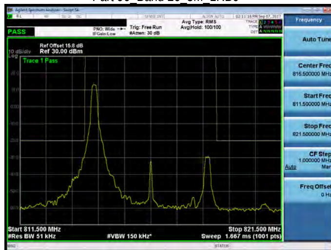
Part 90 Band 26 5M 1RB24
