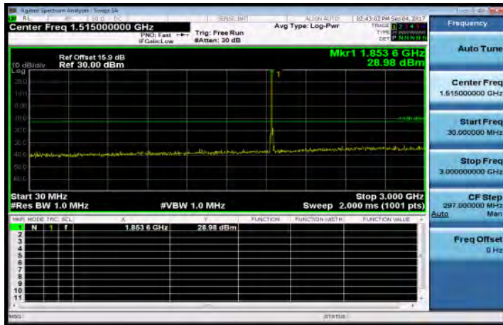
30MHz~3GHz_Band2_10MHz_QPSK_1_0_LowCH18650-1855
