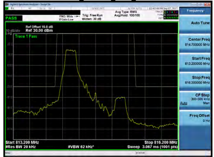
Part 90 Band 26 1.4M 1RB5
