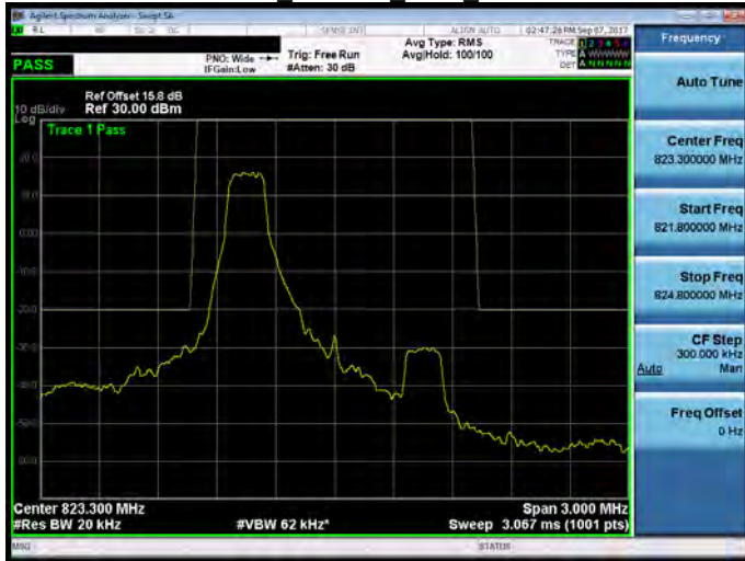
Part 90 Band 26 1.4M 1RB5
