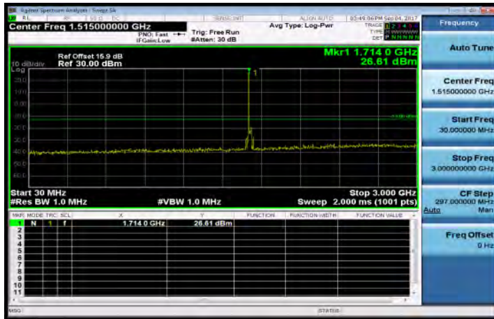
30MHz~3GHz_Band4_20MHz_QPSK_1_0_LowCH20050-1720
