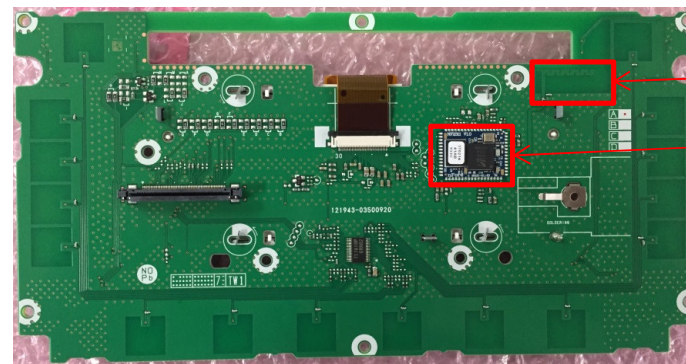
【PANEL_PCB(Solder side)】
