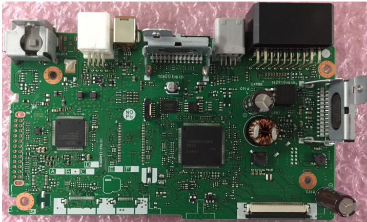
【AUDIO_PCB(Parts side)】
