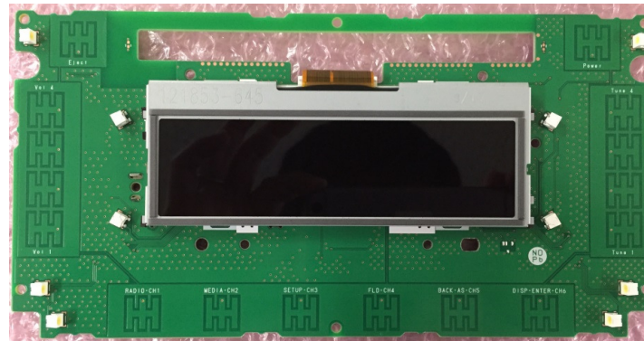
【PANEL_PCB(Parts side)】
