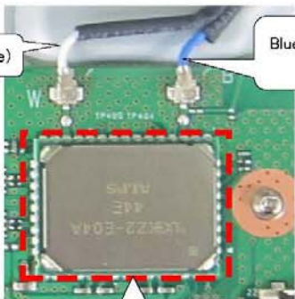
RF Module
