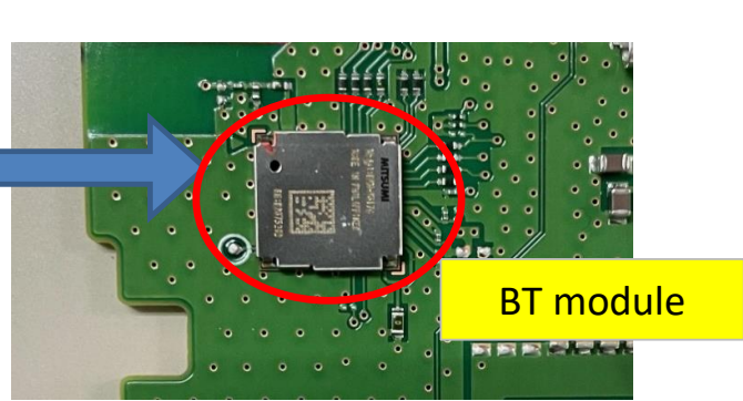
Enlargement
