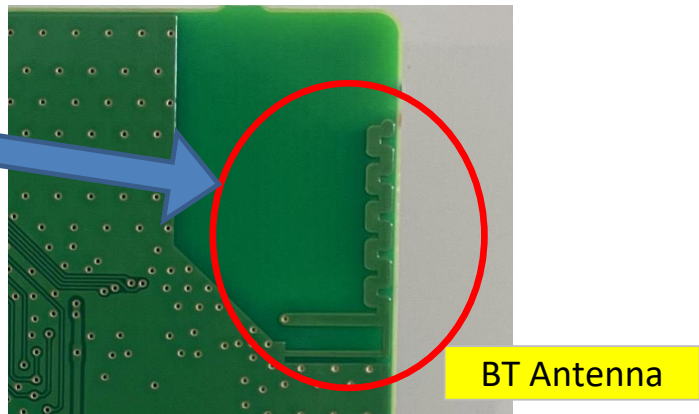
Enlargement
