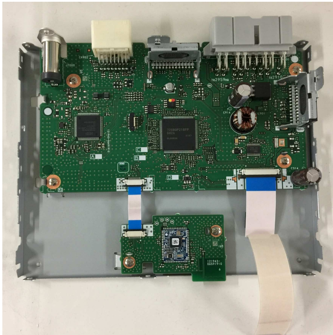
TN0041A 内部写真/internal photo
